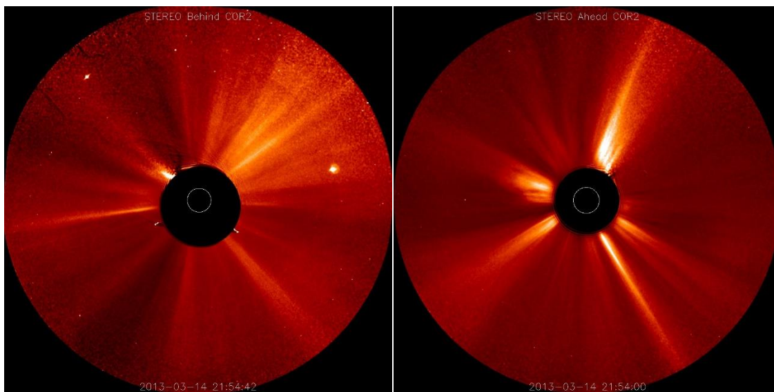
Figura 5.1.8: Imagem da CME obtida pelo STEREO A (direita) e STEREO B (esquerda).
