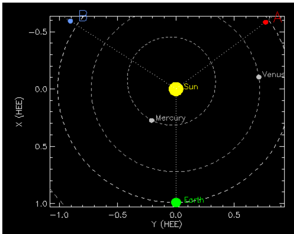
Figura 5.1.6: Imagem órbita dos satélites STEREO A (direita) e STEREO B (esquerda).
