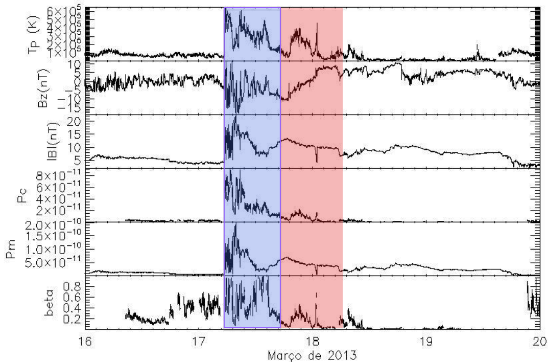
Figura 5.1.2: Parâmetros de plasma do satélite ACE de 16 a 20 de março de 2013.
