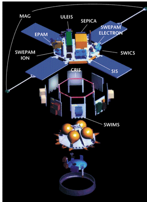
Figura 4.2.1.2: Ilustração da disposição dos instrumentos a bordo do ACE.
