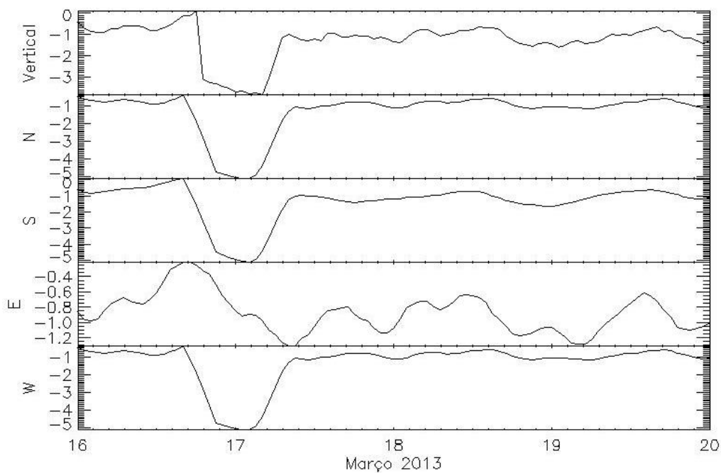
Figura 5.1.3: Variação percentual de muons do DMM do OES.
