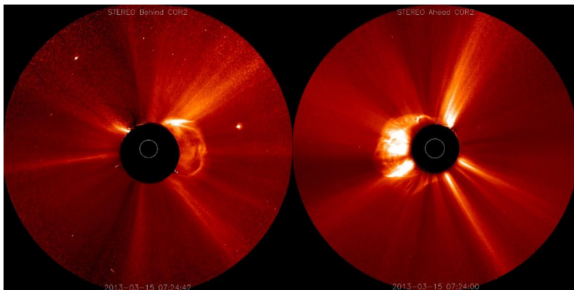
Figura 5.1.10: Imagem da CME do dia 15 de março, obtida pelo STEREO A (direita) e STEREO B (esquerda).
