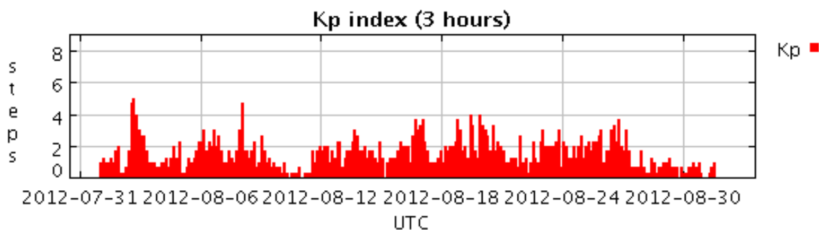
Figura 3.2.1: Índice Kp para o final de julho de 2012 até o final de Agosto de 2012 Fonte: http://spidr.ngdc.noaa.gov/spidr/home.do
