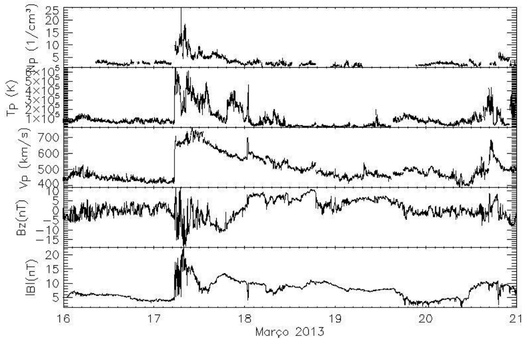
Figura 5.1.1: Parâmetros de plasma do satélite ACE de 16 a 21 de março de 2013.
