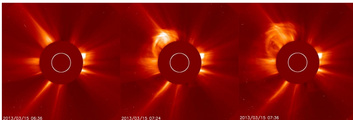
Figura 5.1.9: Sequência de imagens do coronógrafo C2.
