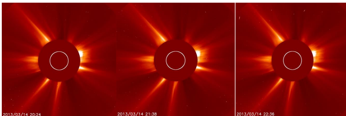
Figura 5.1.7: Sequência de imagens do coronógrafo C2, obtida pelo satélite SOHO.
