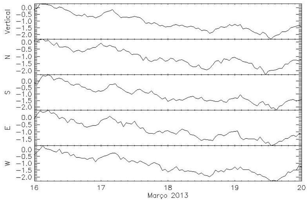
Figura 5.1.4: Variação percentual de muons do DMM instalado em Nagoya.
