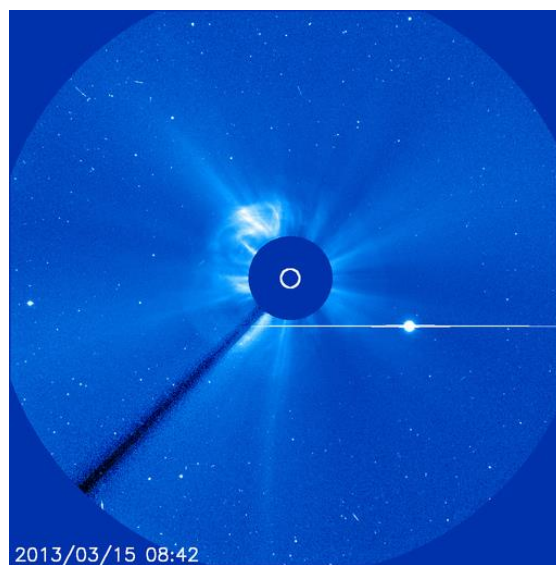
Figura 5.1.11: Imagem da CME do dia 15 de março, obtida pelo coronógrafo C3.
