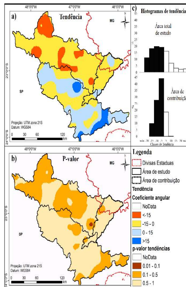
Fig. 5 - (a) Coeficiente angular da regressão linear, relativo à tendência de precipitação acumulada (DJF) de 2003 a 2014; (b) p-valor referente à significância das tendências; (c) histogramas das classes de tendência na área de estudo e na área de contribuição dos reservatórios.
