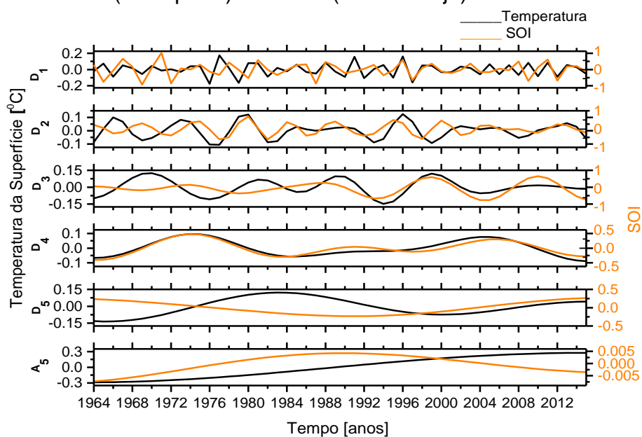
Figura C.105 - Decomposição da anomalia da temperatura da superfície de 24 0 S a 90 0 S (linha preta) e do SOI (linha laranja).
