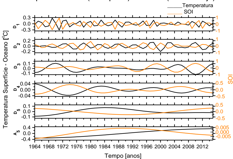
Figura C.106 - Decomposição da anomalia da temperatura superfície - oceano do Equador a 24 0 S (linha preta) e do SOI (linha laranja).
