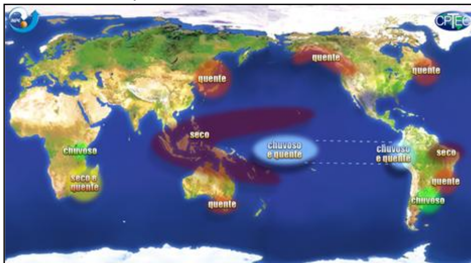
Figura 2.18 - Efeitos globais da ocorrência do El Niño durante os meses de dezembro, janeiro e fevereiro.
