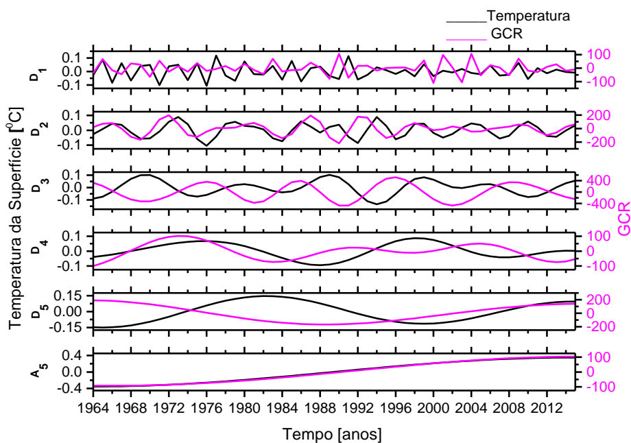
Figura C.72 - Decomposição da anomalia da temperatura da superfície de 24 0 S a 44 0 S (linha preta) e do GCR (linha magenta).
