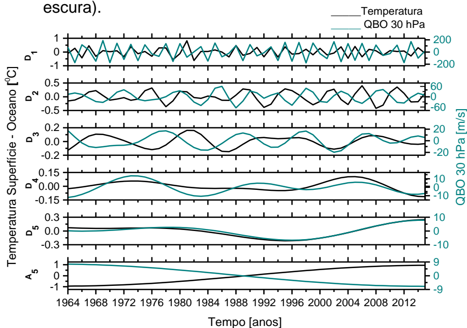
Figura C.59 - Decomposição da anomalia da temperatura superfície - oceano de 64 o N a 90 o N (linha preta) e da QBO 30 hPa (linha verde - escura).
