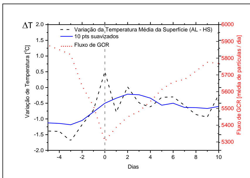
Figura 5.11 - Análise de série de época superposta da variação da temperatura média diária da superfície \Delta T (linha preta tracejada) da região de altas latitudes ( 60^{\circ} - 70^{\circ} ) do Hemisfério Sul e do fluxo de GCR.
