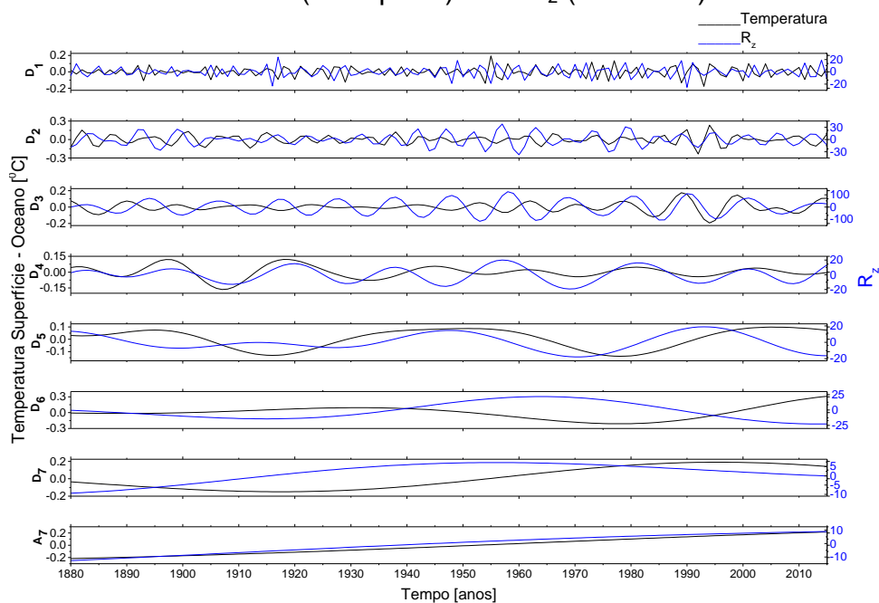
Figura C.17 - Decomposição da anomalia da temperatura superfície - oceano de 24 o N a 44 o N (linha preta) e do R z (linha azul).
