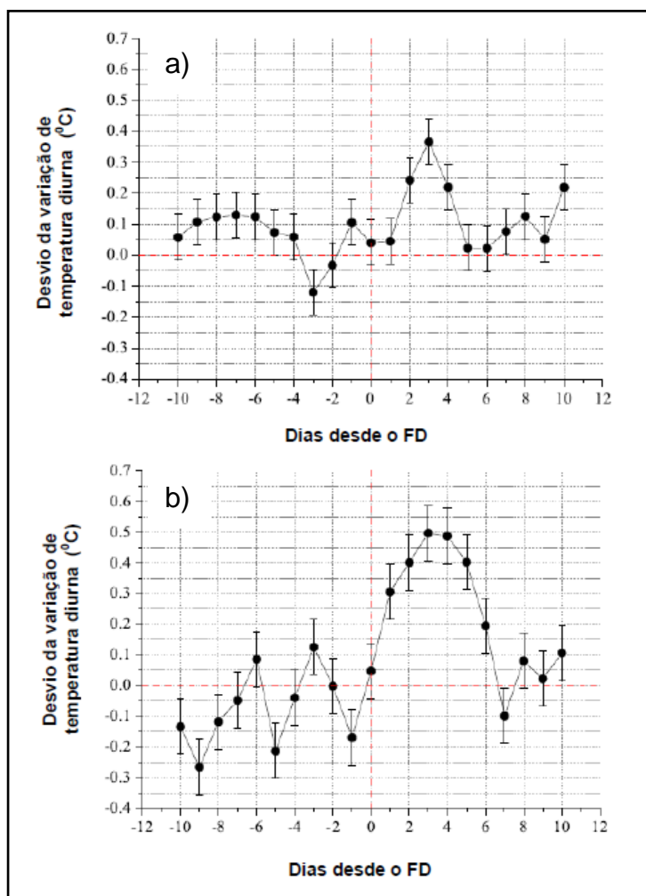
Figura 3.24 - Variação da temperatura diurna de épocas superpostas antes, durante e após a) 22 eventos com amplitudes entre 7% e 10% e b) 13 com amplitudes acima de 10%.
