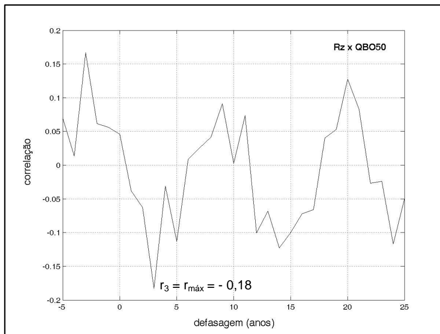
Figura 5.101 - Correlação cruzada entre os dados de R_z e QBO 50 hPa, de 1964 a 2015.
