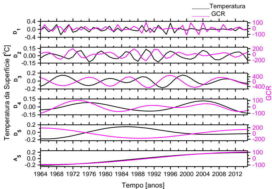
Figura C.73 - Decomposição da anomalia da temperatura da superfície de 44 0 S a 64 0 S (linha preta) e do GCR (linha magenta).
