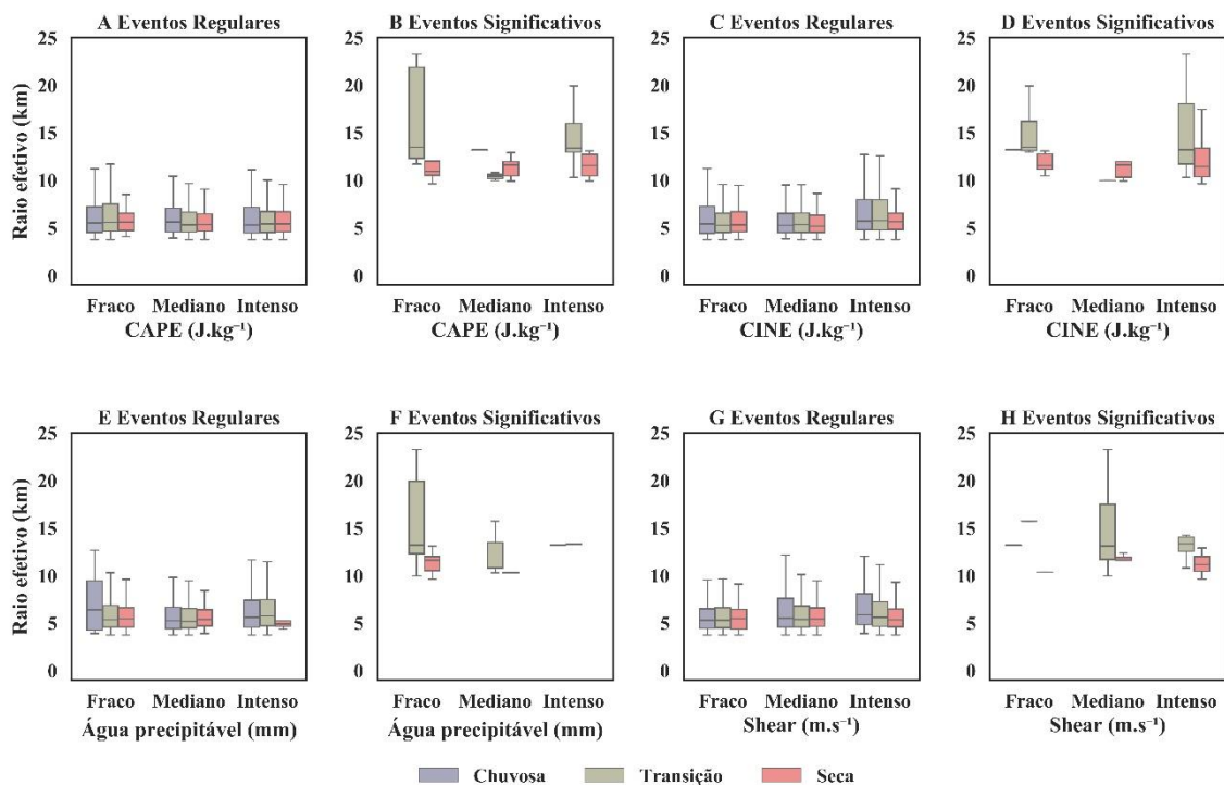
Figura 5.7 - Raio efetivo para eventos regulares e significativos.
