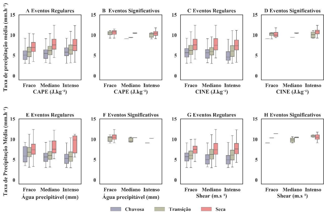
Figura 5.6 - Taxa de precipitação para eventos regulares e significativos.
