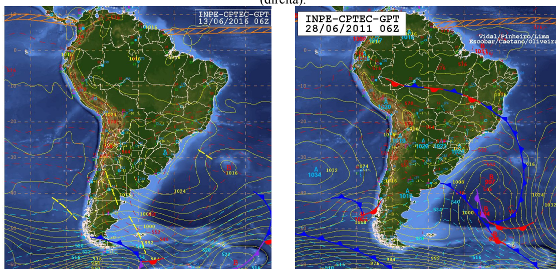
Figura 9 - Análise sinótica das 06Z (03:00 de Brasília) do dia 13/06/2016 (esquerda) e 28/06/2011 (direita).
