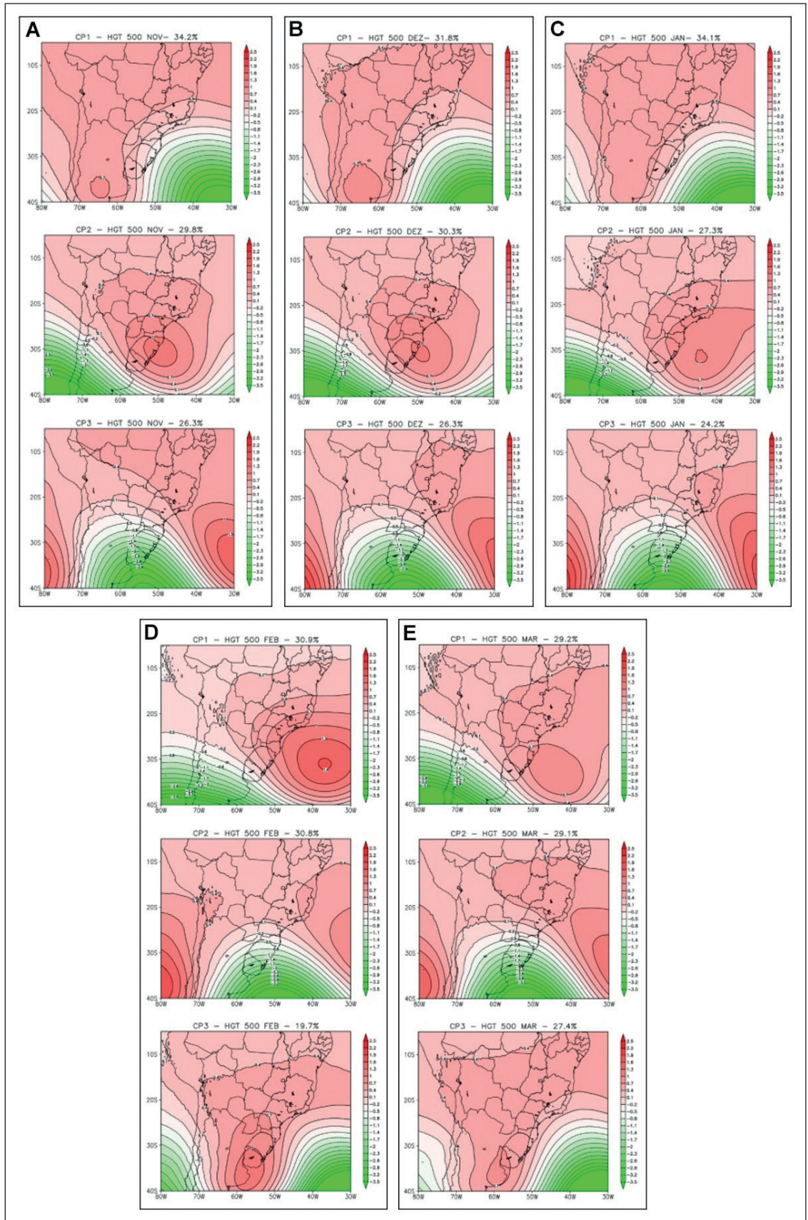
Figura 2 CPs em 500 hPa durante a ECB; A. Novembro; B. Dezembro; C. Janeiro; D. Fevereiro; E. Março.
