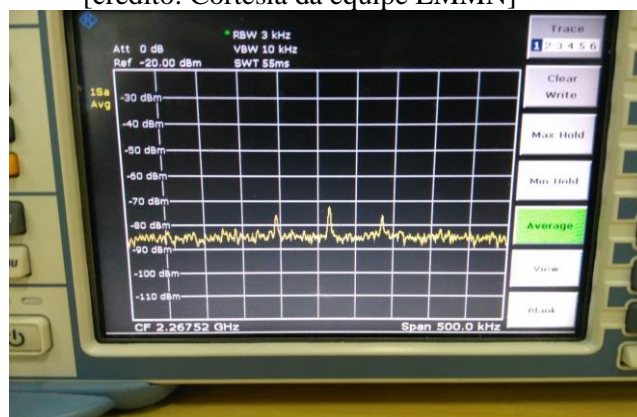
Figura 12. Analisador de Espectro sintonizado para recebimento do sinal do DCS em Banda-S [crédito: Cortesia da equipe EMMN]
