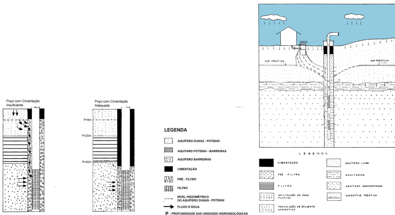
Figura 1 – (a) Representação esquemática de poços no aquífero livre Dunas-Potengi e semi-confinado Barreiras. (b) Corte esquemático mostrando o mecanismo de poluição dos poços com proteção sanitária incompleta. Modificado de ACQUA-PLAN (1988) [5].
