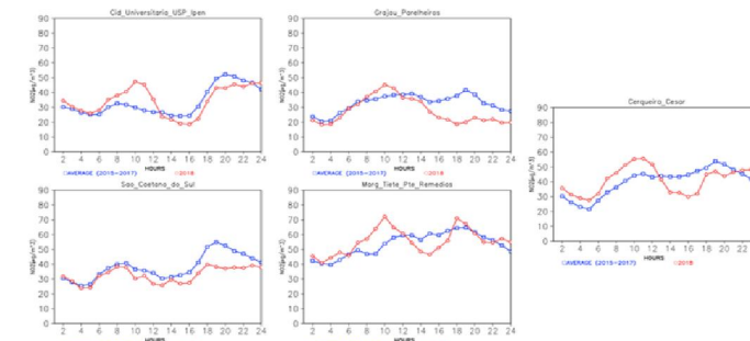
Fig. 3. Concentração de NO 2 (µg m -3 ) na RMSP média horária do período sem greve (2015-2017) e com greve (2018)
