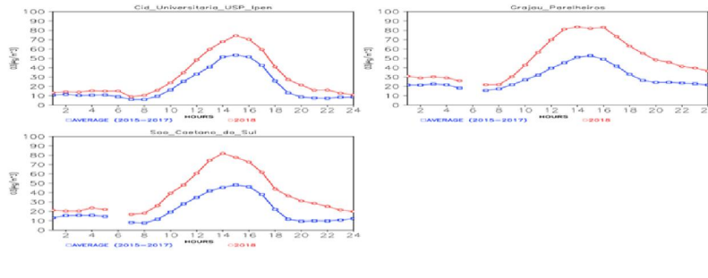
Fig. 4. Concentração de O 3 (µg m -3 ) na RMSP média horária do período sem greve (2015-2017) e com greve (2018)
