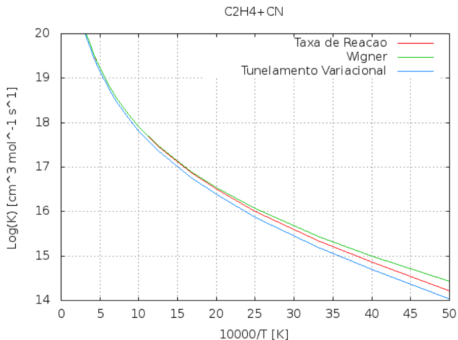
Figura 4 – comparação das taxas com a temperatura recíproca ( \text{K}^{-1} ) para a reação \text{C}_2\text{H}_4 + \text{CN} = \text{C}_2\text{H}_3 + \text{HCN}
