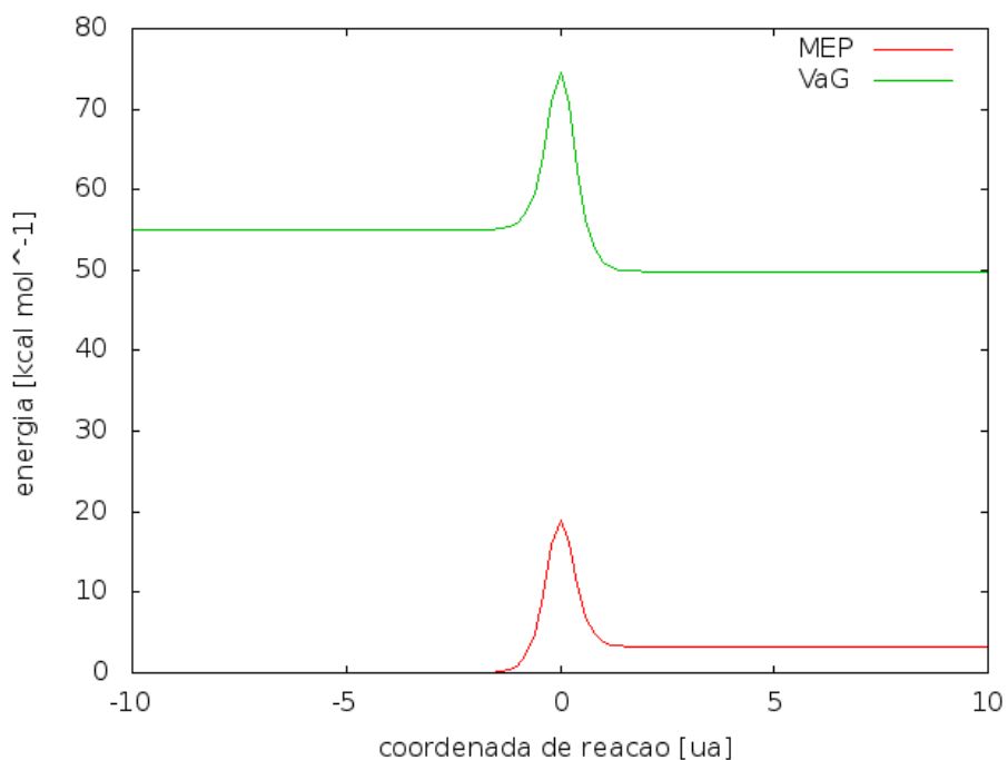
Figura 7 – comparação da MEP com V_a^G para a reação NH_3+H=NH_2+H_2
