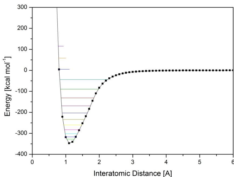
Figura 13 – Curva de energia potencial para a reação CO + CO = CO_2 + C , com os níveis rovibracionais inclusos
