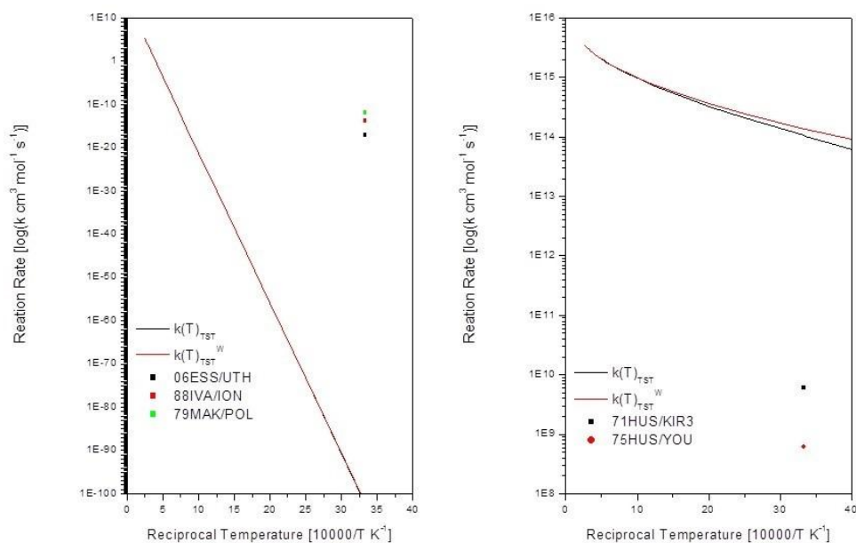
Figura 11 – comparação das taxas com a temperatura recíproca ( K^{-1} ) para a reação CO + CO = CO_2 + C , sem a inclusão dos níveis rovibracionais
