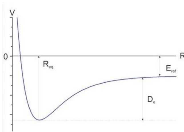
Figura 3: Curva de energia potencial.
