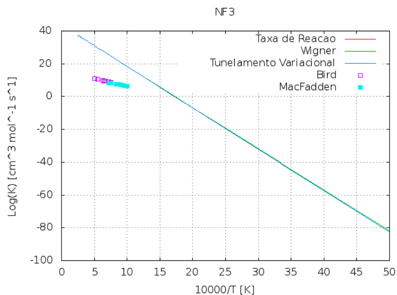
Figura 8 – comparação das taxas com a temperatura recíproca ( \text{K}^{-1} ) para a reação unimolecular \text{NF}_3 = \text{NF}_2 + \text{F} , com os dados de referência Bird [13] e MacFadden [14]
