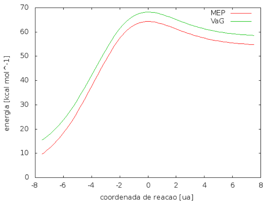
Figura 9 – comparação da MEP com V_a^G para a reação \text{NF}_3 = \text{NF}_2 + \text{F}
