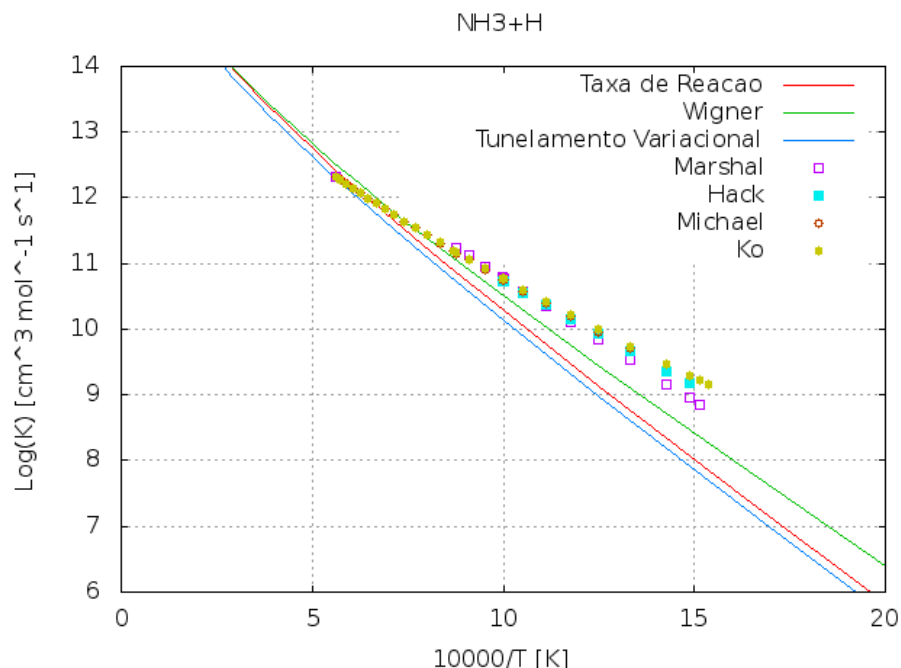
Figura 6 – comparação das taxas com a temperatura recíproca ( K^{-1} ) para a reação NH_3+H=NH_2+H_2 , com os dados de referência Marshall [9], Hack [10], Michael [11] e Ko[12]
