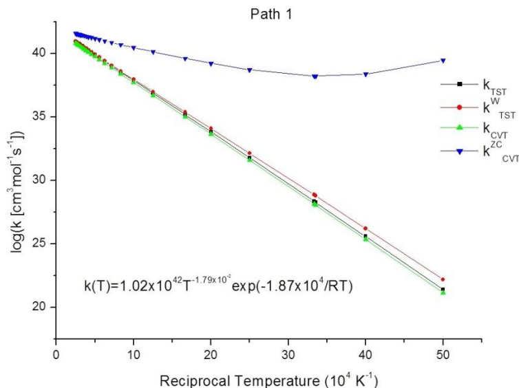
Figura 10 – comparação das taxas com a temperatura recíproca ( \text{K}^{-1} ) para a reação \text{CH}_3\text{CO}_2\text{OH} + \text{H}_2\text{O} = \text{CH}_3\text{O}_2\text{H} + \text{CH}_4
