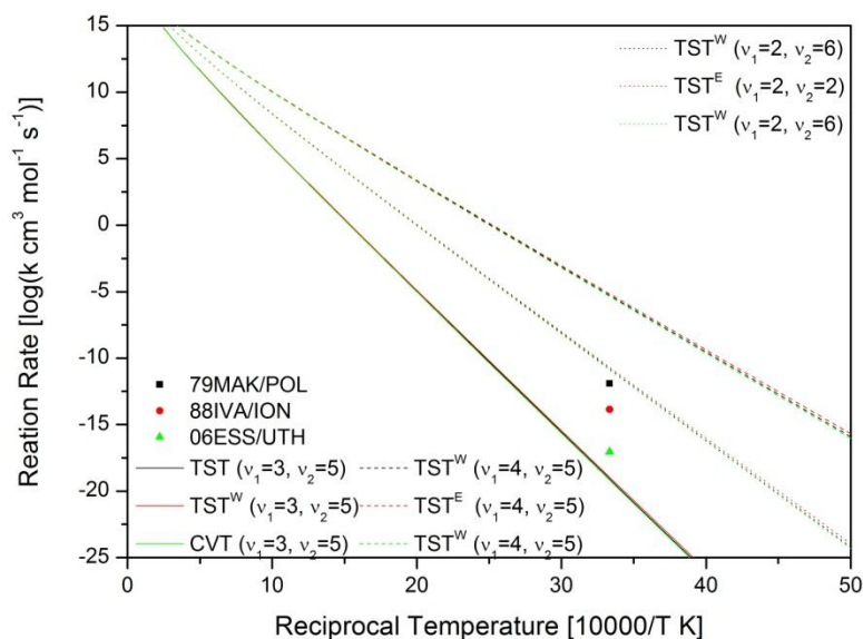
Figura 12 – comparação das taxas com a temperatura recíproca ( K^{-1} ) para a reação CO + CO = CO_2 + C , com os níveis rovibracionais inclusos
