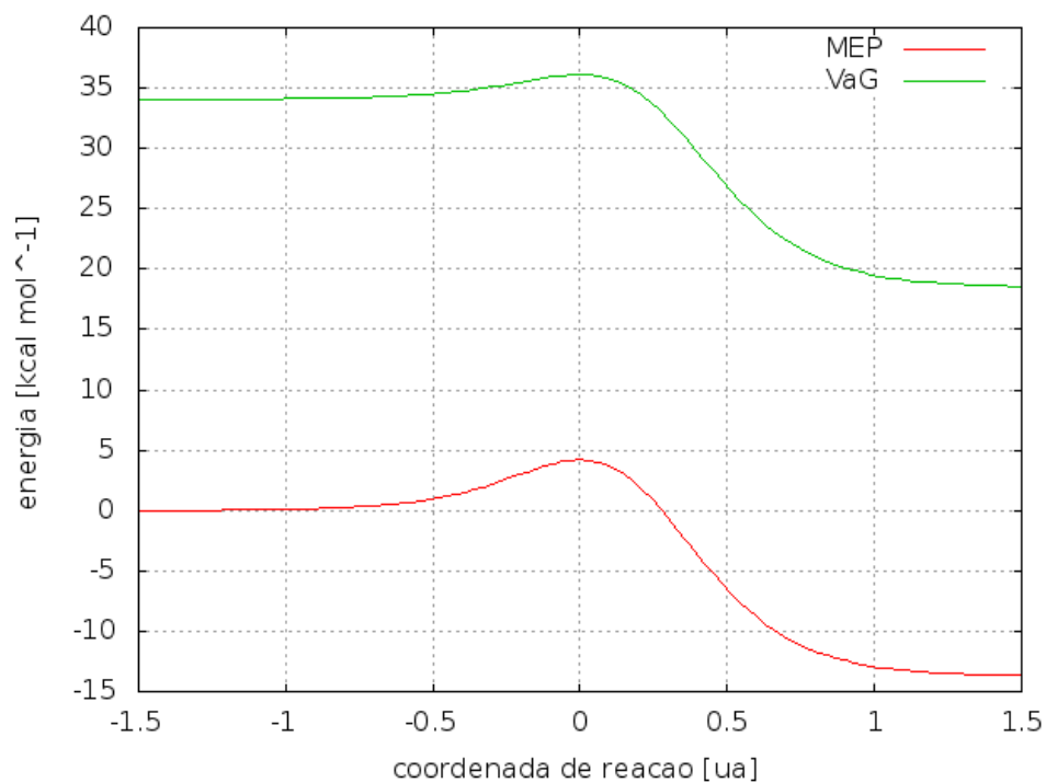
Figura 5 – comparação da MEP com V_a^G para a reação C_2H_4 + CN = C_2H_3 + HCN
