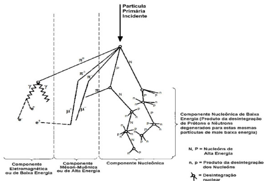
Figura 18: Diagrama esquemático de um chuvaire de raios cósmicos. Fonte: Modificado de Forbush (1993).
