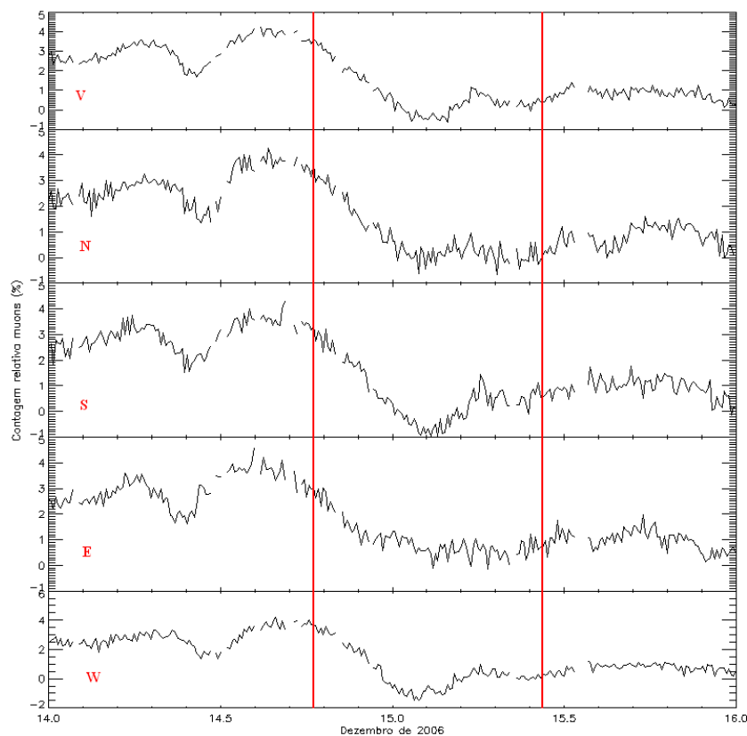
Figura 35: Contagem relativa de muons nas direções vertical (V), norte 30° (N), sul 30° (S), leste 30° (E) e oeste 30° (W), mostrando o decréscimo de Forbush relacionado a uma tempestade geomagnética.
