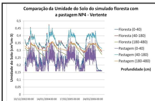
Figura 46. Comparação da umidade do solo – NP4 na Vertente Floresta-Pastagem.
