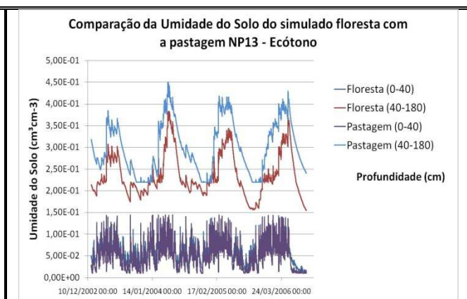
Figura 51. Comparação da umidade do solo – NP13 no Ecótono Floresta-Pastagem.
