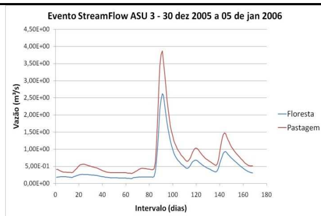
Figura 40. Evento-vazão no período de 30 dezembro a 05 de janeiro de 2006 dos dados da Asu 3 Floresta-Pastagem.
