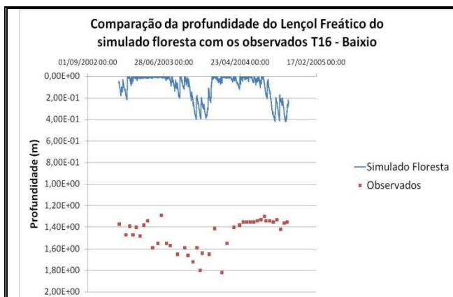
Figura 24. Comparação da profundidade do lençol freático – T16 no Baixio Floresta-Observado.
