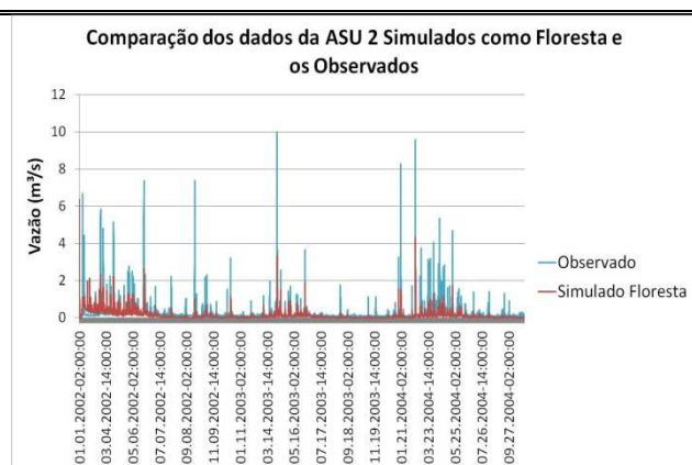
Figura 8. Comparação da vazão dos dados da Asu 2 Floresta-Observado.
