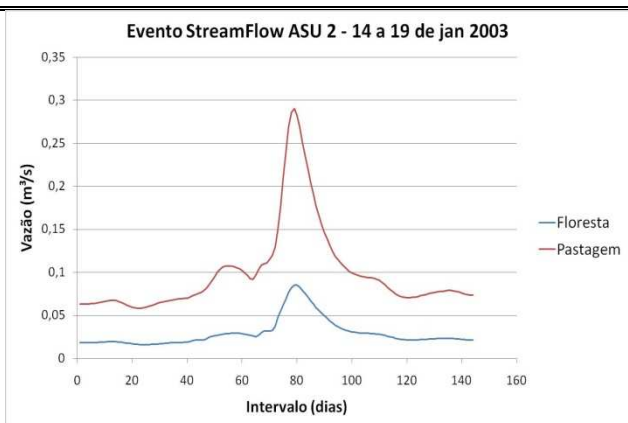
Figura 37. Evento-vazão no período de 14 a 19 de janeiro de 2003 dos dados da Asu 2 Floresta-Pastagem.
