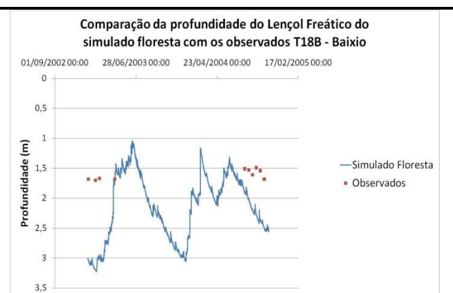
Figura 27. Comparação da profundidade do lençol freático – T18B no Baixio Floresta-Observado.
