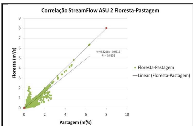
Figura 33. Correlação da vazão dos dados da Asu 2 Floresta-Pastagem.
