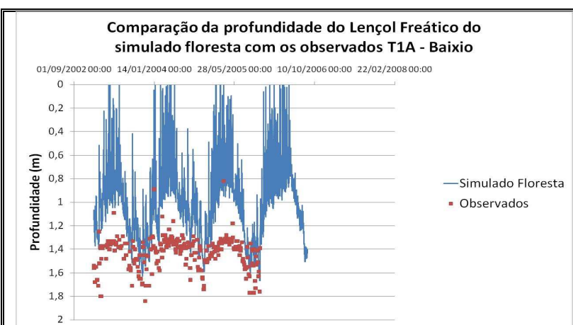
Figura 31. Comparação da profundidade do lençol freático – T1A no Baixo Floresta-Observado.
