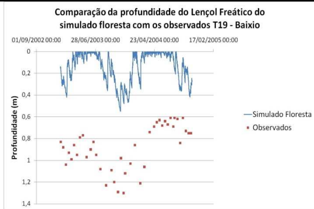
Figura 28. Comparação da profundidade do lençol freático – T19 no Baixo Floresta-Observado.
