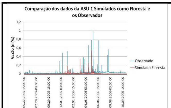
Figura 7. Comparação da vazão dos dados da Asu 1 Floresta-Observado.
