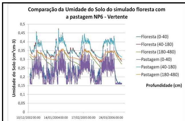
Figura 48. Comparação da umidade do solo – NP6 na Vertente Floresta-Pastagem.
