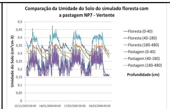
Figura 49. Comparação da umidade do solo – NP7 na Vertente Floresta-Pastagem.
