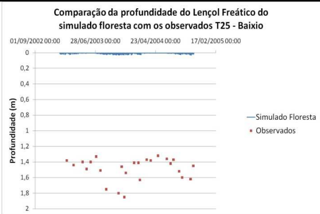
Figura 29. Comparação da profundidade do lençol freático – T25 no Baixo Floresta-Observado.
