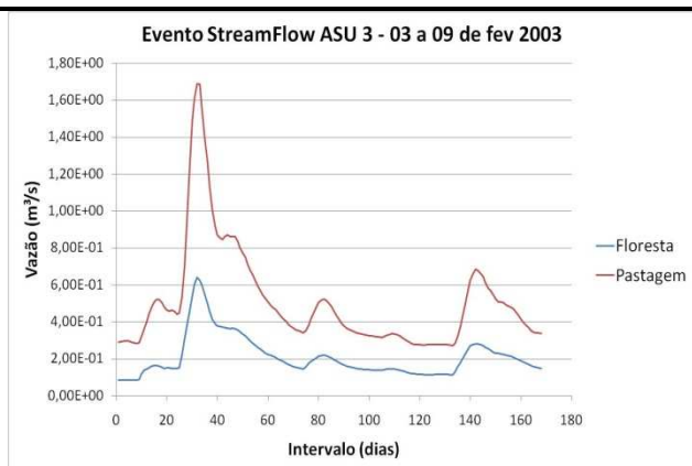
Figura 39. Evento-vazão no período de 03 a 09 de fevereiro de 2003 dos dados da Asu 3 Floresta-Pastagem.
