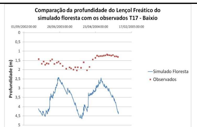
Figura 25. Comparação da profundidade do lençol freático – T17 no Baixio Floresta-Observado.
