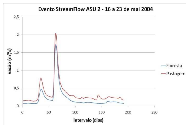
Figura 38. Evento-vazão no período de 16 a 23 de maio de 2004 dos dados da Asu 2 Floresta-Pastagem.
