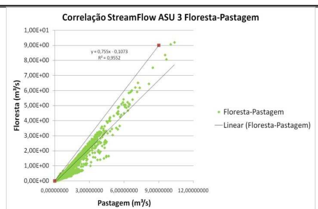
Figura 34. Correlação da vazão dos dados da Asu 3 Floresta-Pastagem.
