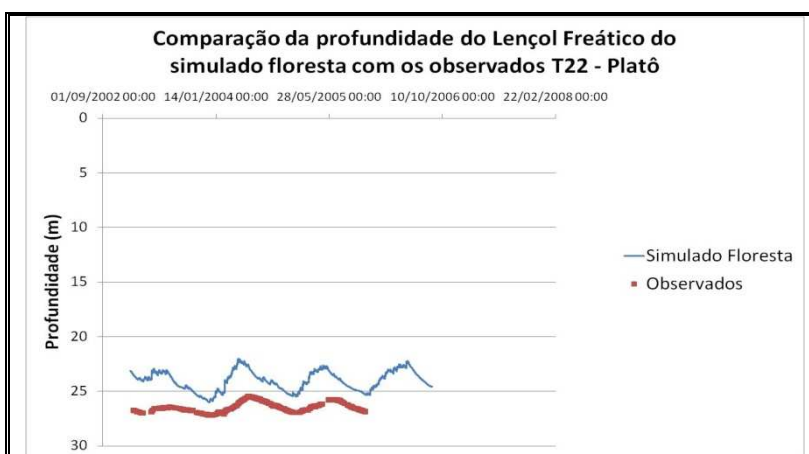
Figura 30. Comparação da profundidade do lençol freático – T22 no Platô Floresta-Observado.
