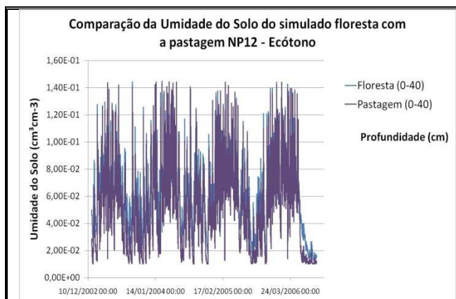
Figura 50. Comparação da umidade do solo – NP12 no Ecótono Floresta-Pastagem.
