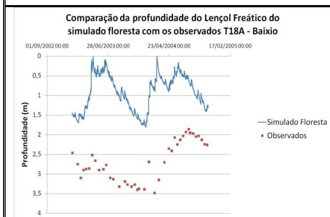
Figura 26. Comparação da profundidade do lençol freático – T18A no Baixio Floresta-Observado.
