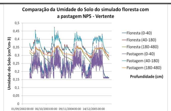
Figura 47. Comparação da umidade do solo – NP5 na Vertente Floresta-Pastagem.
