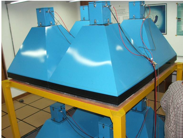
Figura 3.2 – Foto de protótipo telescópio detector de muons instalado no OES/CRS/CIE/INPE – MCT mostrando em azul os 8 detectores em duas camadas.
