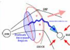
Figura 4: Representação esquemática do cone de partículas na direção Sol - CME - Terra.
