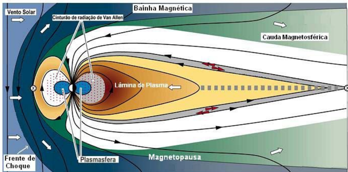
Figura 1.14 – Devido à interação com o vento solar, a magnetosfera toma a forma da figura acima. Fonte: Tese de mestrado – Aline de Lucas - ESTUDO DA DINÂMICA DA CORRENTE DE ANEL DURANTE A FASE PRINCIPAL DE SUPERTEMPESTADES MAGNÉTICAS.
