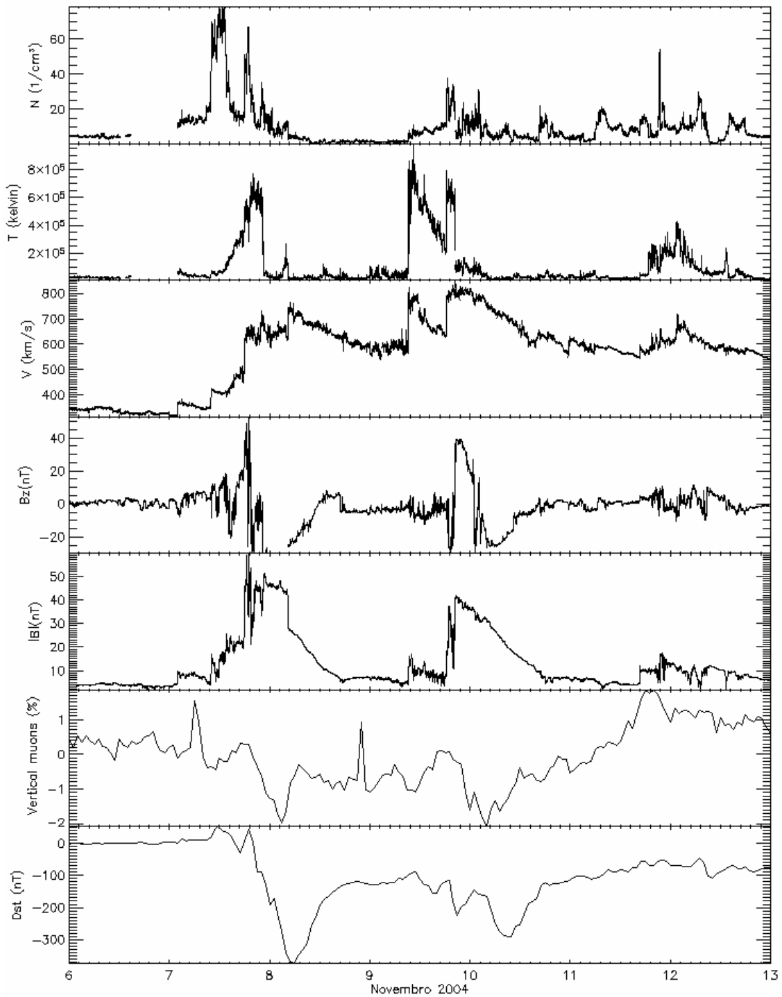
Figura 4.8– Índice Dst, muons telescópio protótipo e dados do Satélite ACE correlacionados.
