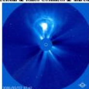
Figura 1: Ejeção de massa coronal em 27 de fevereiro de 2000 fotografada por LASCO C2 and C3. (Fonte: NASA Satellite SOHO)
