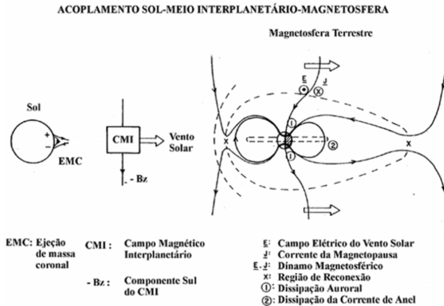
Figura 1.15 – Acoplamento entre Sol, Meio Interplanetário e magnetosfera Terrestre. Fonte: Adaptada de Gonzalez et al. (1994).
