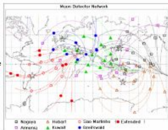
Figura 3: Rede mundial de detectores de raios cósmicos de alta energia – muons (utilizada).
