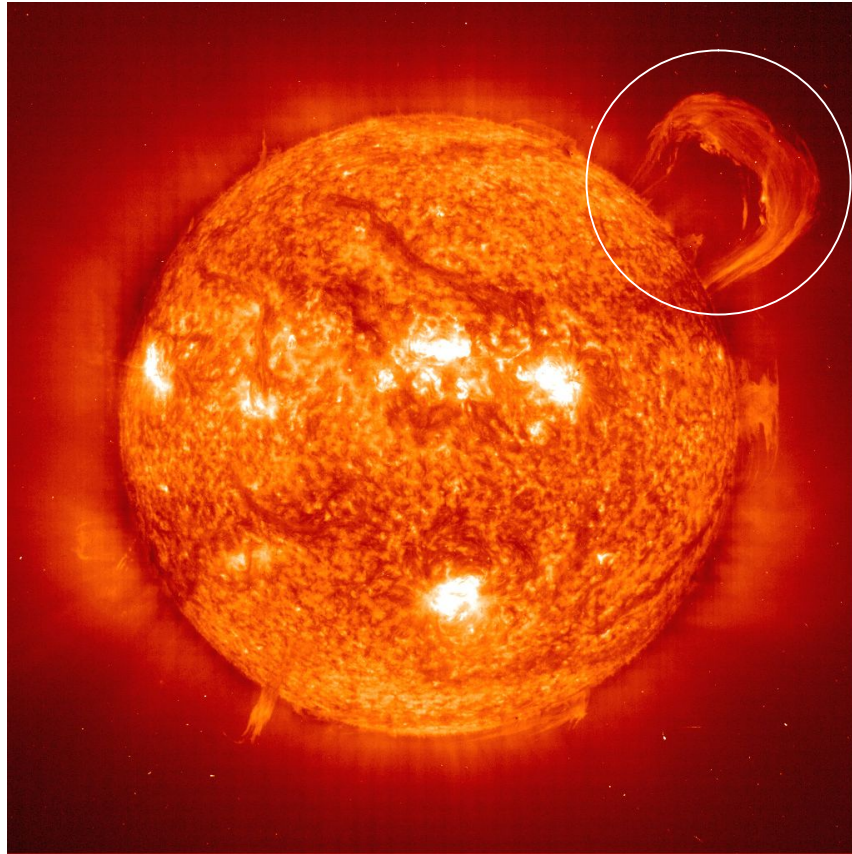
Figura 1.6 – Proeminência solar visível na região do extremo ultravioleta EIT (SOHO/EIT - -Extreme ultraviolet Imaging Telescope).
