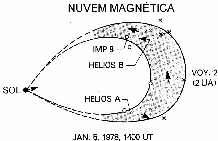
Figura 1.12 – Geometria de uma nuvem magnética.
