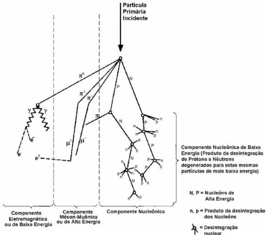
Figura 2.1 – Figura esquemática dos raios cósmicos que colidem com partículas da atmosfera Terrestre (chuveiro de raios cósmicos). FONTE: Modificado de Forbush (1993).
