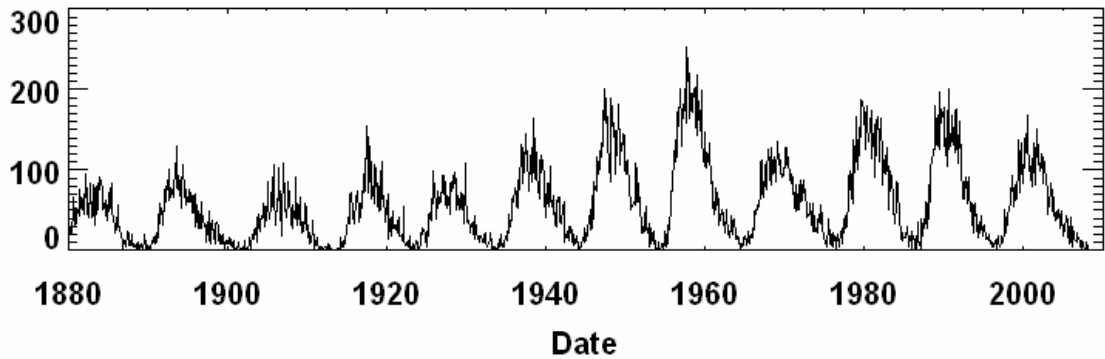
Figura 1.4 – Gráfico do número de manchas solares em função do tempo, ciclo de atividade solar de 1880 a 2000 aproximadamente.
