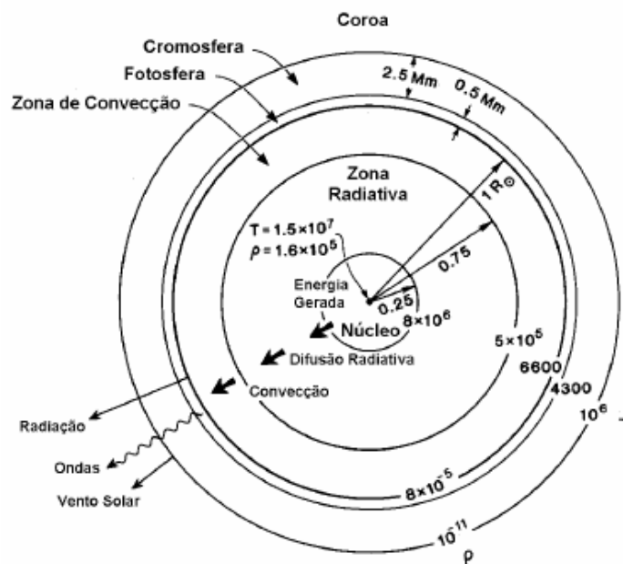
Figura 1.2 – Clássica estrutura solar de seu interior. Fonte: Kivelson e Russell, 1995.
