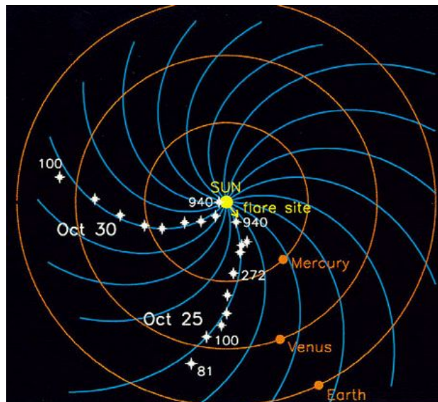
Figura 1.9 – Ilustração do Campo Magnético Interplanetário. (Fonte: http://www.windows.ucar.edu/tour/link=/sun/imf.sp.html&edu=high )
