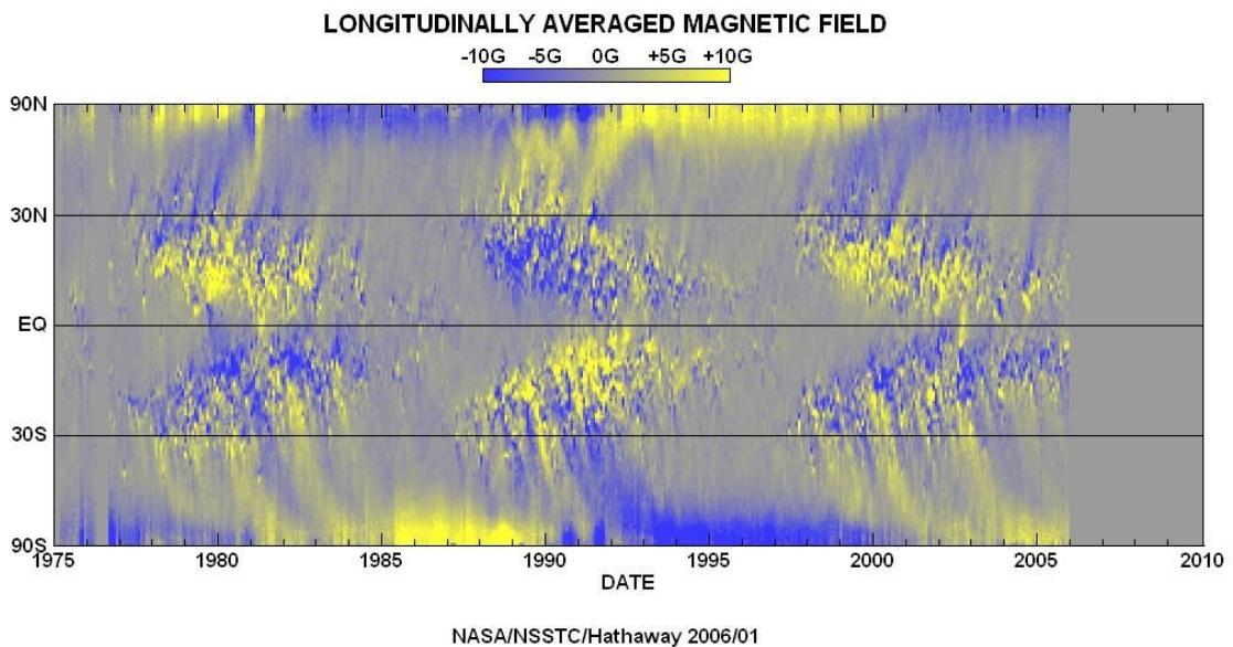
Figura 1.5 – Diagrama da borboleta do período de 1977- 2006 aproximadamente.
