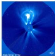
Figura 1: Ejeção de massa coronal em 27 de março de 2006 observada por LASCO C2 and C3. (Fonte: NASA Satellite SOHO)
