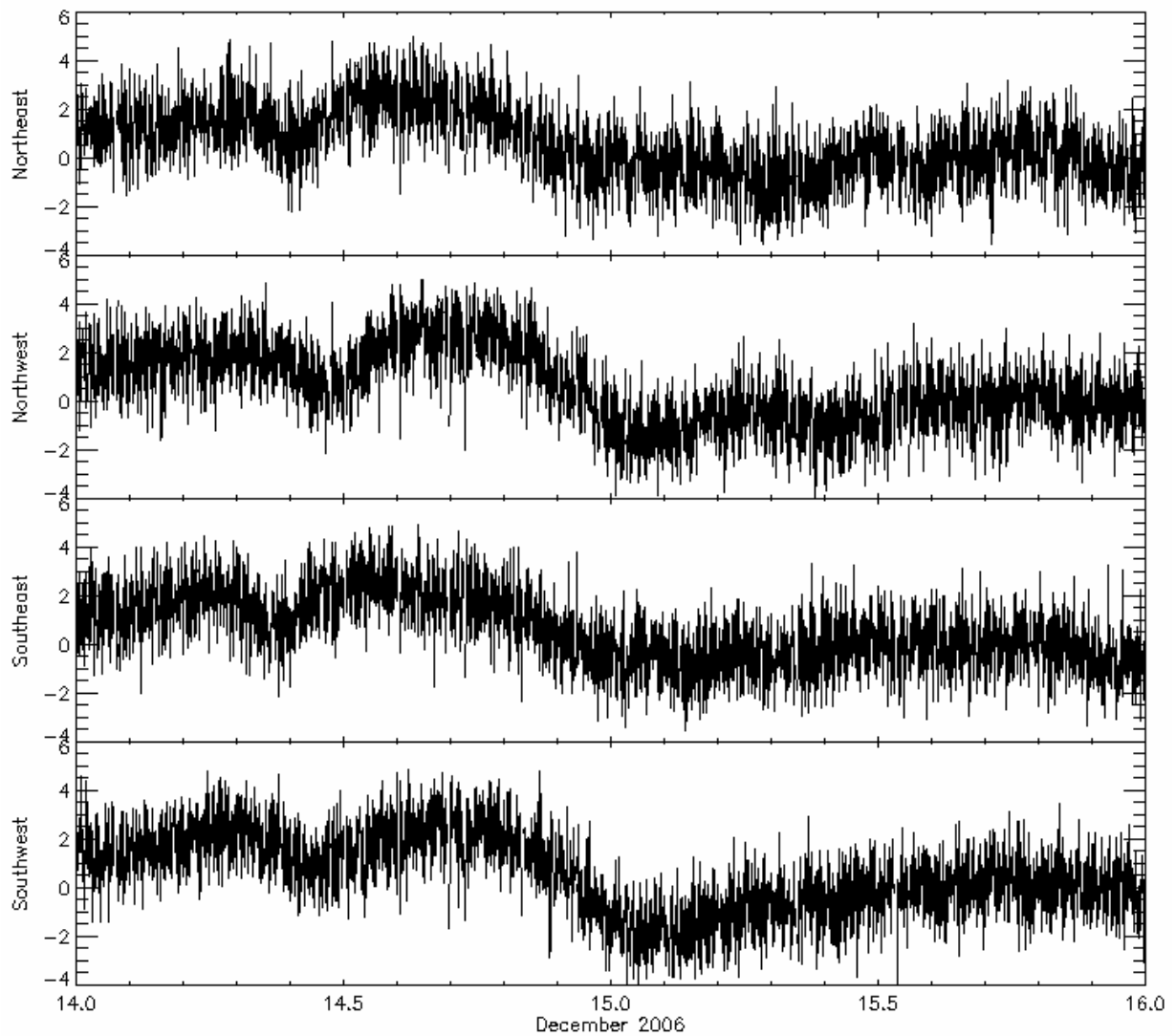
Figura 4.6 – Mesmas direções comparadas com o protótipo.
