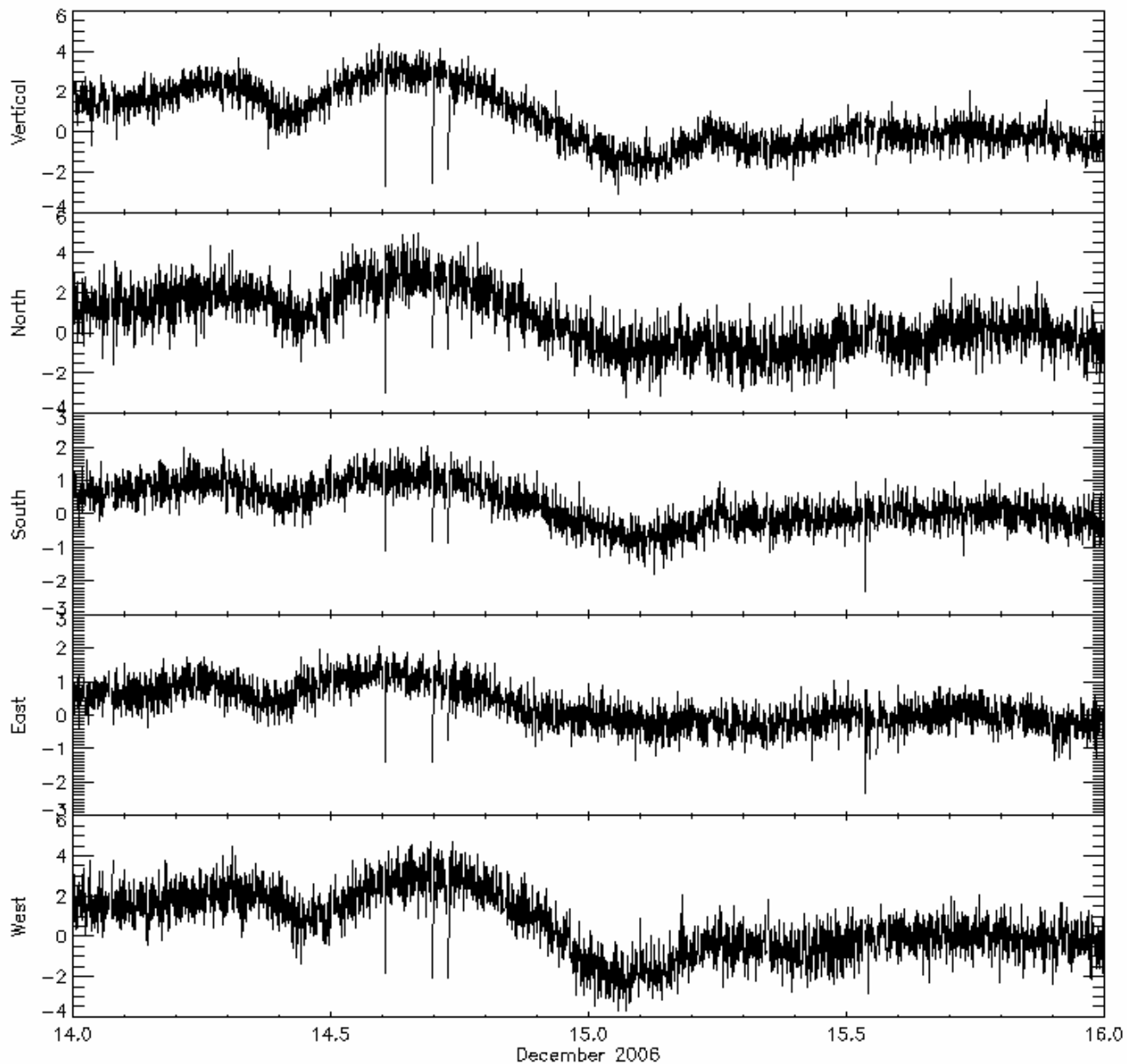
Figura 4.5– Gráficos das componentes N, S, E e W comparadas com a vertical.
