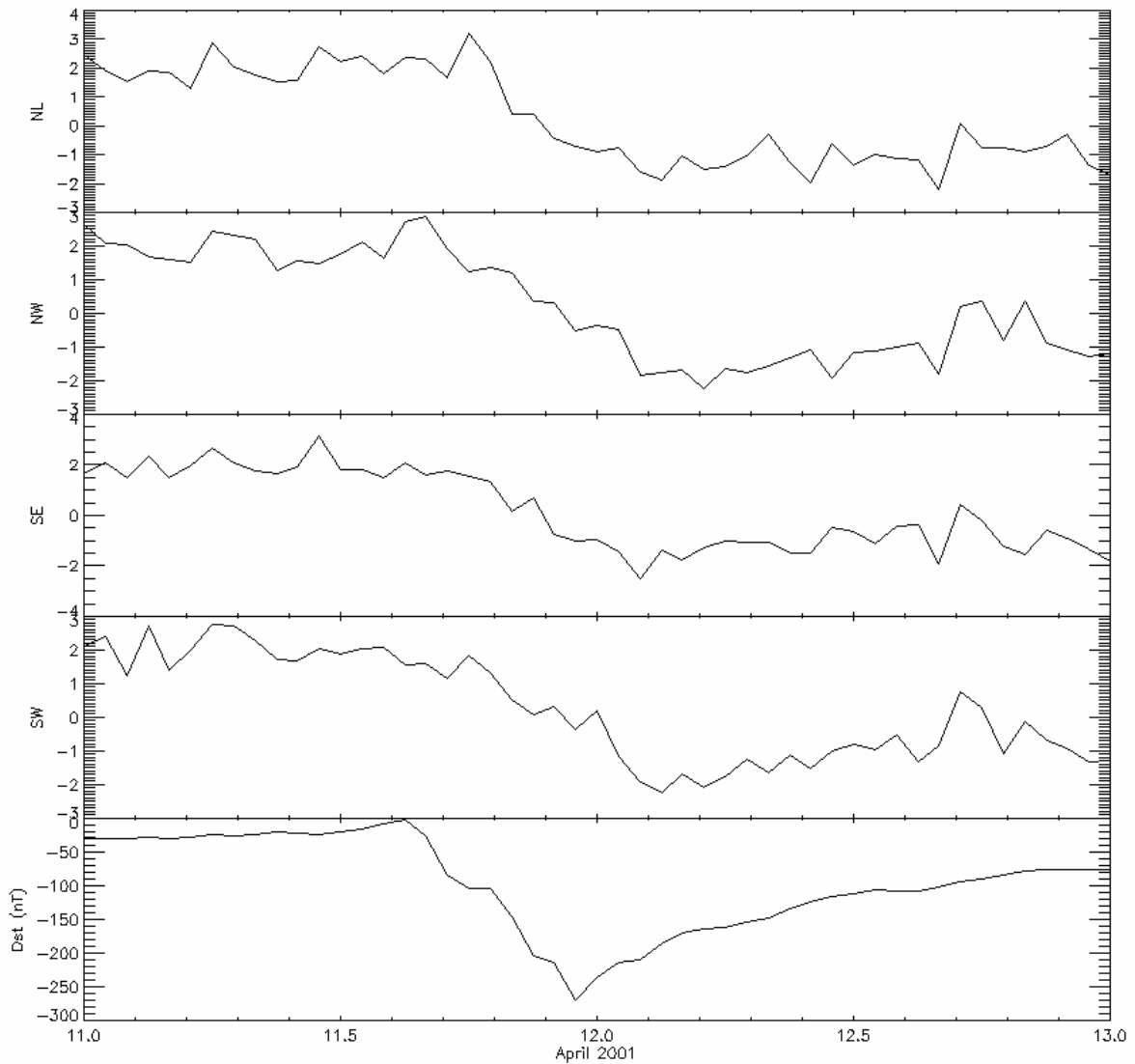
Figura 4.3 – Outras direções comparadas com o índice Dst.
