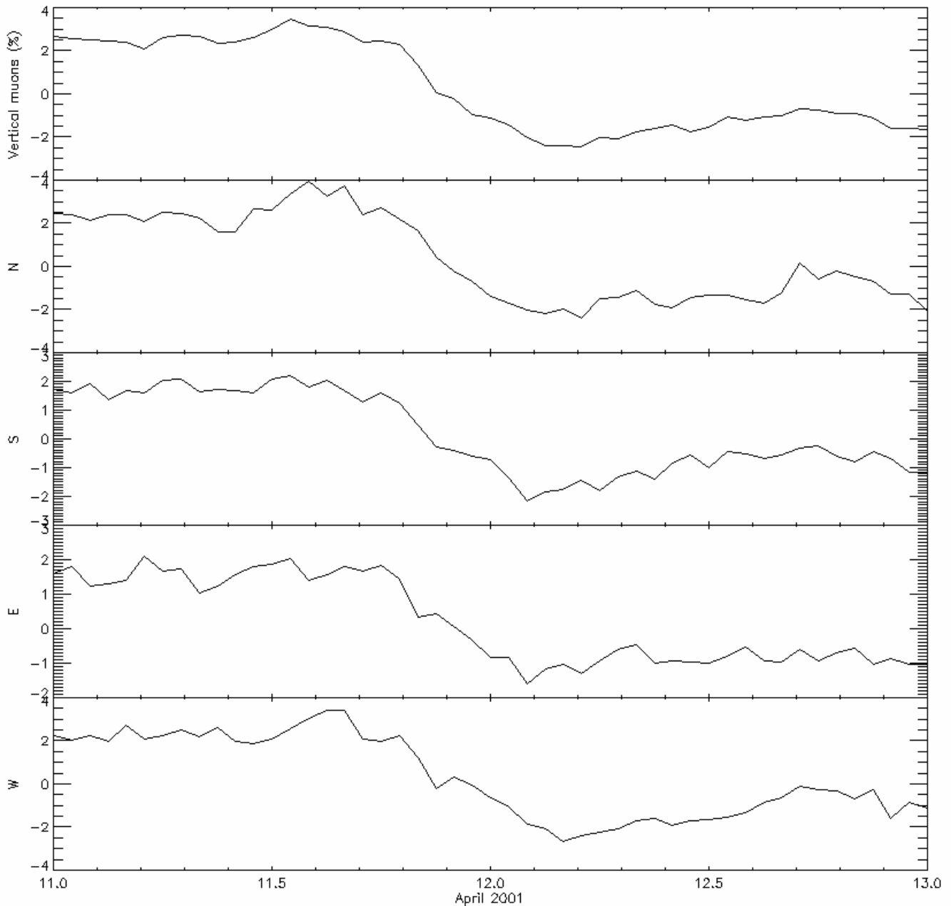
Figura 4.2 – Gráficos das componentes N, S, E e W.
