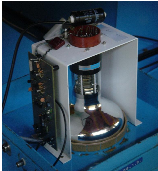
Figura 3.7 – Foto da fotomultiplicadora utilizada no detector de raios cósmicos – muons.
