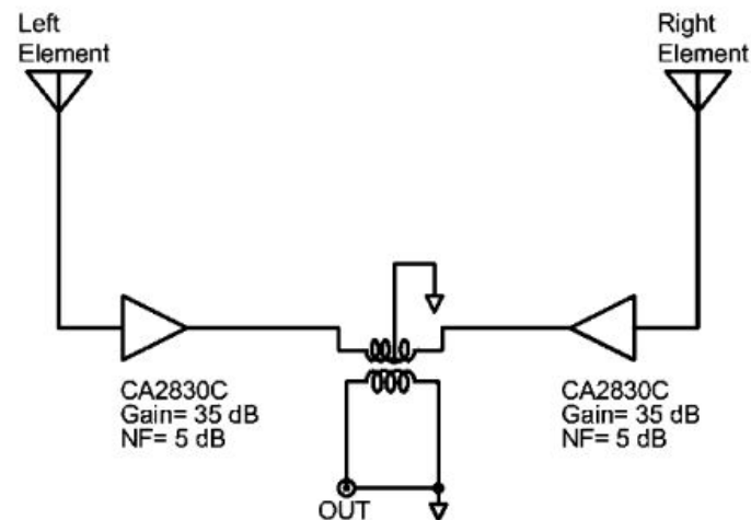
FIG. 5.25 – BALUN ATIVO.
