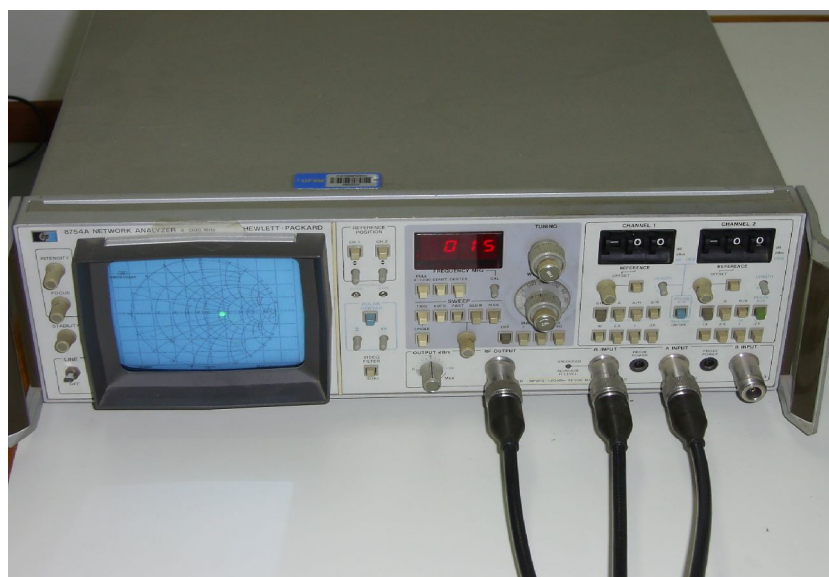
FIG. 5.4 - ANALISADOR DE REDE DA HP, MODELO 8754A, DO LABORATÓRIO DE RADIOFREQUÊNCIA E COMUNICAÇÕES DO CENTRO REGIONAL SUL DE PESQUISAS ESPACIAIS – LRC/CRS/CIE/INPE – MCT, EM SANTA MARIA, RS.
