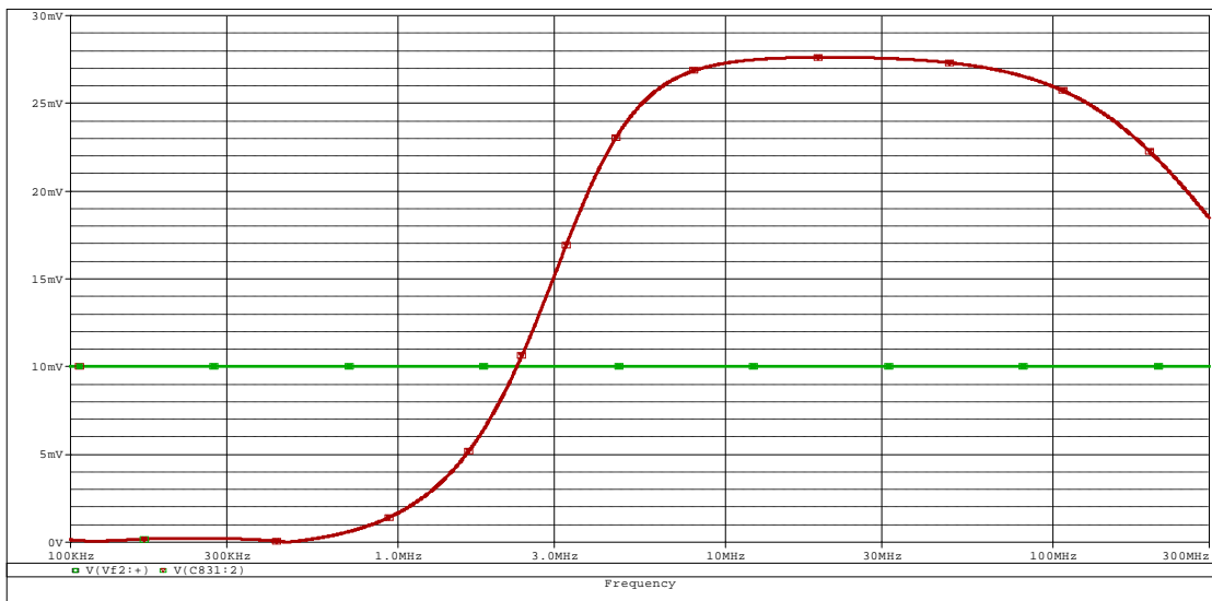
FIG. 5.28 – TENSÕES DE ENTRADA/SAÍDA DO CIRCUITO DA FIG. 5.27 PARA CASAMENTO DE IMPEDÂNCIA PARA ANTENA PROTÓTIPO SIMILAR À DO SISTEMA LOFAR.
