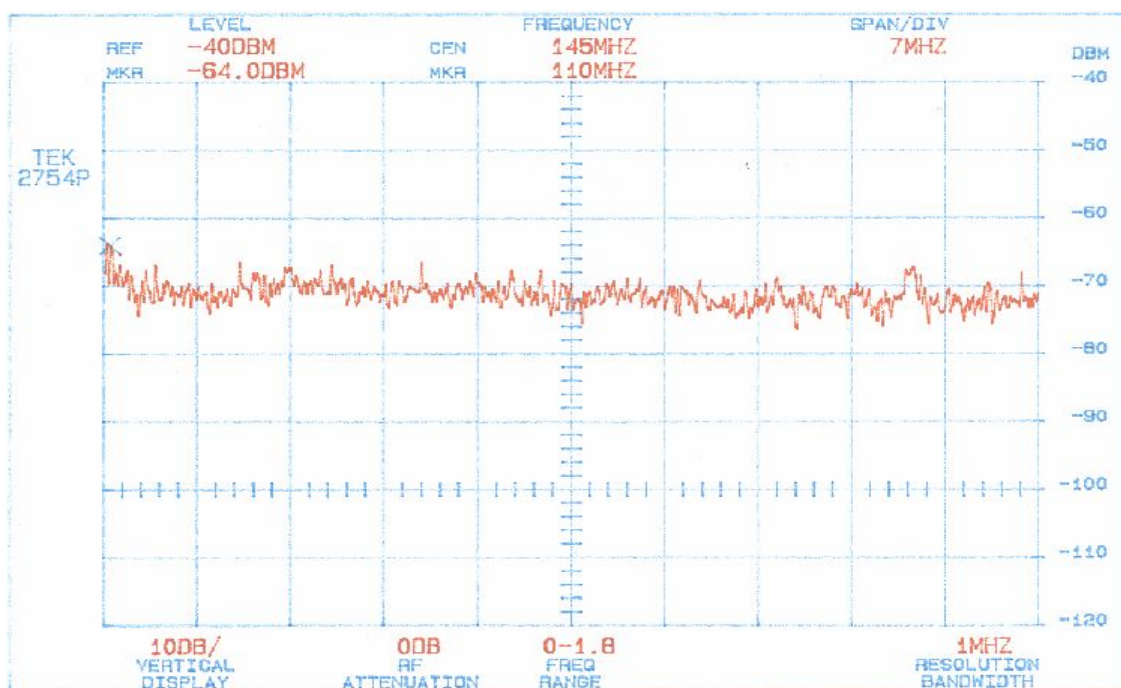
FIG. 5.8 - GRÁFICO DOS SINAIS NA LARGURA DE BANDA DE 110 – 180 MHZ, NO OBSERVATÓRIO ESPACIAL DO SUL EM SÃO MARTINHO DA SERRA, RS, EM 2003.
