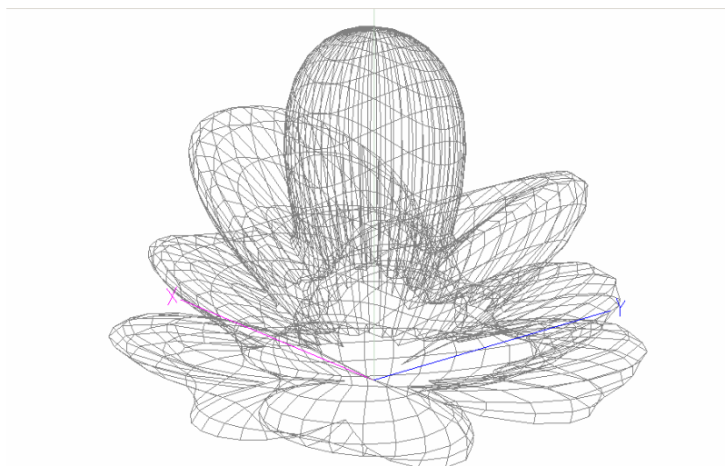
FIG. 5.36 – DIAGRAMA DE IRRADIAÇÃO TRIDIMENSIONAL DA ANTENA DIPOLO SIMILAR À DO SISTEMA LOFAR PARA A FREQUÊNCIA DE 90 MHZ.
