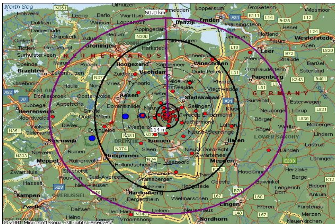
FIG. 1.3.6.1 – EM VERMELHO, NO MAPA, A DISPOSIÇÃO DAS PRIMEIRAS 32 ESTAÇÕES DA FASE 1 DO LOFAR
