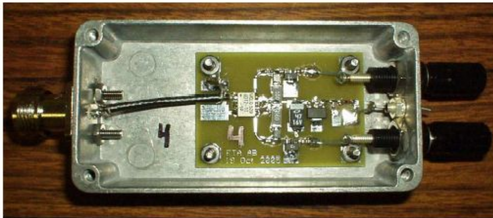
FIG. 5.26 – PRÉ-AMPLIFICADOR MOSTRANDO AS CONECÇÕES DA ANTENA DIPOLO À DIREITA E DO CABO COAXIAL 50 OHMS À ESQUERDA.
