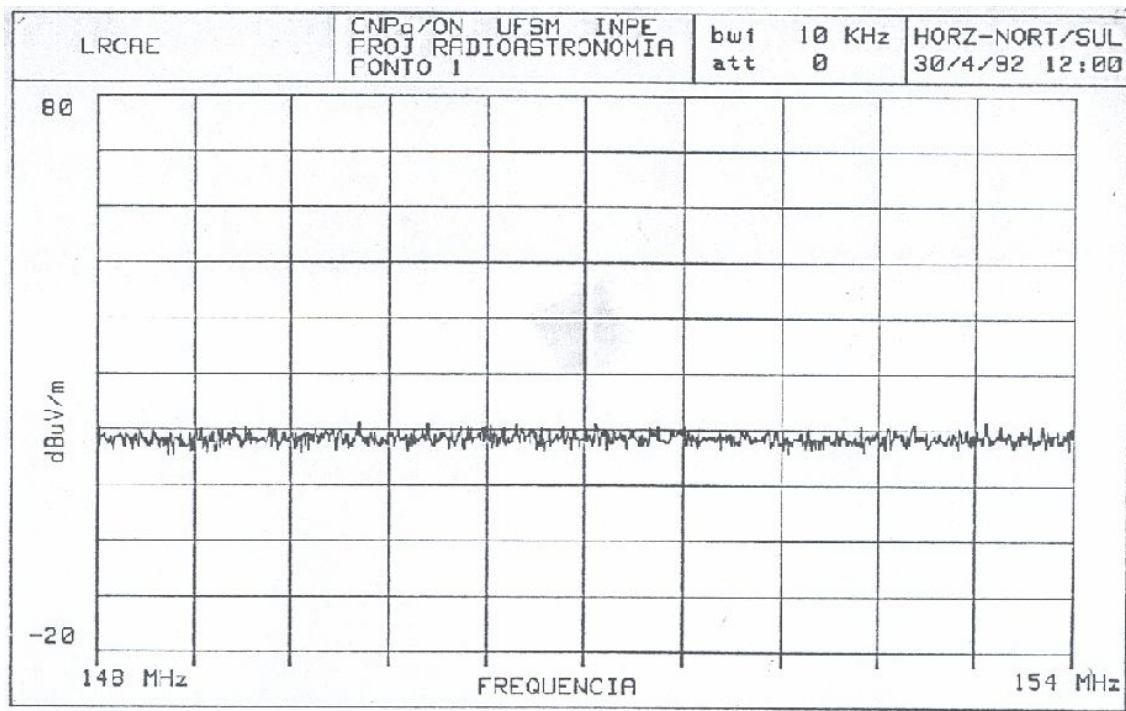
FIG. 5.6 - GRÁFICO DOS SINAIS NA LARGURA DE BANDA DE 148 – 154 MHz, NO OBSERVATÓRIO ESPACIAL DO SUL EM SÃO MARTINHO DA SERRA, RS, EM 1992.
