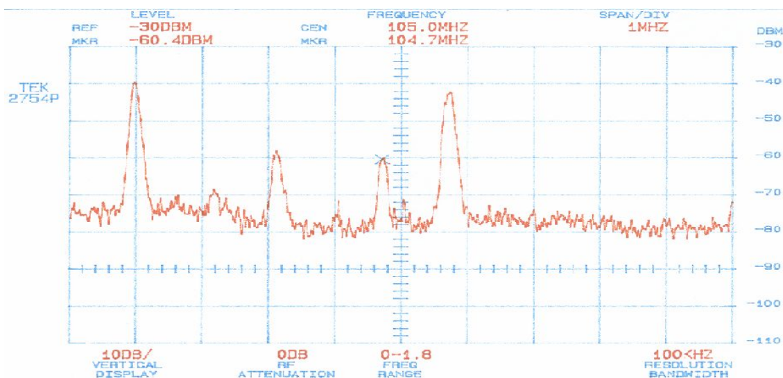
FIG. 5.7 - GRÁFICO DOS SINAIS NA LARGURA DE BANDA DE 100 – 110 MHZ, NO OBSERVATÓRIO ESPACIAL DO SUL EM SÃO MARTINHO DA SERRA, RS, EM 2003.
