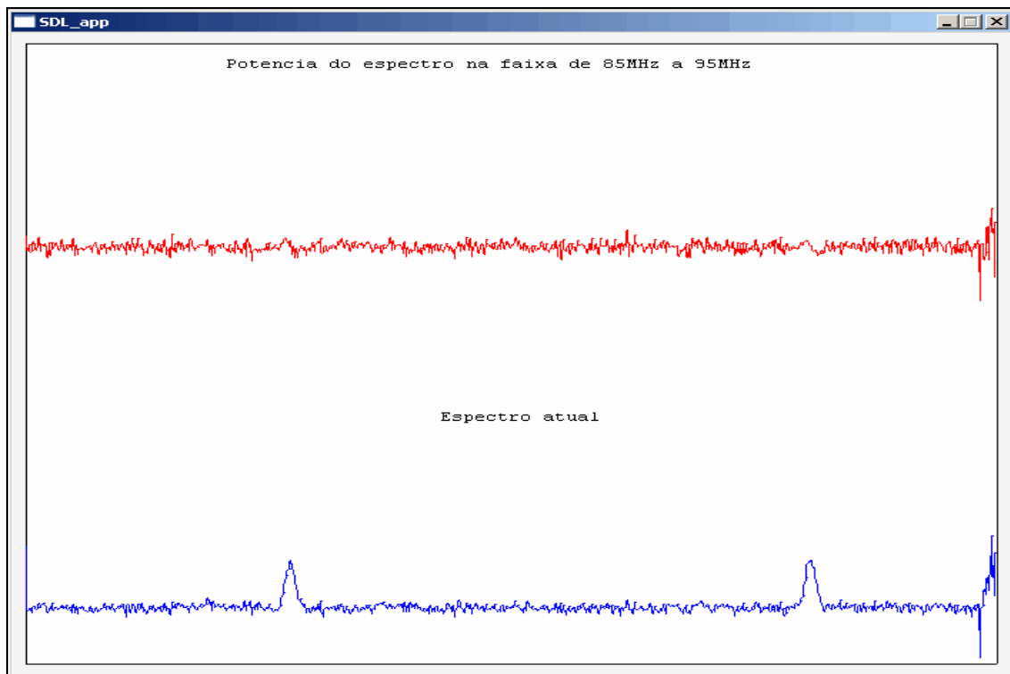
FIG. 2.3.4.1 – GRÁFICOS DO ESPECTRO RECEBIDO (AZUL) E A DIFERENÇA ENTRE A POTÊNCIA ATUAL E A POTÊNCIA COMPARADA (VERMELHO) PARA A FAIXA DE 85 MHZ A 95 MHZ
