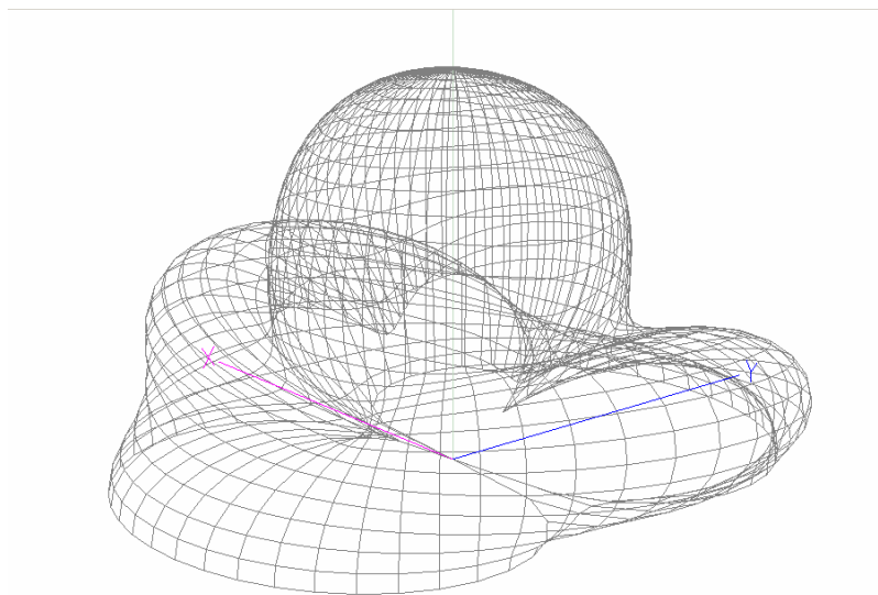
FIG. 5.35 – DIAGRAMA DE IRRADIAÇÃO TRIDIMENSIONAL DA ANTENA DIPOLO SIMILAR À DO SISTEMA LOFAR PARA A FREQUÊNCIA DE 45 MHZ.
