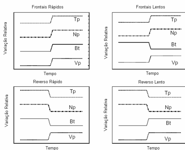
FIGURA 3. 1 - Diagrama ilustrando os perfis de quatro tipos diferentes de choques: Frontais Rápidos, Frontais Lentos, Reversos Rápidos e Reversos Lentos, com a respectiva variação nos parâmetros de plasma e campo magnético interplanetário.
