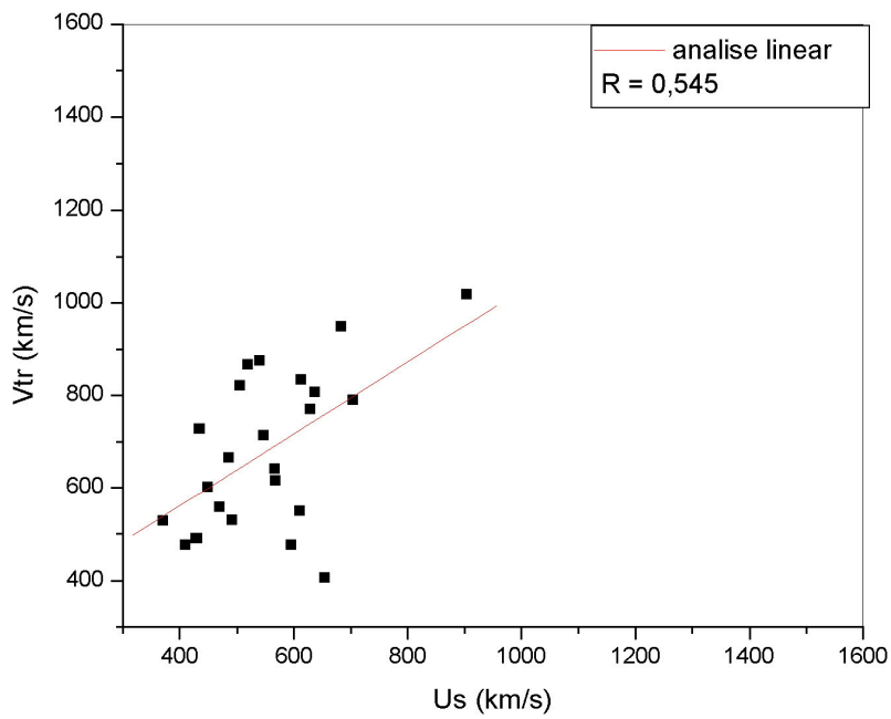
Figura 4.2.1. 4: Relação entre a velocidade de transito e a velocidade instantânea do choque U_s . Obtivemos a equacao V_{tr} = 250,21 + 0,78U_s \pm 148 (km/s)
