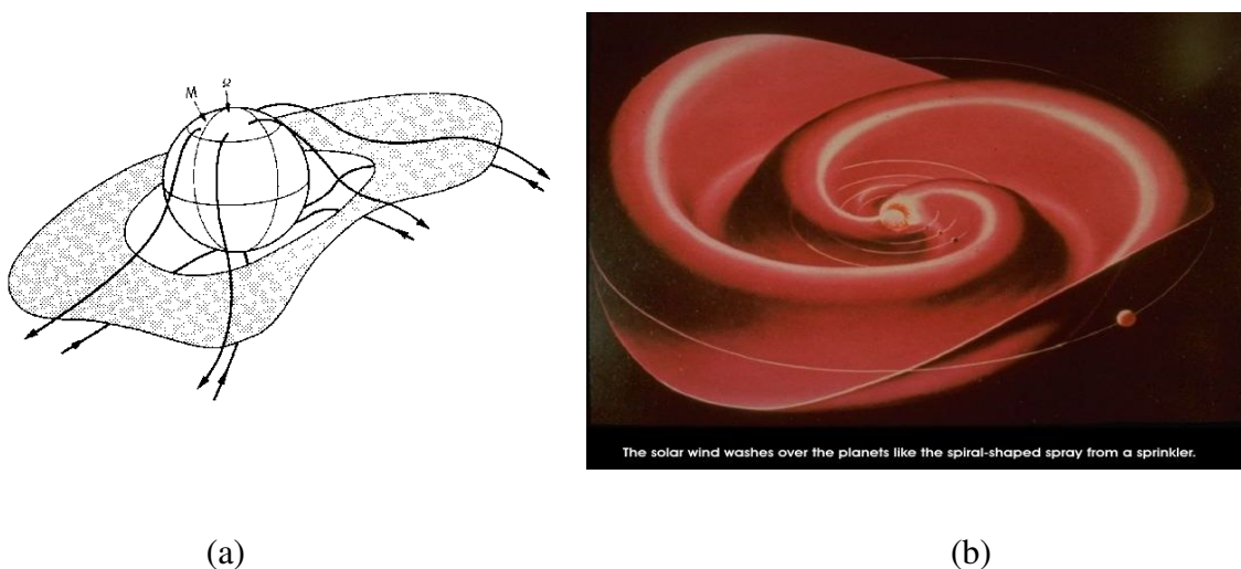
FIGURA 2.4 – (a) Lamina de Corrente Heliosférica – LCH, próxima ao Sol. (b) Aspecto do Campo Magnético Interplanetário.
