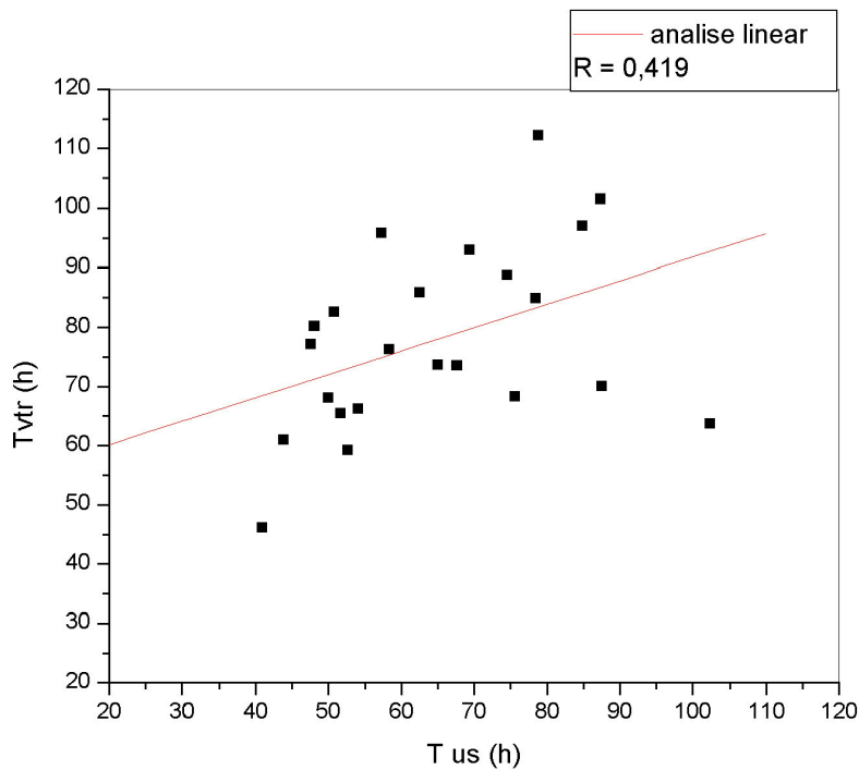
Figura 4.2.1. 5 : Relação entre a velocidade de transito e a velocidade instantânea do choque U_s . Obtivemos a equação T_{tr} = 52,28 + 0,39U_s \pm 14 (h).
