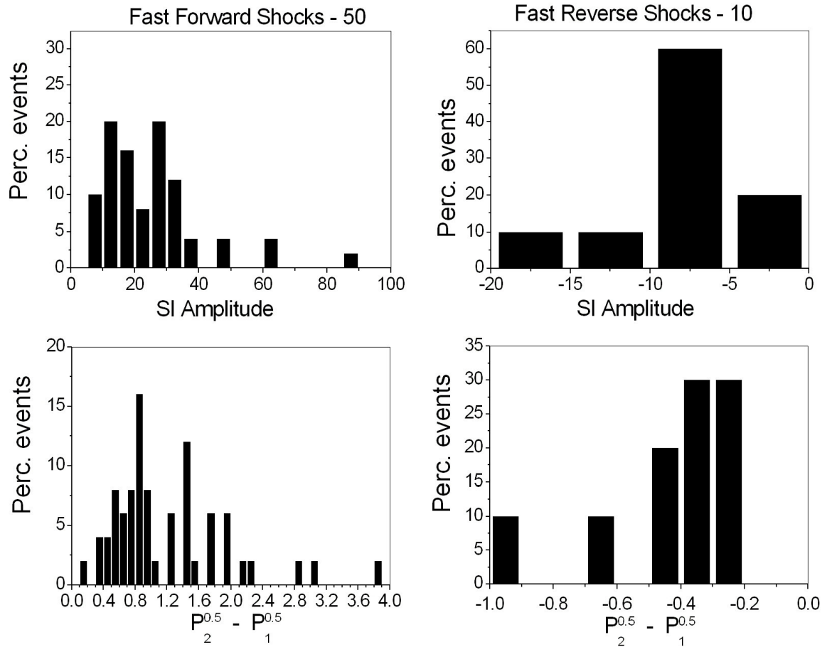
Figura 4.2.3.8: Distribuição do SI e P_2^{1/2} - P_1^{1/2} dos FFS (na esquerda) e dos FRS (na direita).
