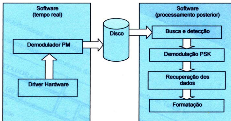
Figura 1: Diagrama para o receptor realizado em software
