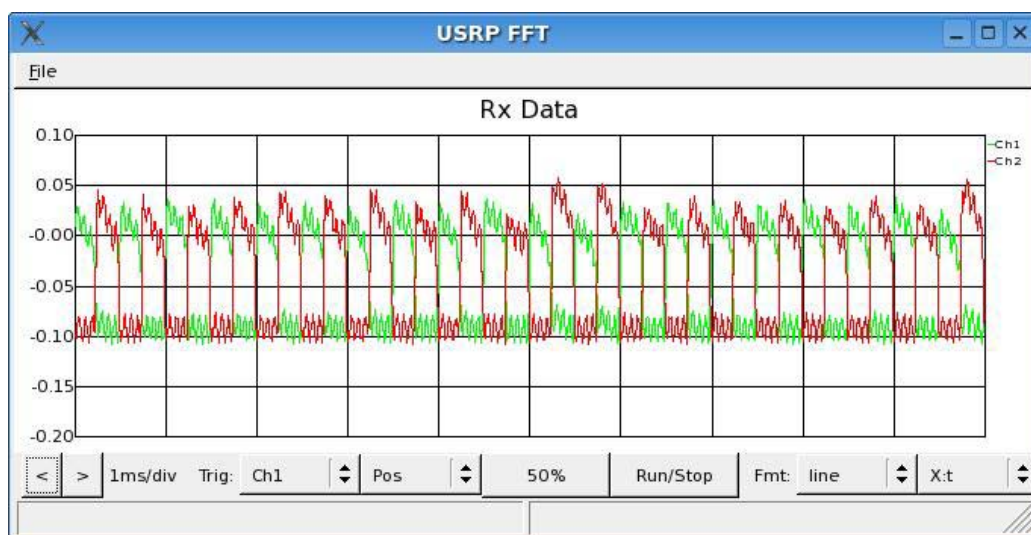
Figura 9: Saída do algoritmo Costas Loop incorporado ao GNU Radio sobre um sinal BPSK
