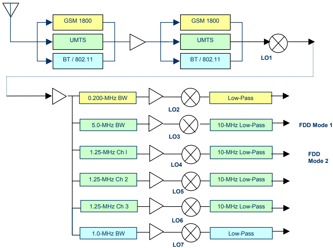
Figura 3: Sistema de recepção Multi-modo baseado em hardware [3]
