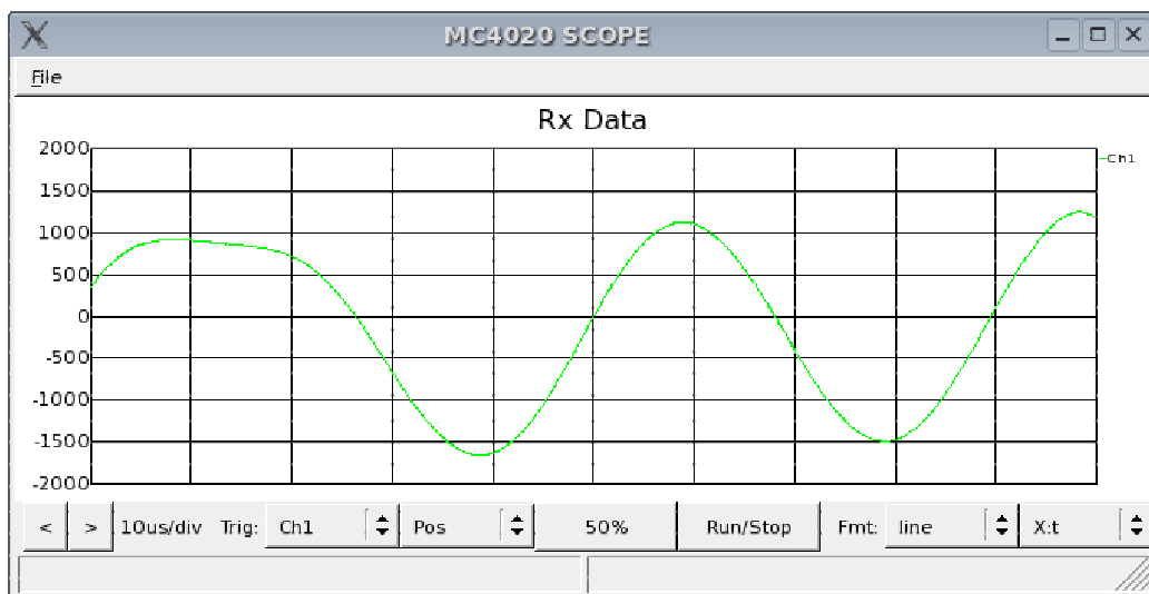
Figura 7: Um sinal modulado em fase captado pela placa MC4020 usando GNU Radio
