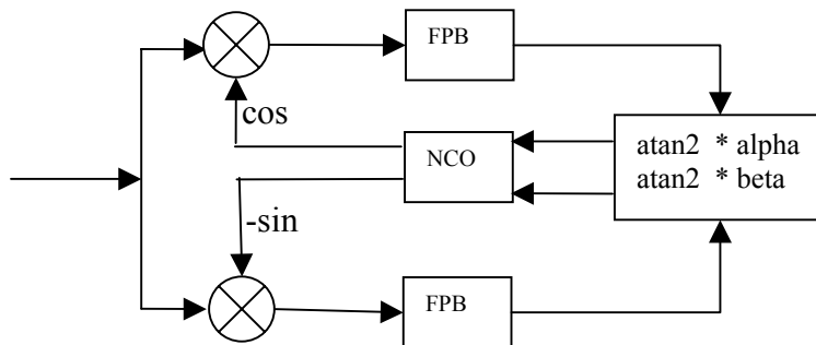
Figura 6: Diagrama de blocos da classe GrCostasLoop do GNU Radio 0.x . O trabalho do módulo é implementado na função Work e consiste em:
