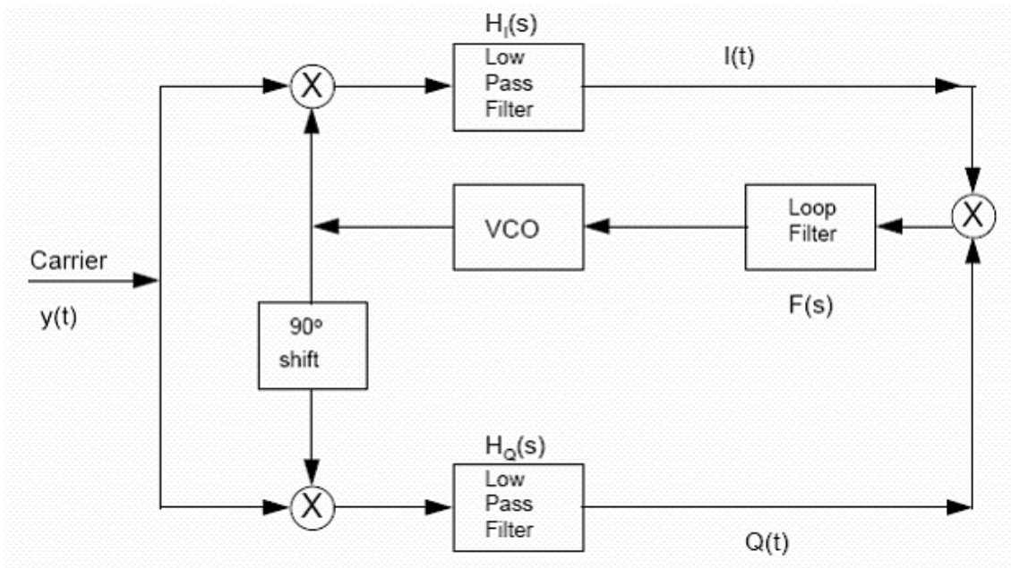
Figura 5: Diagrama de Blocos do Costas Loop [4]
