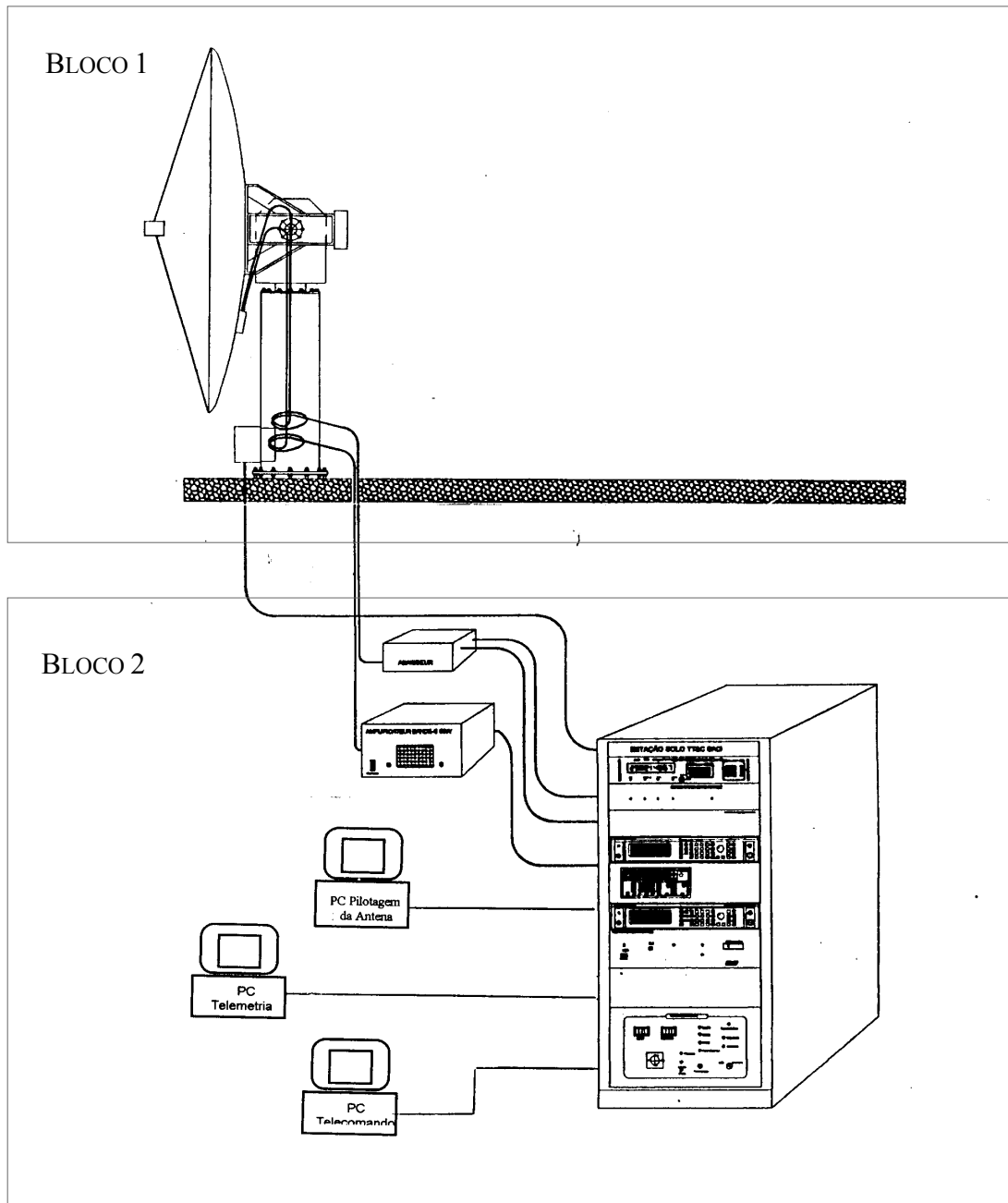
Figura 2: Visão geral da Estação Solo para o micro-satélite SACI-1
