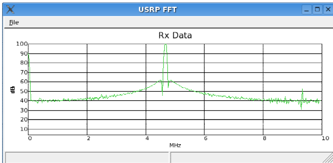
Figura 8: FFT de um sinal modulado em fase captado pela placa MC4020 usando GNU Radio
