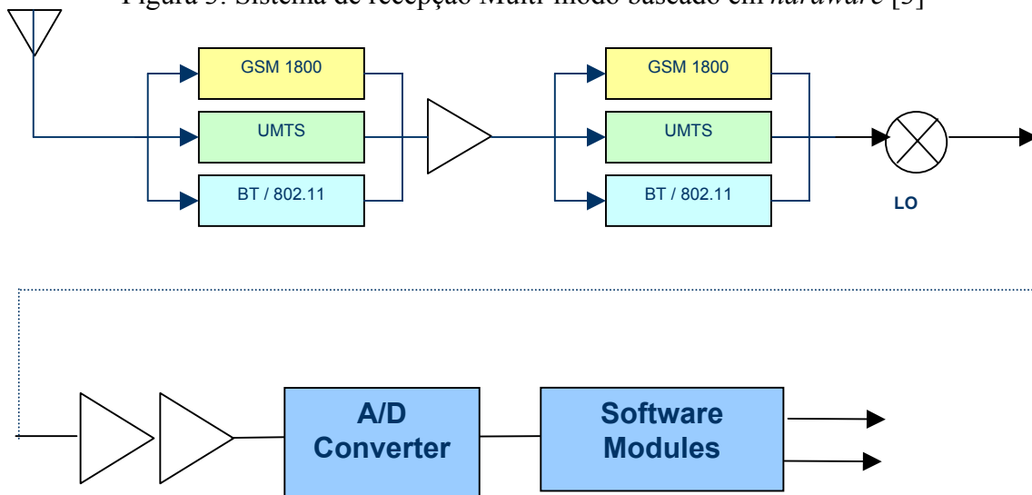
Figura 3: Sistema de recepção Multi-modo baseado em hardware [3]
