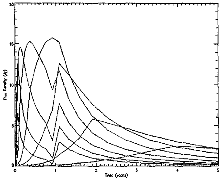
Figura 6 - Modelo de curvas de luz (em várias frequências) para a explosão média de um quasar, obtido neste trabalho
