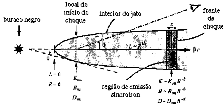
Figura 1 - Ondas de choque em um jato não-cônico (Türler et. al., 2000b)
