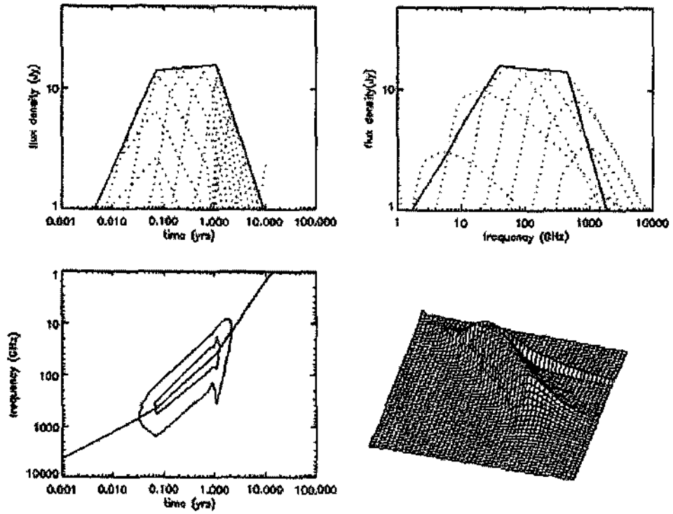
Figura 5 - Evolução logarítmica da explosão média do 3C273 segundo o ajuste de curvas de luz realizado neste trabalho
