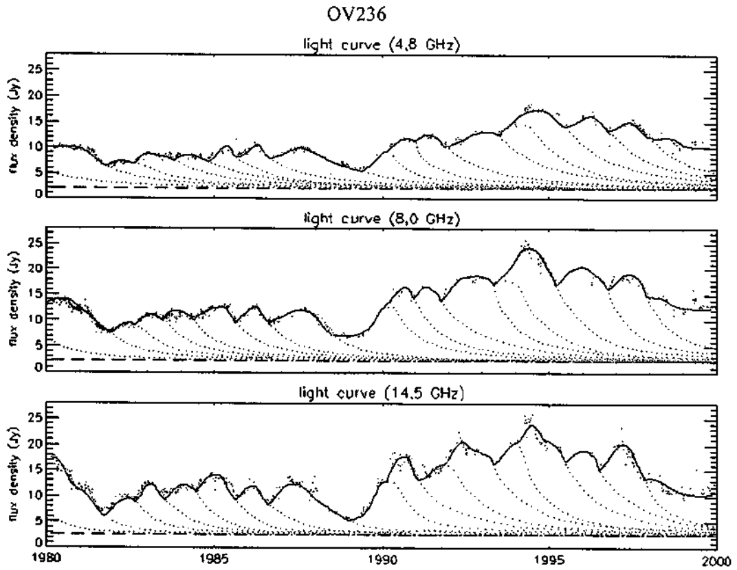
Figura 8 - Decomposição das curvas de luz do OV236, para 4.8, 8.0 e 14.5 GHz
