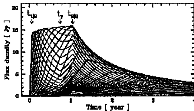
Figura 4 - Modelo de curvas de luz (em várias frequências) da explosão média para o 3C273
