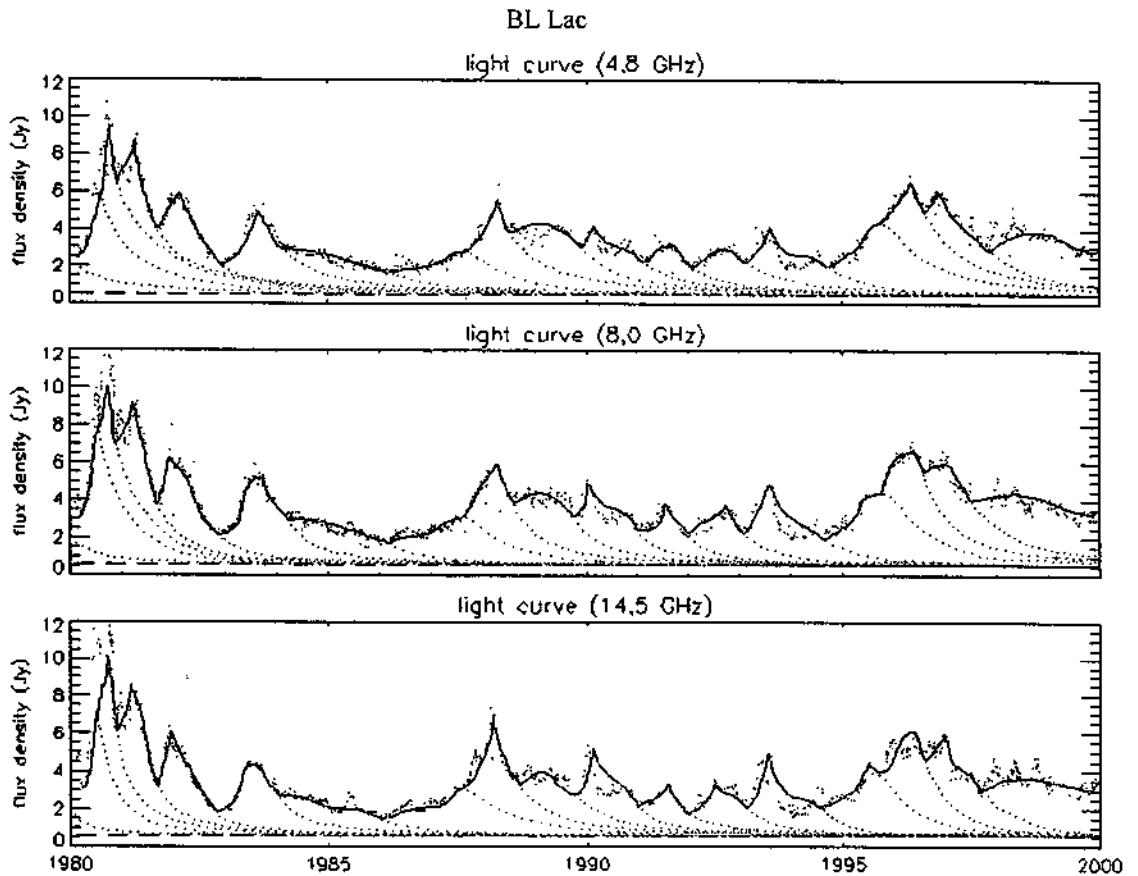
Figura 9 - Decomposição das curvas de luz do BL Lac, para 4.8, 8.0 e 14.5 GHz
