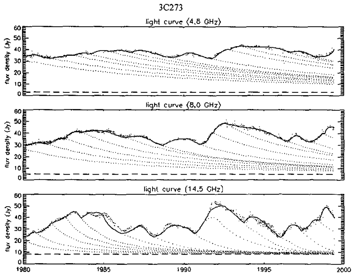
Figura 7 - Decomposição das curvas de luz do 3C273, para 4.8, 8.0 e 14.5 GHz, em séries de explosões modeladas neste trabalho
