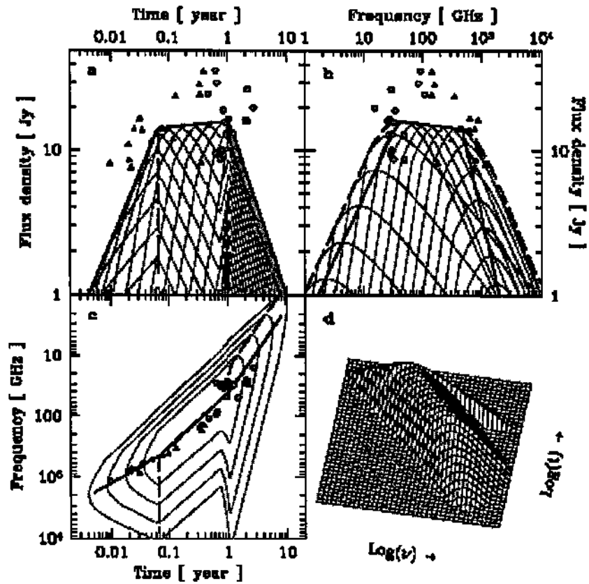
Figura 3 - Evolução logarítmica da explosão média para o 3C273 (Türler et. al., 2000b)
