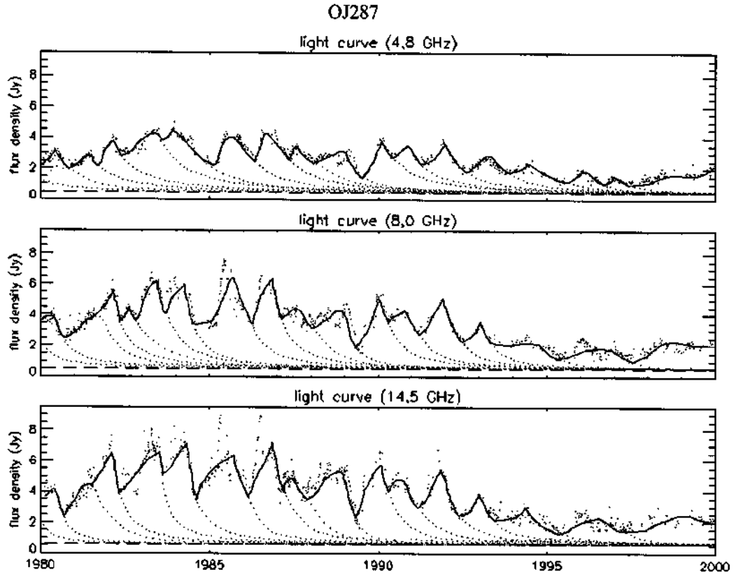
Figura 10 - Decomposição das curvas de luz do OJ287, para 4.8, 8.0 e 14.5 GHz
