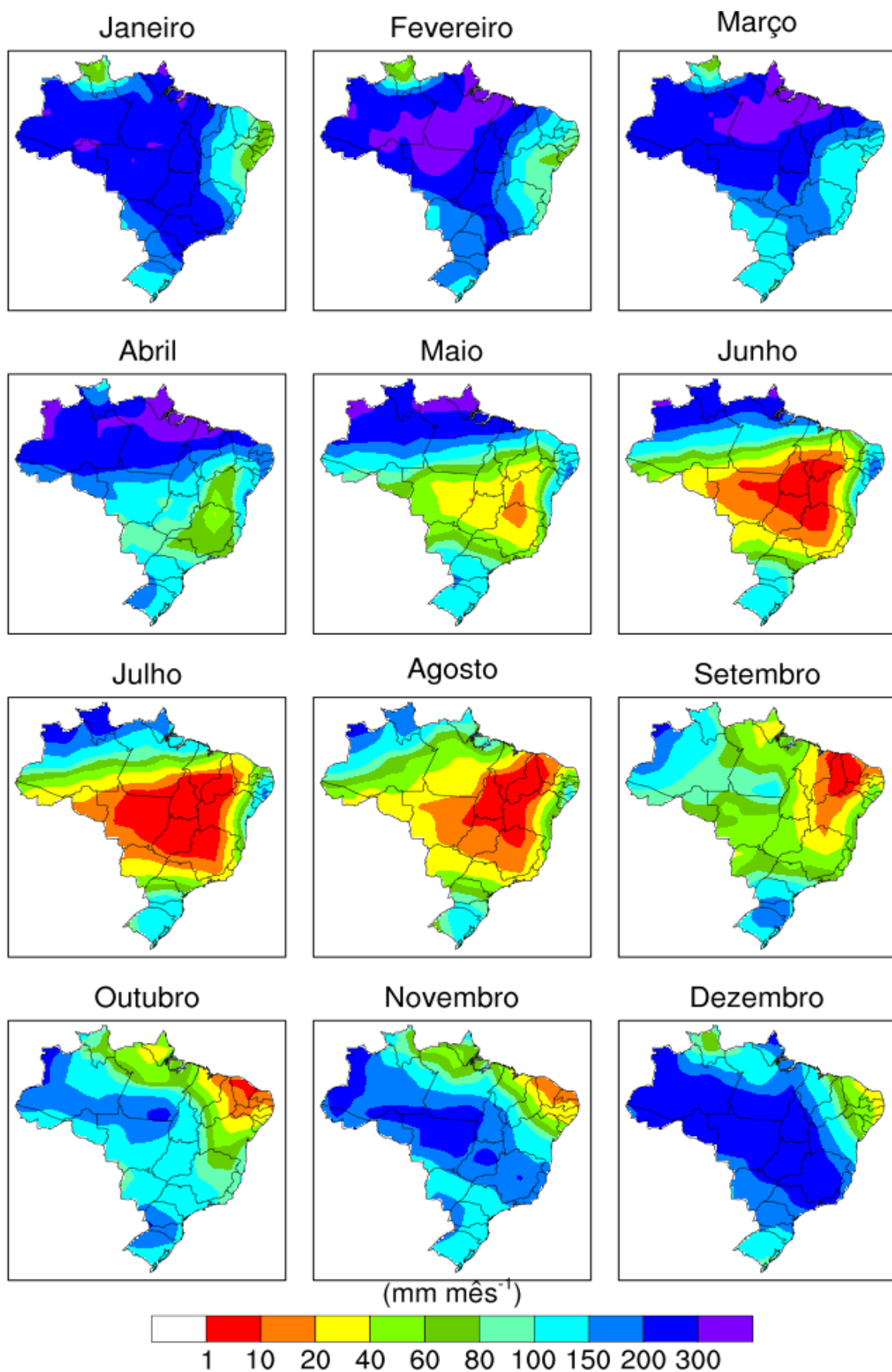
Figura 3. Normal climatológica de precipitação (1981 a 2010) do Brasil. A unidade está em \text{mm mês}^{-1} .
