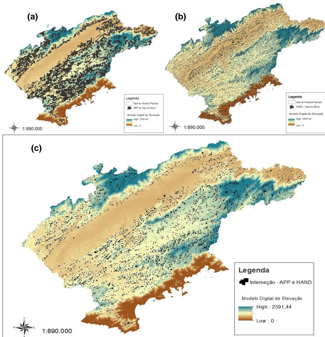
Figura 4. Resultados: (a) Mapeamento das Áreas de Preservação Permanente em Topo de Morros; (b) Topos de Morro extraídos a partir do algoritmo HAND; (c) Áreas de acertos do algoritmo HAND.
