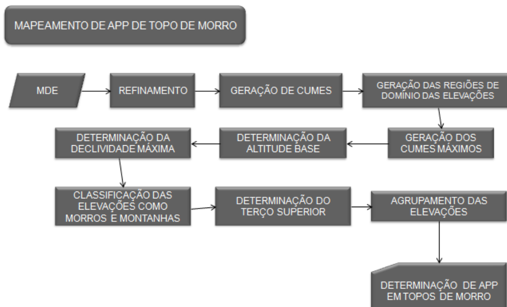
Figura 2. Método para determinação das APPs em topos de morro. Fonte: Adaptada Peluzio et. al., (2010)
