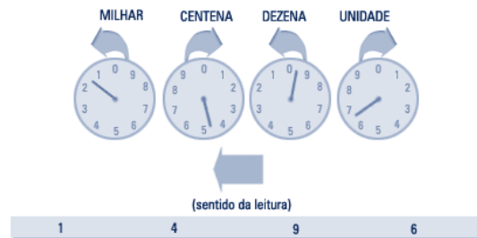
Figura 2.1.1. Medidor Analógico[5].
