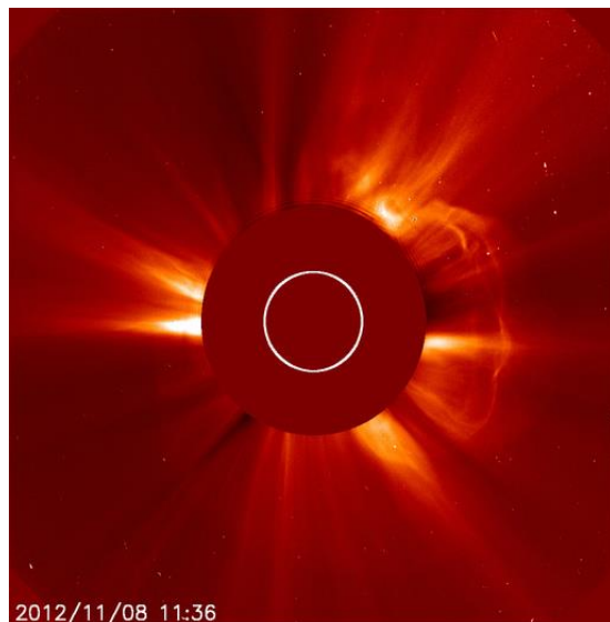
Figura 5.1.9: Imagem do C2, obtida pelo SOHO.
