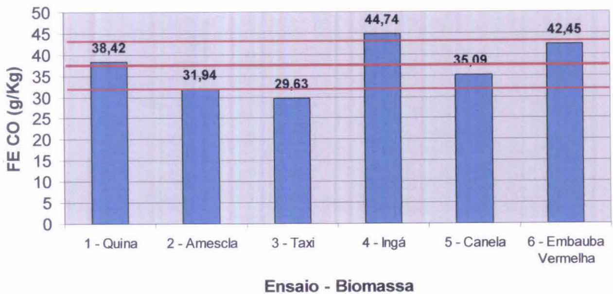
Figura 13 – Fatores de Emissão de CO.
