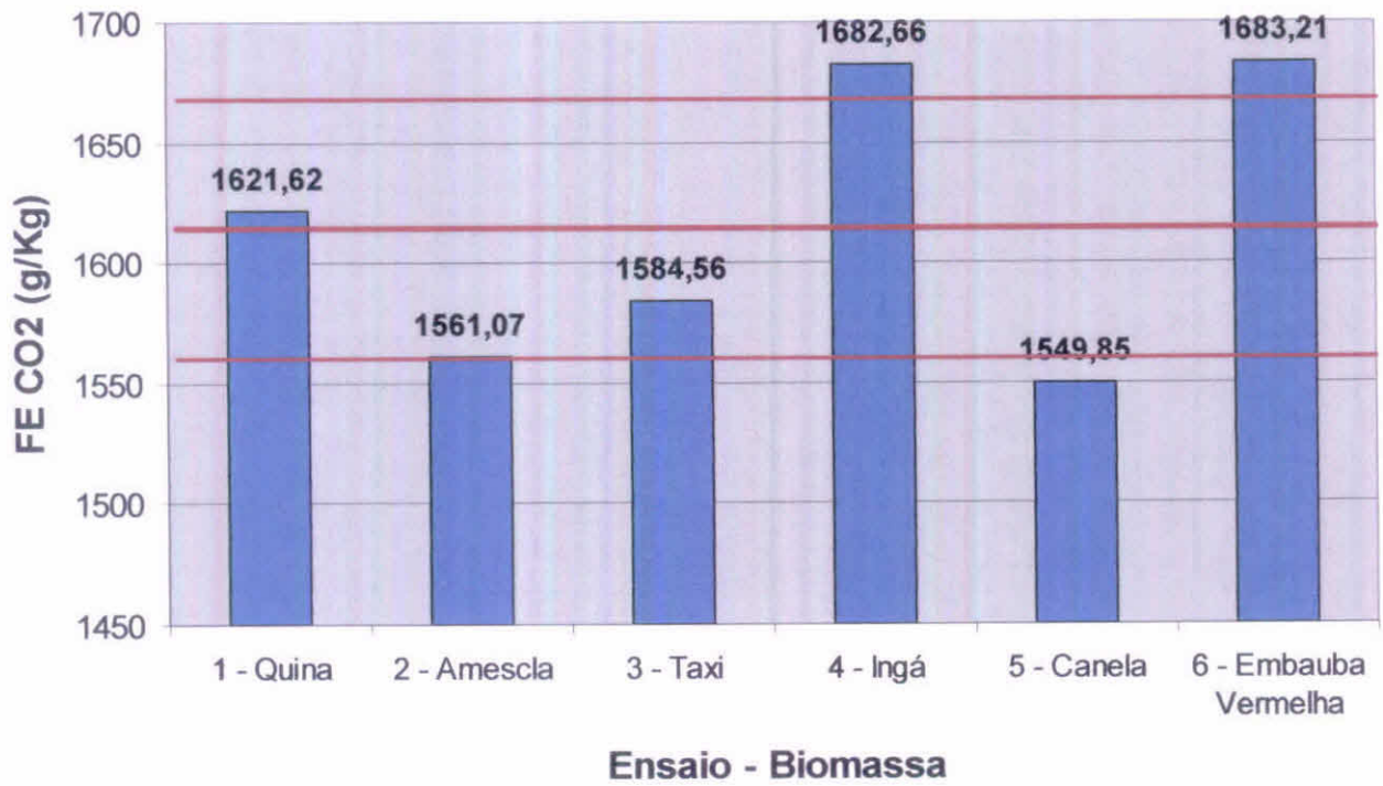
Figura 12 – Fatores de Emissão de CO 2 .
