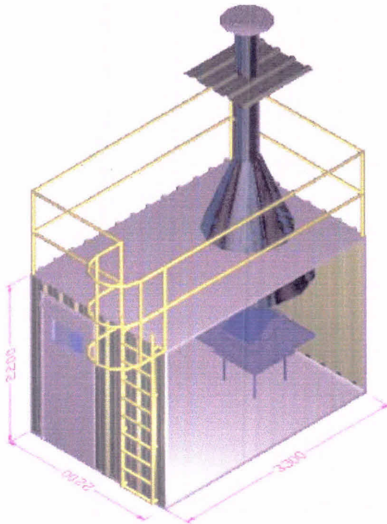
Figura 1 - Desenho ilustrativo do dispositivo experimental.
