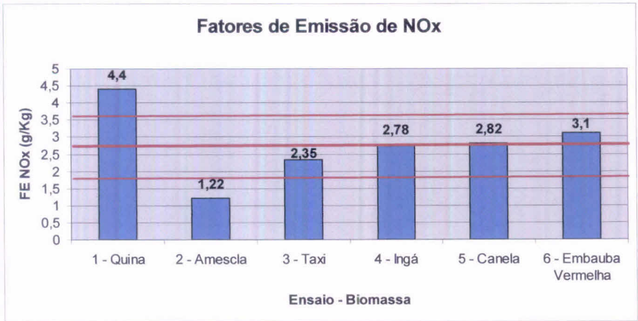
Figura 14 – Fatores de Emissão de NO x .
