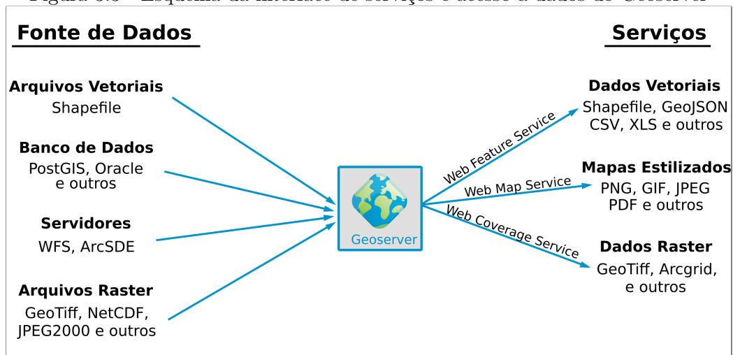
Figura 3.3 - Esquema da interface de serviços e acesso a dados do Geoserver
