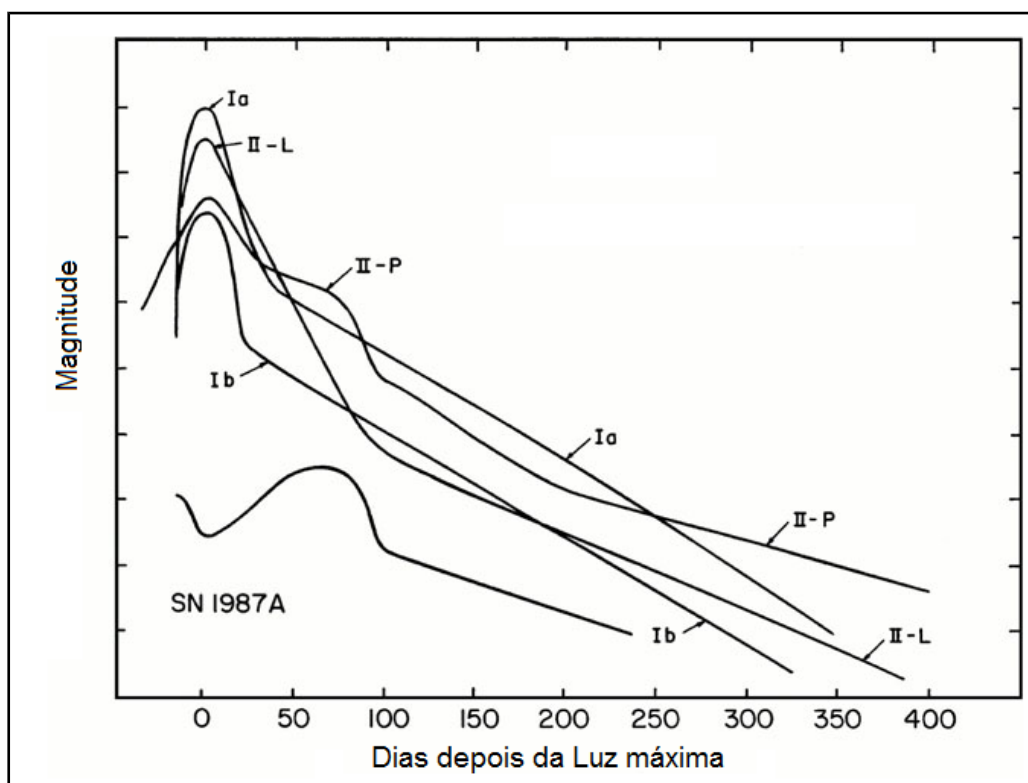
Figura 2.11 – Diversidade das Curvas de luz de supernovas
