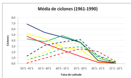
Figura 1- Número médio de ciclôgeneses durante o período de 1961-1990 por faixa de latitude para inverno (azul), primavera (verde), verão (vermelho) e outono (amarelo), obtido a partir dos dados da Reanálise 1 do NCEP/NCAR (linha contínua) e os dados do modelo Eta (linha tracejada).
