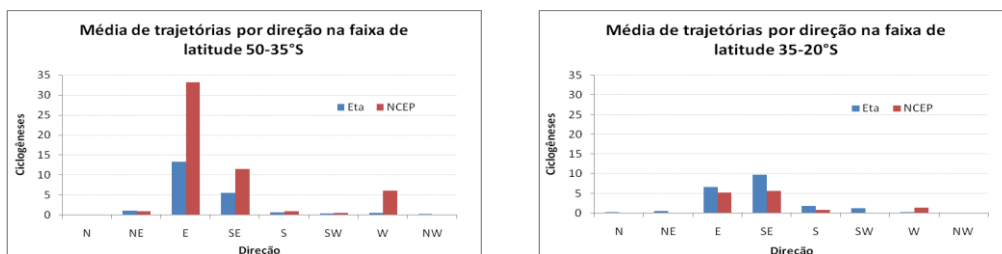
Figura 2 - Média de trajetórias dos ciclones por direção no período de 1961 a 1990, a partir de dos dados da Reanálise 1 do NCEP/NCAR (vermelho) e dos dados do modelo Eta (azul) para as faixas de latitude: (a) 50-35°S e (b) 35-20°S.
