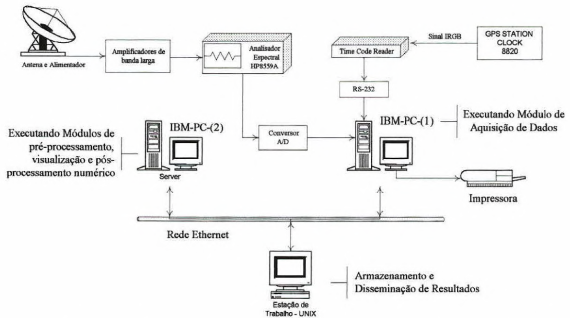
Fig. 1 – Diagrama de blocos representando o Brazilian Solar Spectroscop (BSS) de alta sensibilidade (~ 2 ufs), alta resolução espectral (3 MHz) e alta resolução temporal (10 - 1000 ms).
