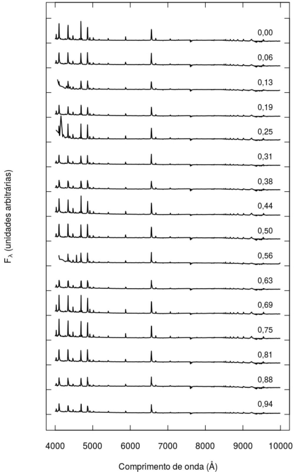
Figura 4.1 - Os 16 espectros de fluxo para AM Her obtidos ao longo de um período orbital, deslocados entre si de 50 unidades. A fase orbital é mostrada à direita em cima de seus respectivos espectros.
