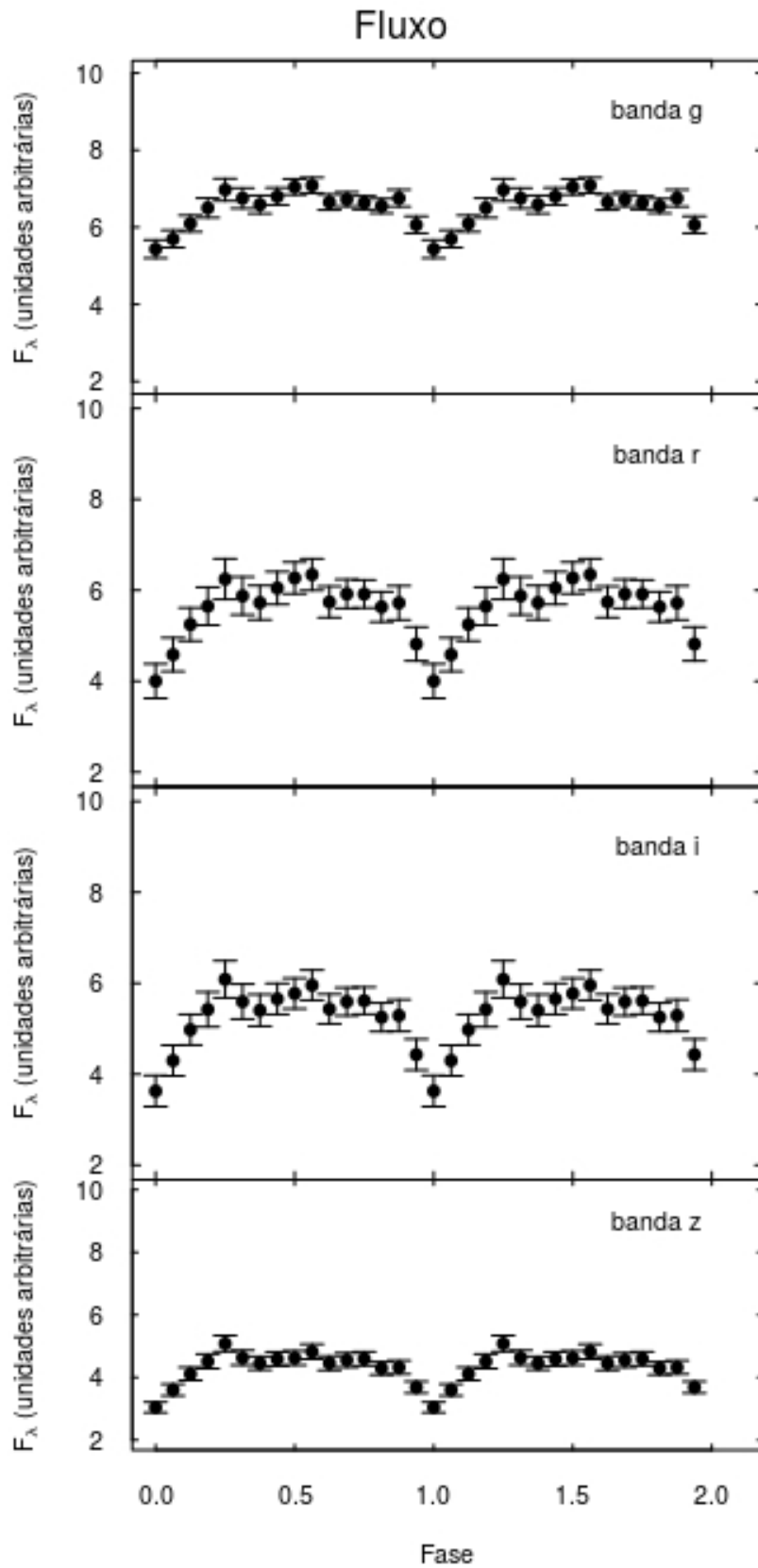
Figura 4.25 - Diagramas de fases para os filtros g, r, i e z do Sloan Digital Sky Survey a partir dos dados de fluxo.
