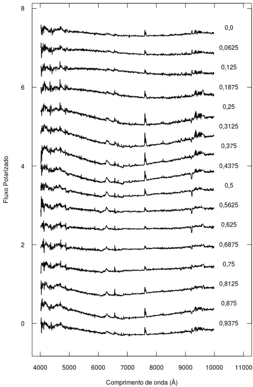
Figura 4.8 - Fluxo polarizado ao longo do ciclo orbital em unidades arbitrárias de fluxo. A fase é mostrada a direita de cada espectro.
