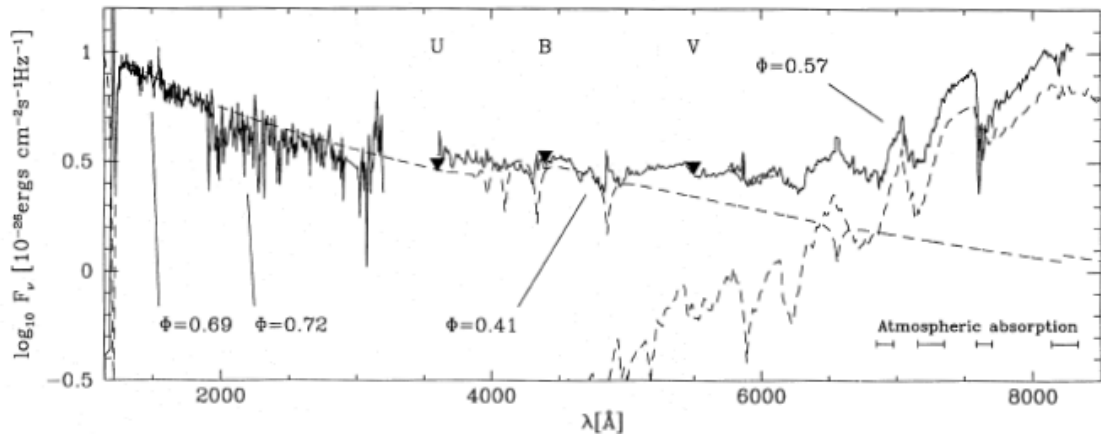
Figura 1.12 - Espectro de fluxo para AM Her ajustados com uma curva modelo de atmosfera de anã branca com temperatura de 24.000 K e com um espectro de uma estrela do tipo M4.
