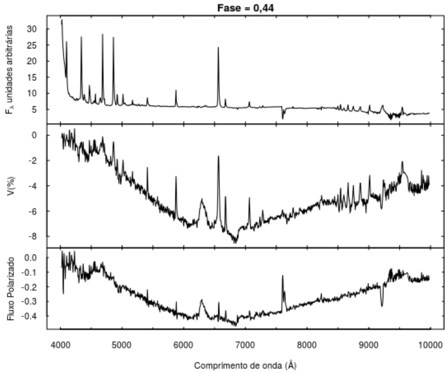
Figura 4.16 - Fluxo, polarimetria e fluxo polarizado para a fase 0,44.
