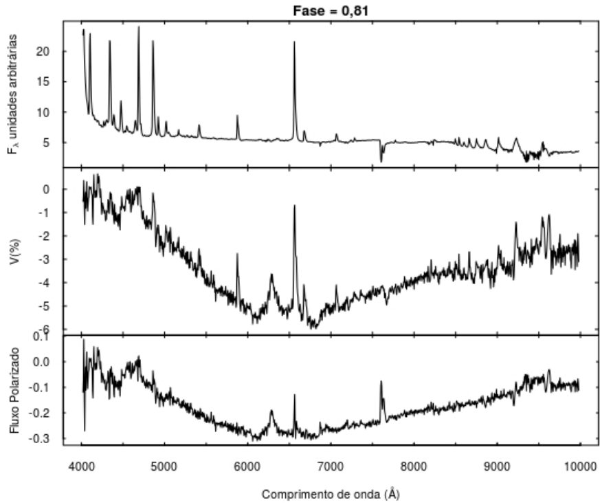
Figura 4.22 - Fluxo, polarimetria e fluxo polarizado para a fase 0,81.
