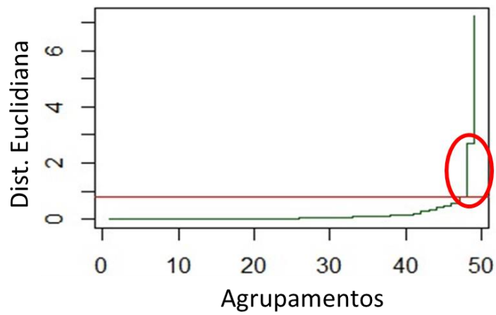
Figura 4.7. Exemplo de um gráfico de seqüências de agrupamento. O platô vertical destacado pelo elipse em vermelho ilustra o limiar que pode ser utilizado como limiar de similaridade.
