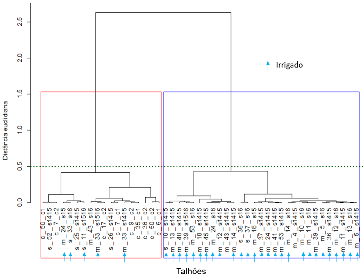
Figura 5.16. Dendrograma da análise interespecífica baseada nos valores de NDVI, com todos os talhões.
