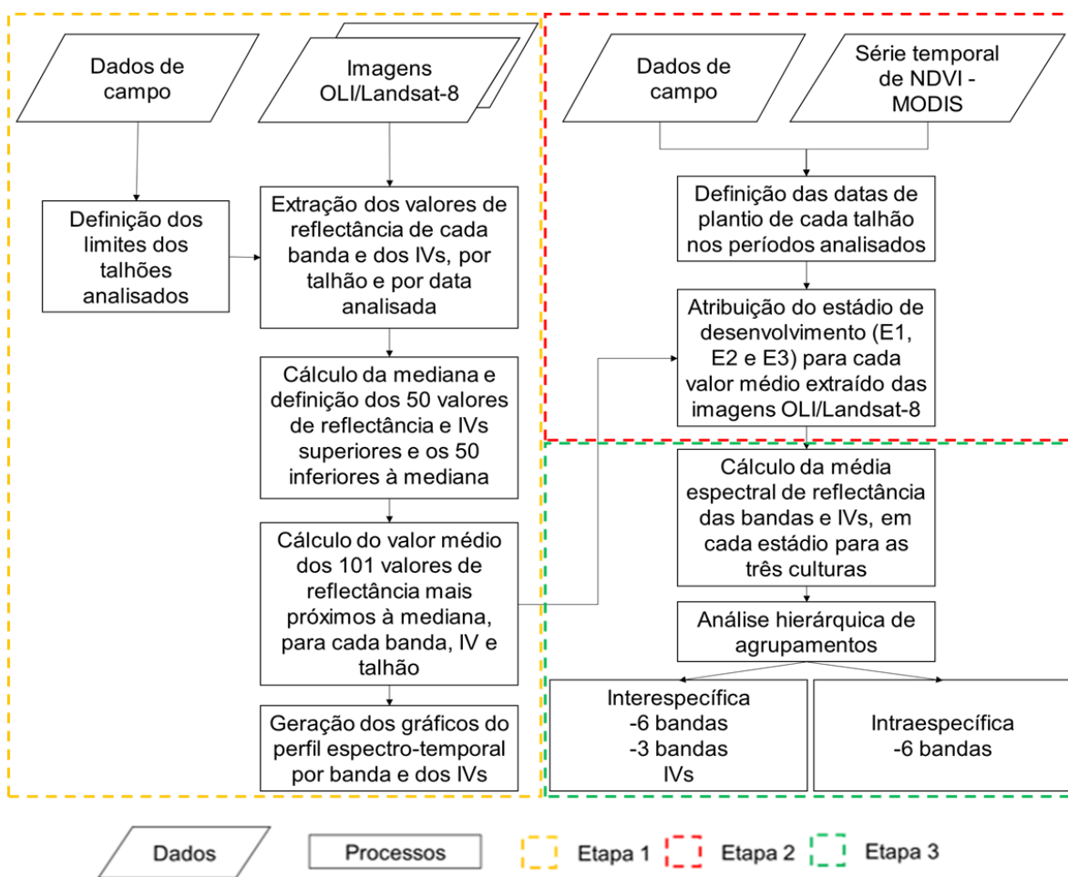
Figura 4.1. Fluxograma das etapas metodológicas efetuadas na presente pesquisa.
