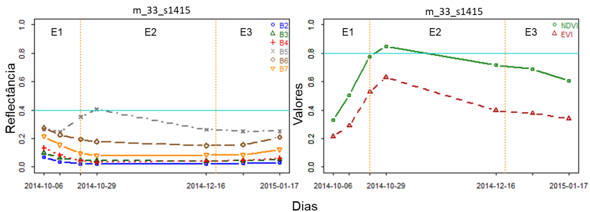
Figura 5.10. Perfil espectro-temporal do talhão de milho Id 33 cultivado durante a safra 2014/15. Os limiares adotados (linhas horizontais azuis claras) de 0.4 e 0.8 foram estabelecidos com base nos perfis espectro-temporais. A linha vertical laranja indica a separação entre os estádios E1 e E2.
