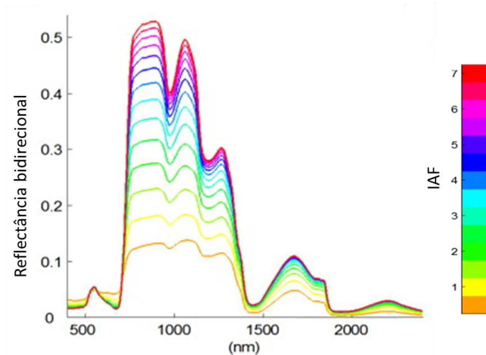
Figura 2.2. Valores de reflectância nas diferentes faixas espectrais de acordo com o aumento do IAF.
