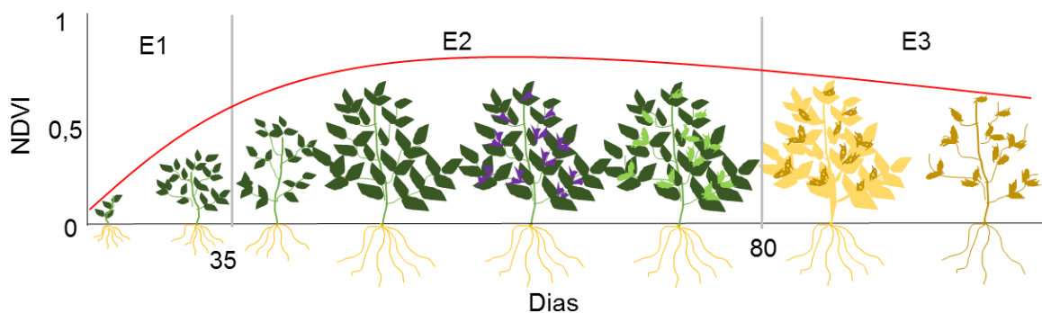
Figura 4.6. Estádios de desenvolvimento da soja com os respectivos intervalos de dias.
