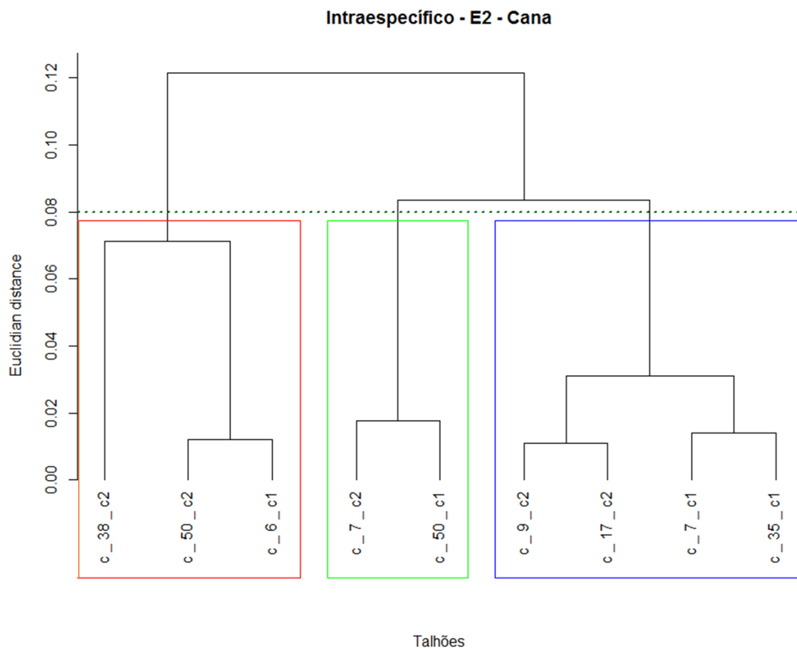
Figura 5.21. Dendrograma da análise intraespecífica de talhões de cana baseada em todas as bandas.
