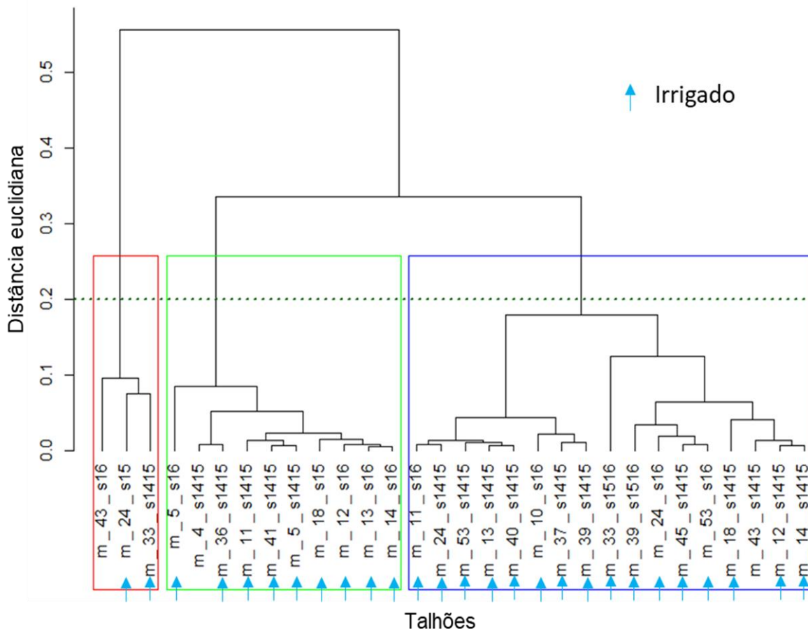
Figura 5.19. Dendrograma da análise intraespecífica de talhões de milho baseada em todas as bandas.
