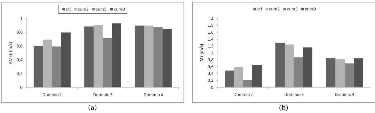
Figura 4 – Índices estatísticos velocidade do vento para os domínios das diferentes parametrizações de convecção ( cumulus ): (a) RMSE e (b) ME.
