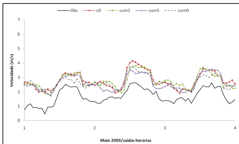
Figura 5 - Evolução temporal da velocidade do vento para o modelo WRF para as diferentes configurações de convecção (cumulus): (a) Domínio 2; (b) Domínio 3 e (c) Domínio 4.
