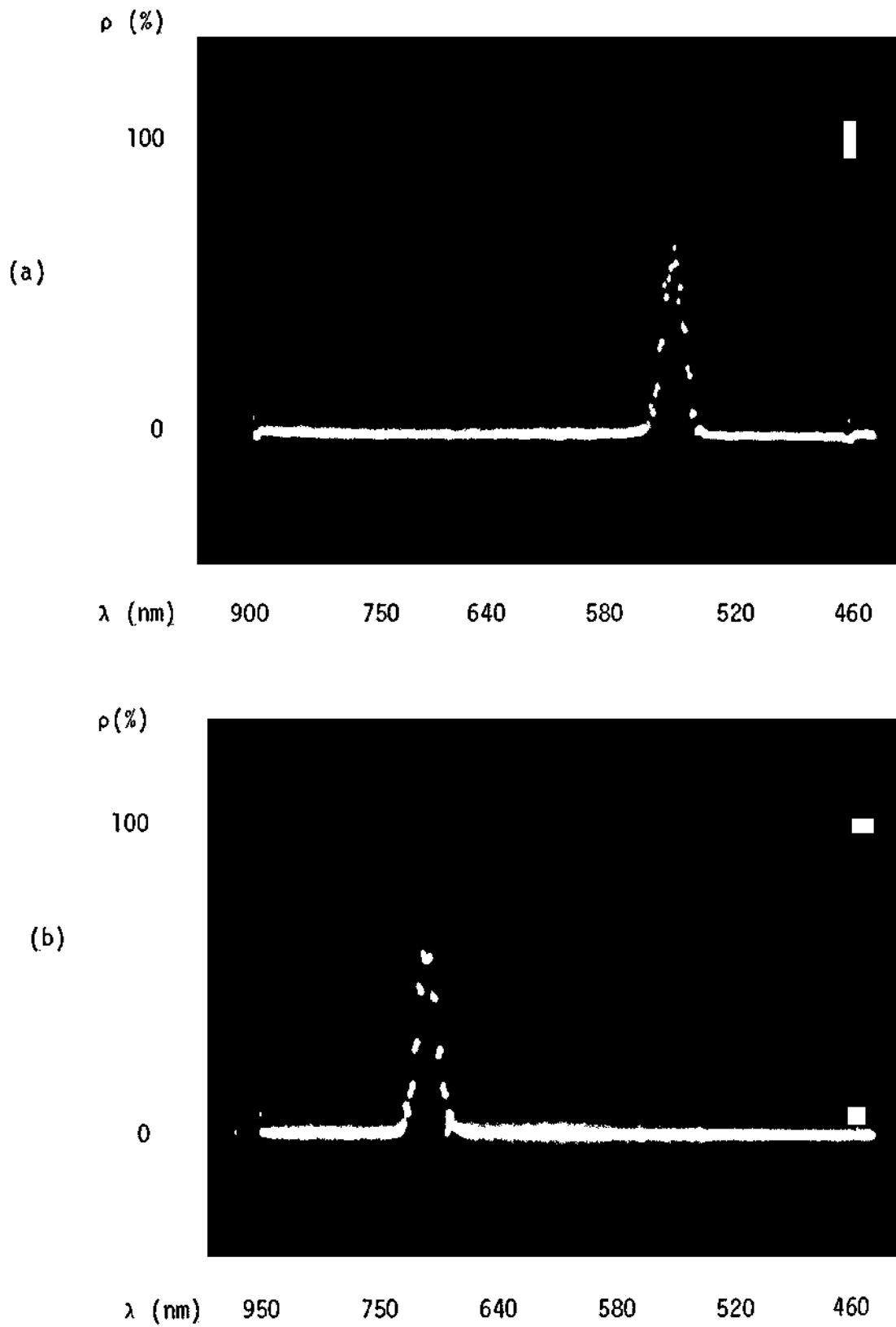
Fig. 6.3 - Curvas de transmitância de filtros de inteferência com Banda de 10 nm.
