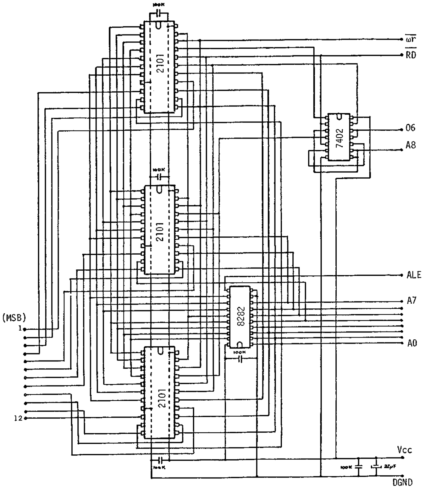
Fig. D.3 - Memória intermediária.
