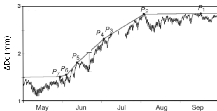
Figura 3.5 - Metodologia extrair os valores de crescimento do tronco (Cr). P1 a P7 = representam os máximos de \Delta D_c
