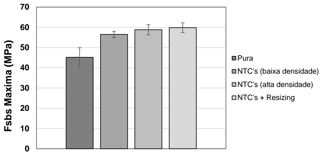
Figura 4.19 – Tensão de Cisalhamento ( F_{sbs} ) de amostras puras, fibras com baixa e alta densidade de NTC's e fibras com NTC's e camada de resizing.
