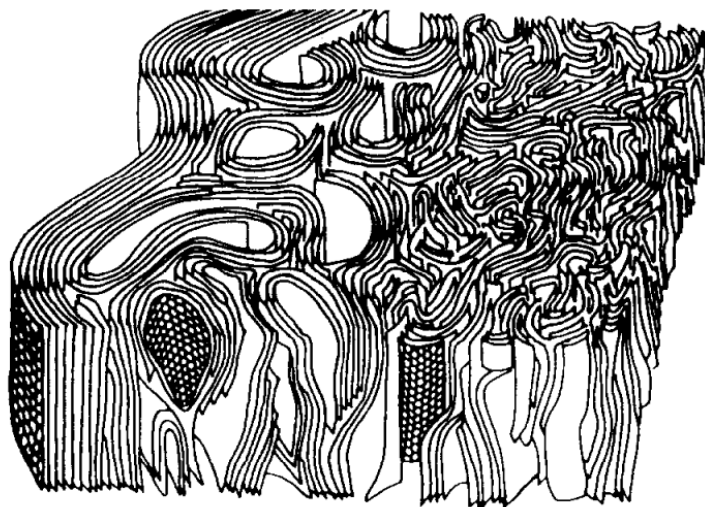
Figura 2.2 – Estrutura da Fibra de Carbono proposta por Johnson.
