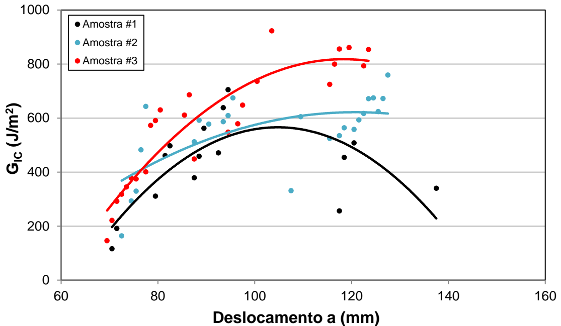
Figura C.1 - Curvas R a partir dos ensaios de Tenacidade à Fratura no Modo I, para amostras puras.
