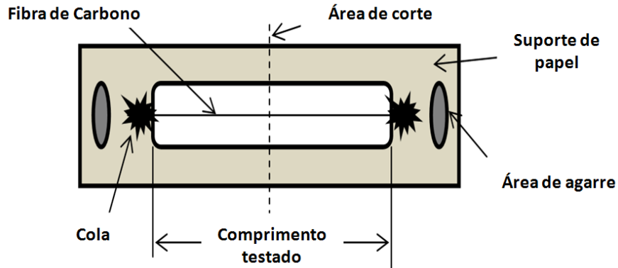
Figura 3.6 – Ilustração esquemática da montagem das amostras.
