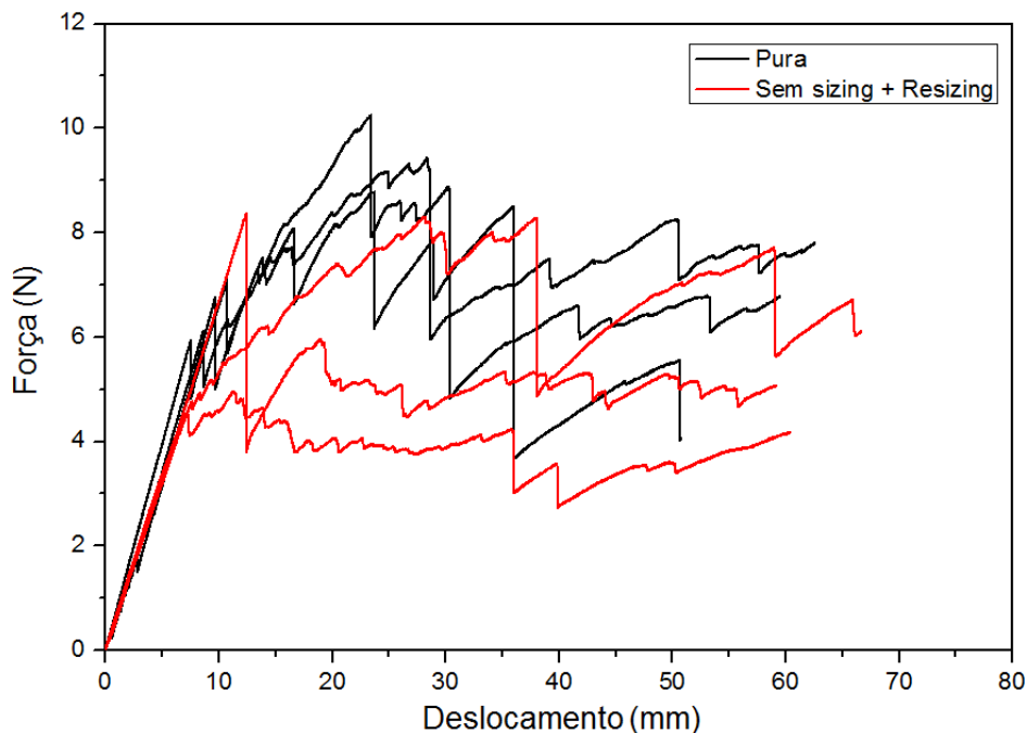
Figura 4.31 – Curvas de Força em função do Deslocamento a partir dos ensaios de Tenacidade à Fratura no Modo I, para amostras puras, sem sizing e com resizing.
