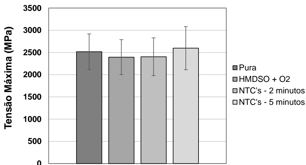
Figura 4.9 – Tensão Máxima de ruptura no ensaio de tração longitudinal em cada etapa do tratamento.
