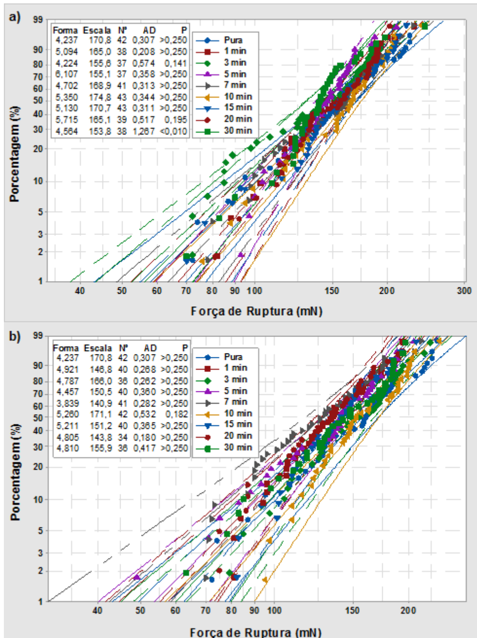
Figura A.1 - Plotagem de probabilidade dos resultados do teste de tração em monofilamentos expostos a temperatura de: a) 650 °C e b) 800 °C.
