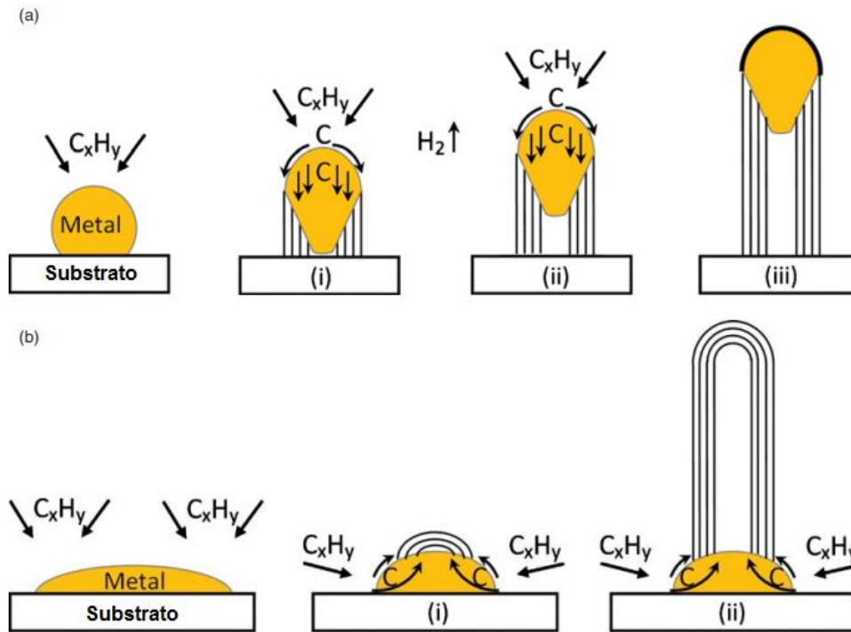
Figura 2.16 – Mecanismos de crescimento para NTC's: (a) modelo tipo ponta, (b) modelo tipo base.
