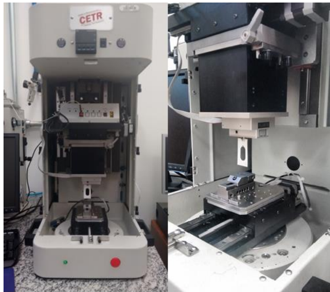
Figura 3.5 – Tribômetro CETR adaptado para Teste de Tração de monofilamento.
