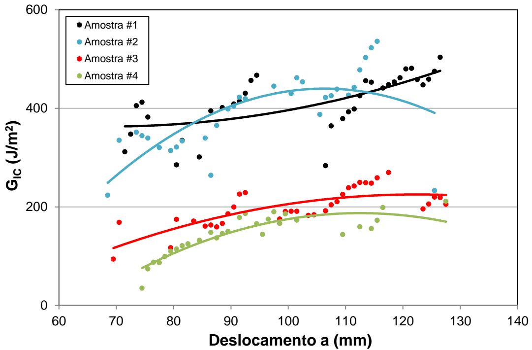
Figura C.3 - Curvas R a partir dos ensaios de Tenacidade à Fratura no Modo I, para amostras com NTC's e resizing.
