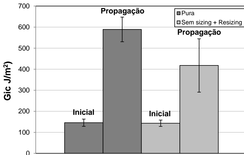
Figura 4.32 –Taxa de Liberação de Energia Inicial e Total a partir dos ensaios de Tenacidade à Fratura no Modo I, para amostras puras, sem sizing e com resizing.
