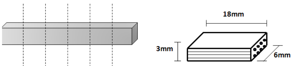
Figura 3.12 – Corte e dimensões das amostras para ensaio de cisalhamento interlaminar.
