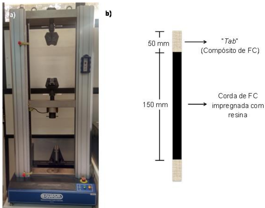
Figura 3.7 – a) Máquina de teste de tração Equilam EQTB-20 e b) Esquema de montagem das amostras.
