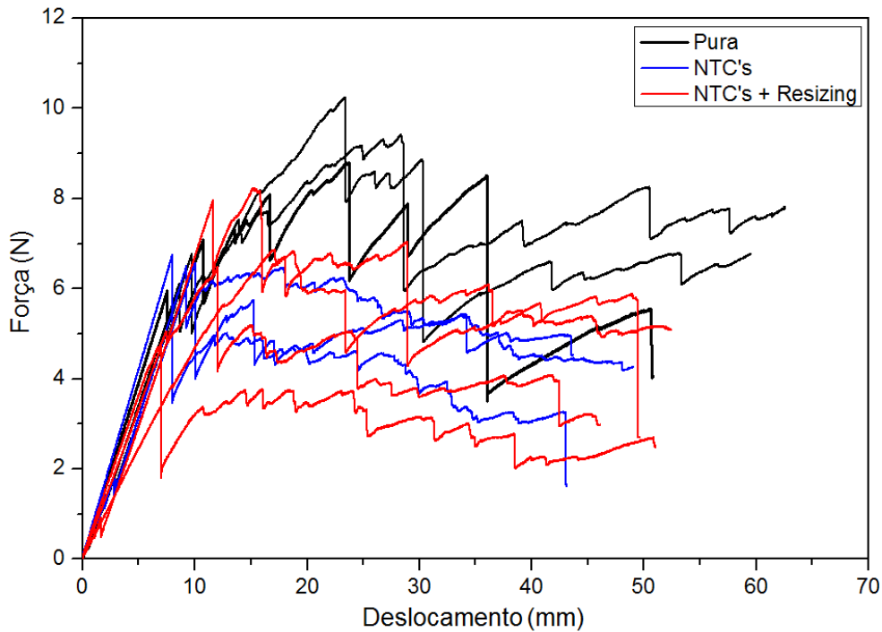
Figura 4.24 – Curvas de Força em função do Deslocamento a partir dos ensaios de Tenacidade à Fratura no Modo I, para amostras puras, com NTC's e NTC's com resizing.
