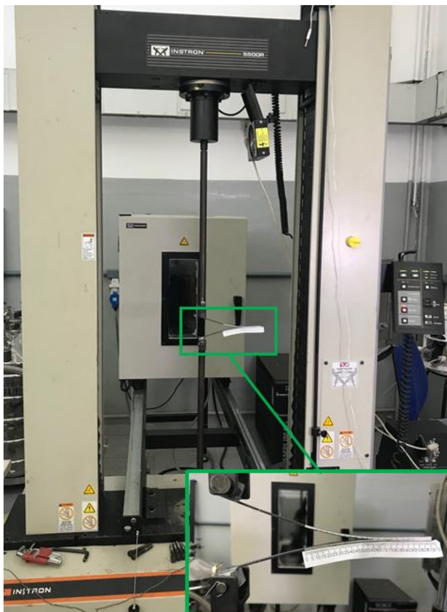
Figura 3.14 – Máquina Instron para ensaio da tenacidade à fratura.
