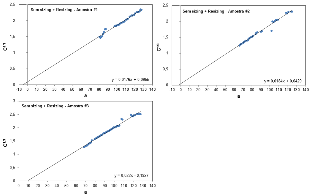
Figura B.4 – Curvas de Correção do Método MBT para amostras sem sizing e resizing
