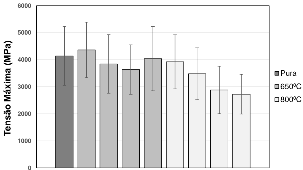
Figura 4.4 – Tensão de Ruptura alcançadas pelas FC's com crescimento de NTC's a 650 °C e 800 °C.
