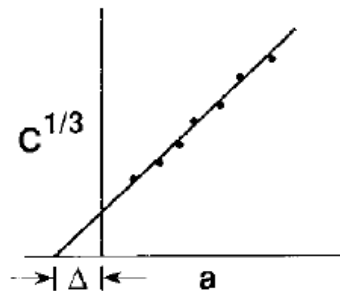
Figura 2.22 – Gráfico utilizado para determinar “ \Delta ” na Teoria de Feixe Modificado.
