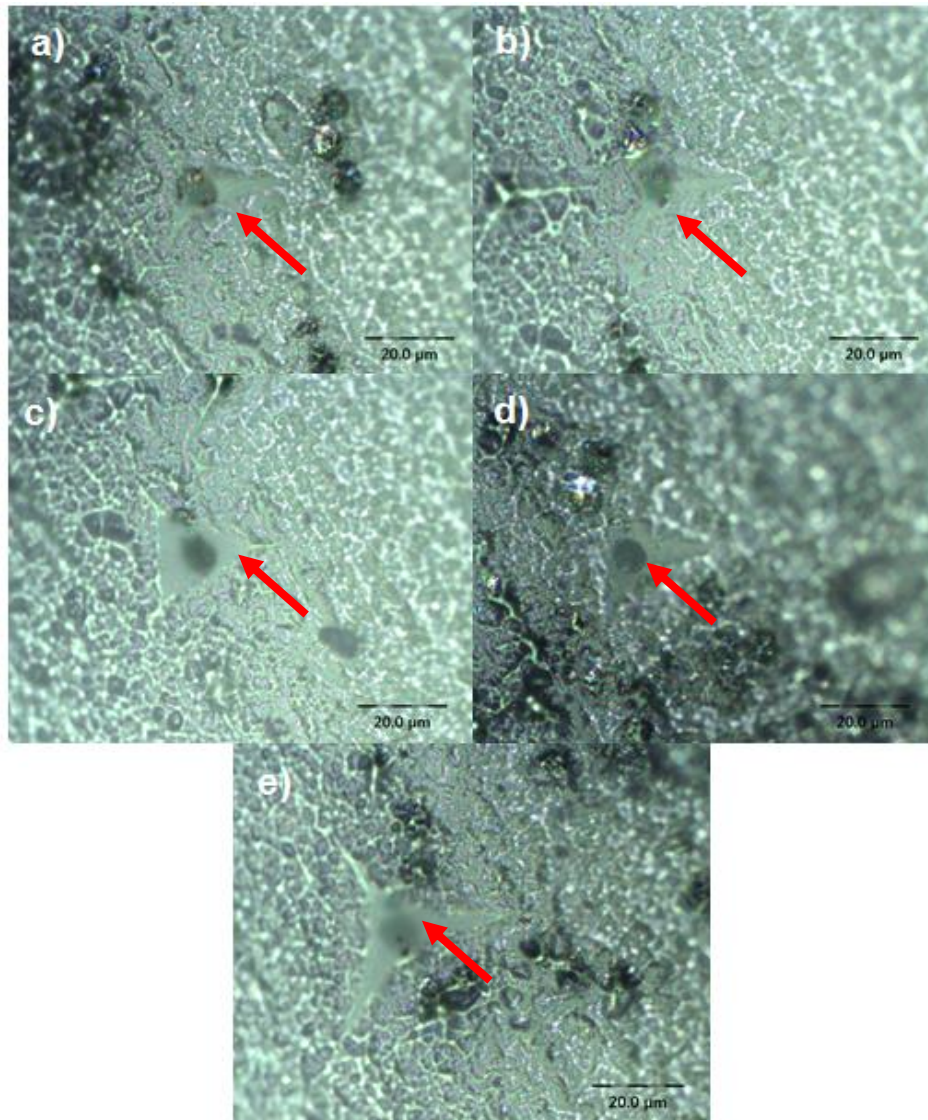
Figura 4.12 – Microscopia das amostras puras após indentação, aplicando uma carga máxima de: a-d) 100 mN e e) 250 mN.
