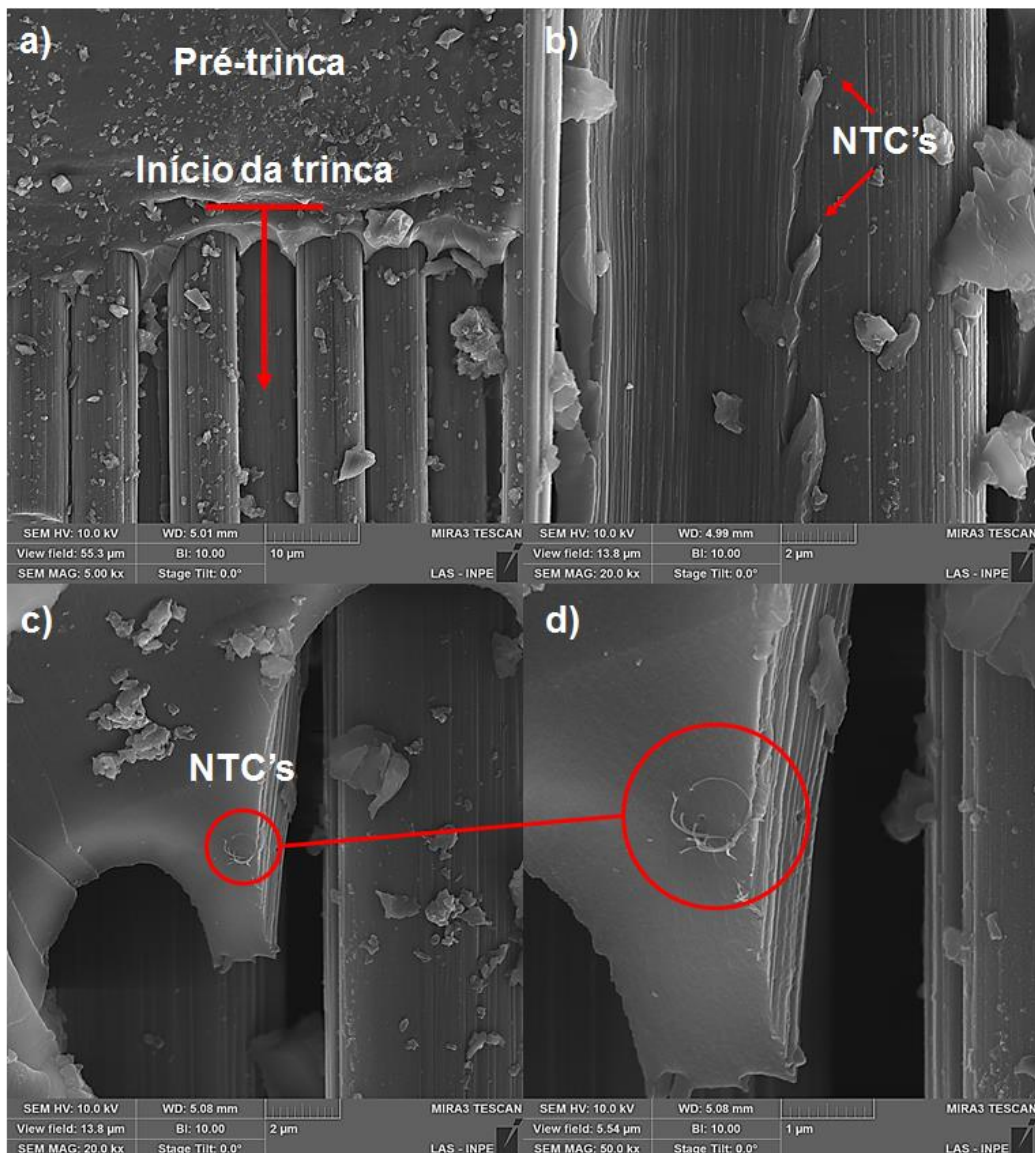
Figura 4.34 – Micrografias MEV-FEG do início da trinca após o ensaio de tenacidade à fratura em amostras com NTC's.
