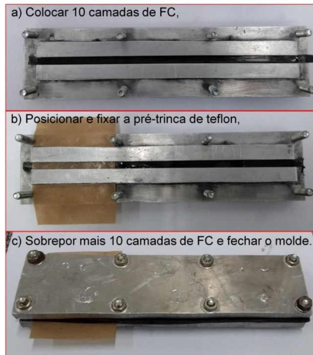
Figura 3.13 – Etapas da manufatura dos compósitos para ensaio.
