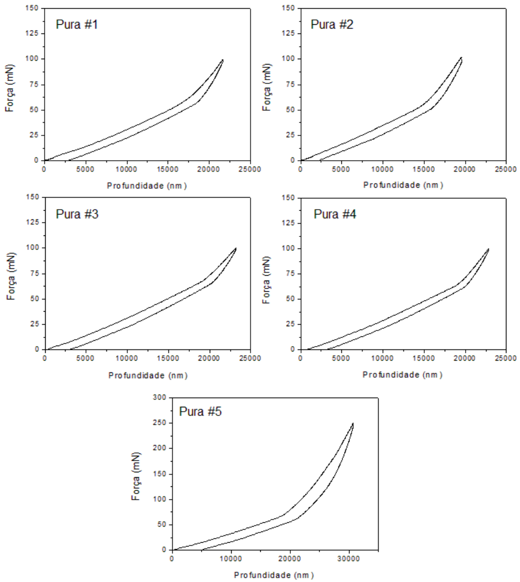
Figura 4.11 – Curvas de Força em função da Profundidade das fibras puras.
