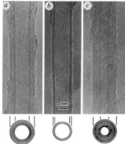
Figura 2.12 – Micrografias eletrônicas de transmissão dos nanotubos observados por Iijima e ilustração da seção transversal: a) Nanotubo com 5 folhas e diâmetro externo de 6.7 nm, b) nanotubo com 2 folhas e diâmetro de 5.5 nm e c) nanotubo com 7 folhas e 6.5 nm de diâmetro externo.
