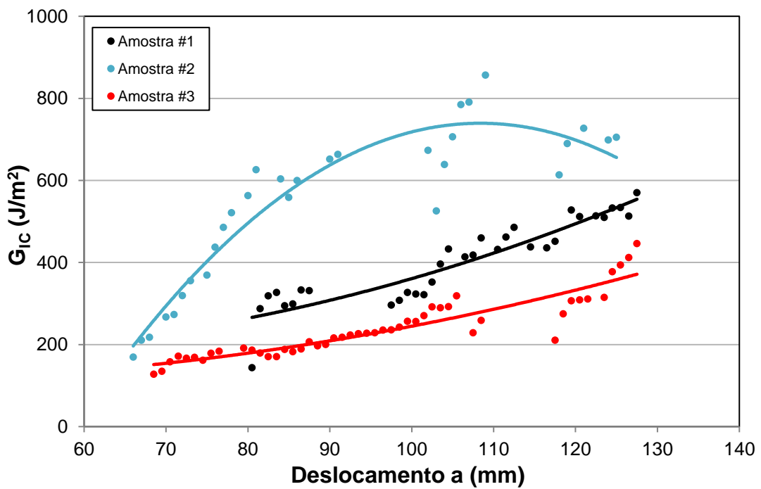
Figura C.4 - Curvas R a partir dos ensaios de Tenacidade à Fratura no Modo I, para amostras sem sizing com resizing.
