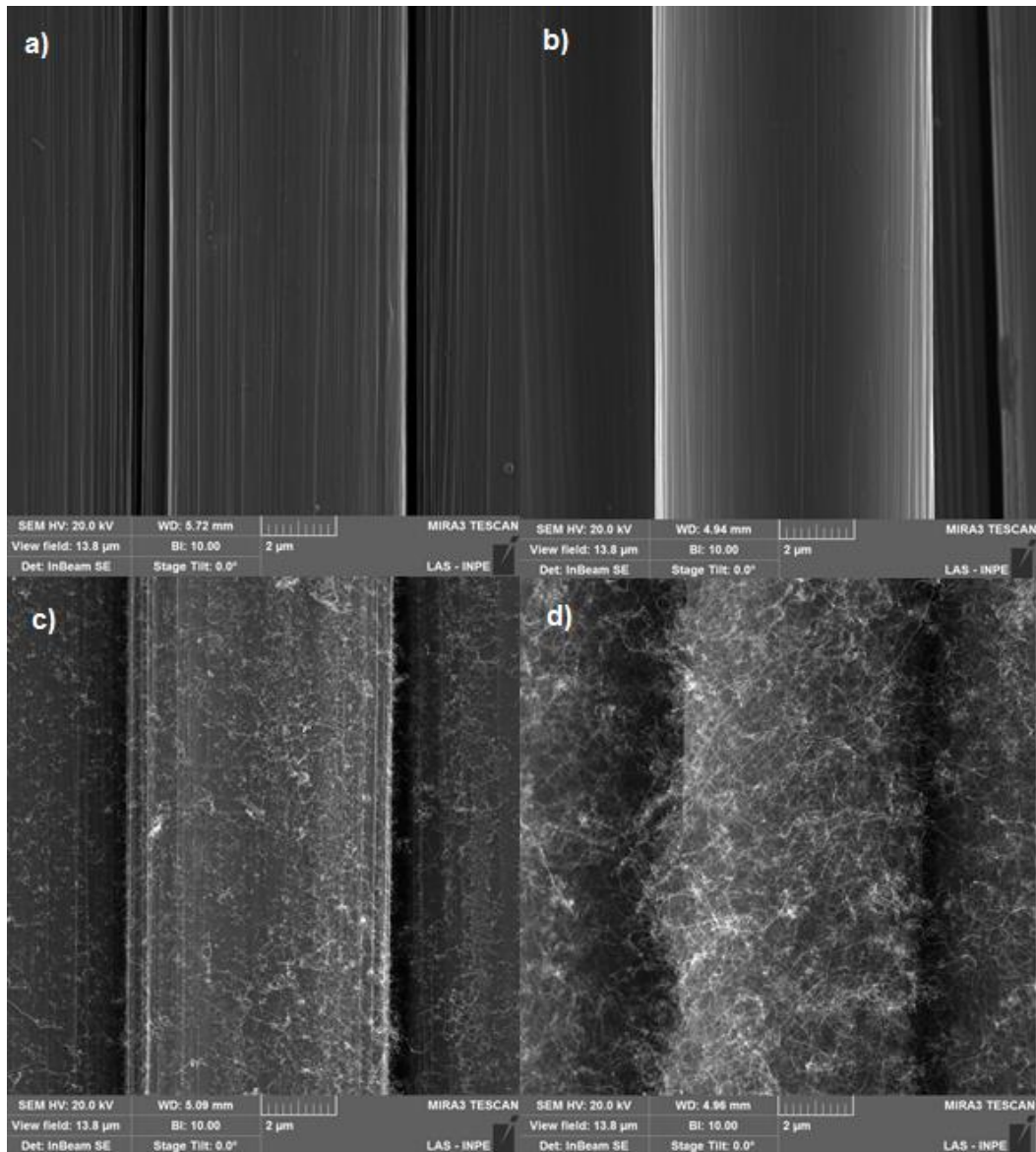
Figura 4.7 – Micrografias MEV-FEG da FC: a) pura, b) após tratamento com HMDSO e oxidação, c) com deposição de NTC's por 2 minutos e d) com deposição de NTC's por 5 minutos.
