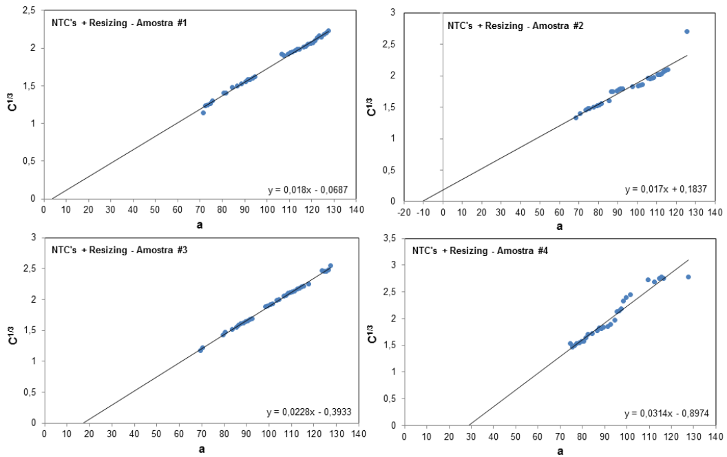
Figura B.3 – Curvas de Correção do Método MBT para amostras com NTC's e resizing
