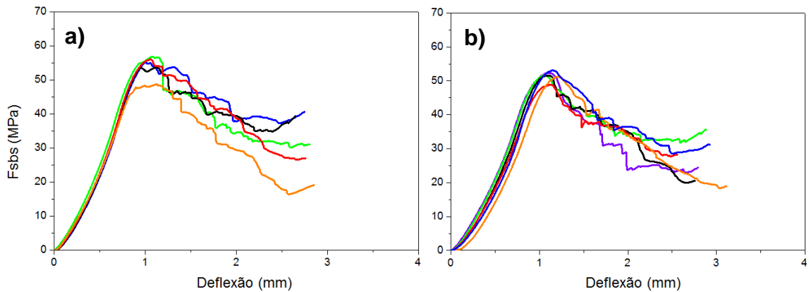
Figura 4.15 – Gráficos de Tensão de Cisalhamento em função da deflexão para amostras: a) puras e b) com tratamento superficial de HMDSO e oxidação.
