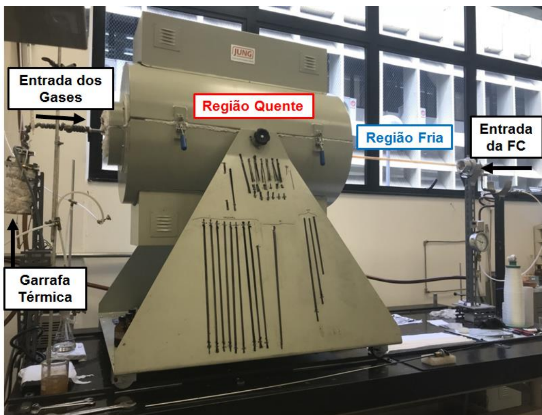
Figura 3.4 – Forno tubular utilizado para crescimento de NTC's.
