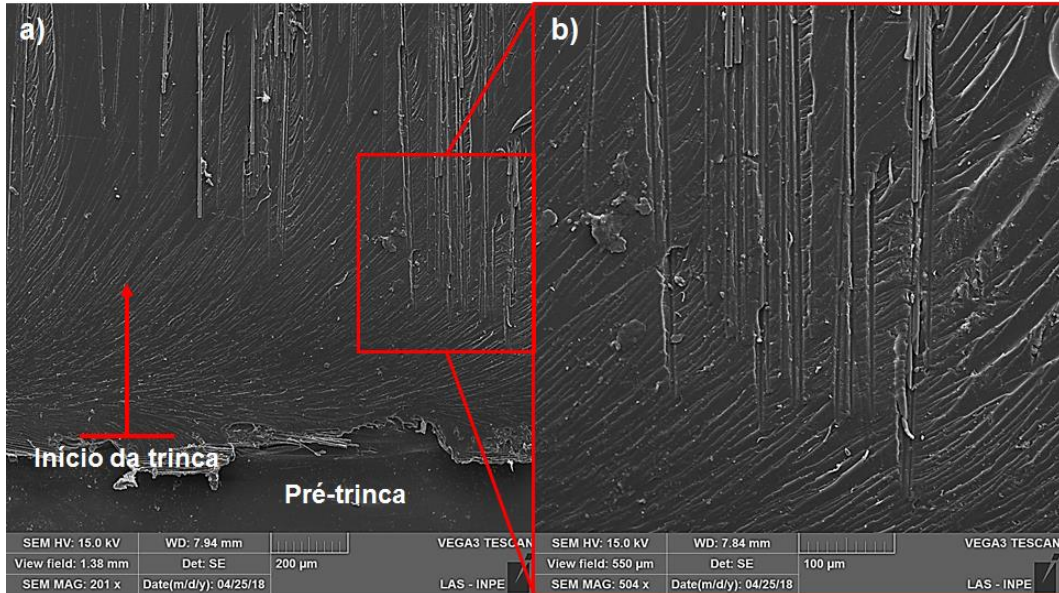
Figura 4.35 – Micrografias MEV-FEG do início da trinca após o ensaio de tenacidade à fratura em amostras com NTC's e resizing.
