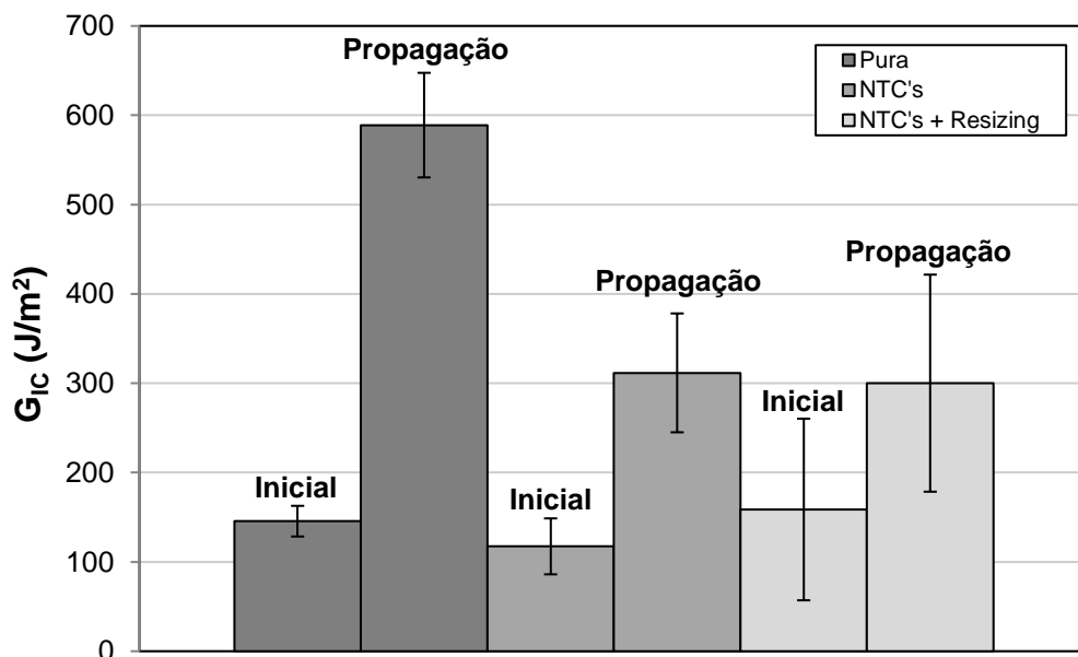
Figura 4.30 – Taxa de Liberação de Energia Inicial e Total a partir dos ensaios de Tenacidade à Fratura no Modo I, para amostras puras, com NTC's e NTC's com resizing.
