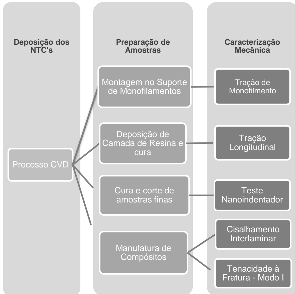
Figura 3.3 – Fluxograma das etapas após a deposição dos NTC's na FC.
