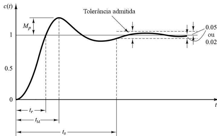
Figura 4.7 - Parâmetros de desempenho de uma resposta ao degrau
