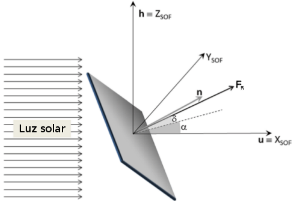
Figura 3.1 - Esquema da orientação da vela no Referencial Orbital da Espaçonave (SOF)
