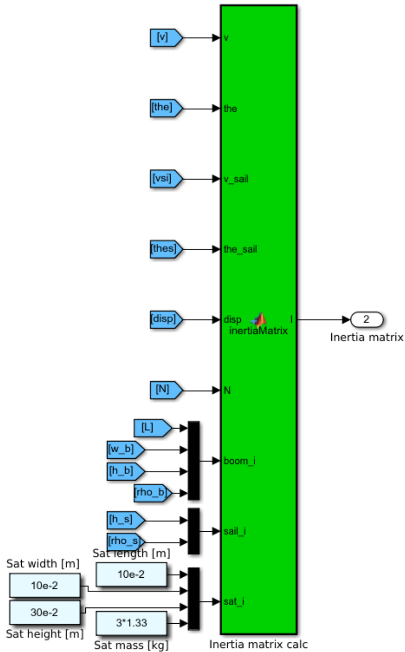
Figura 4.17 - Bloco da atualização do tensor de inércia da espaçonave
