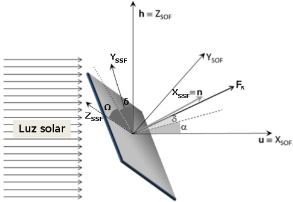
Figura 4.11 - Esquema de orientação da vela no SOF e no SSF
