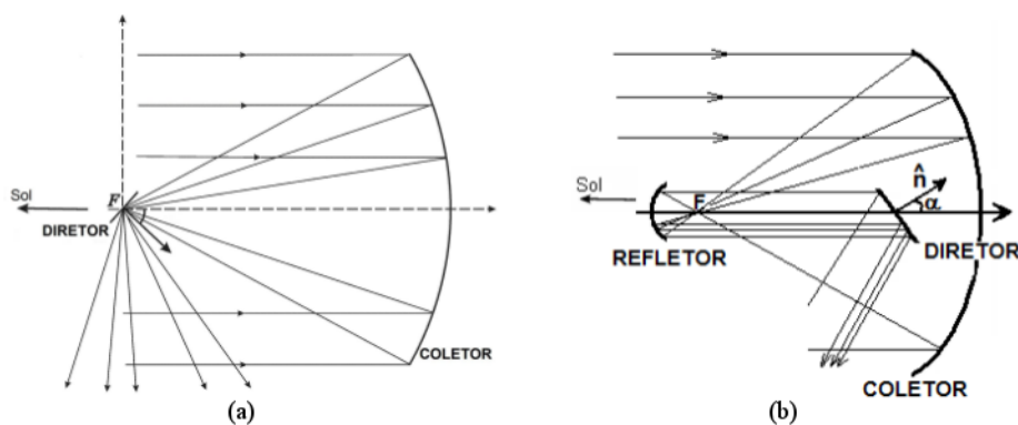
Configurações: (a) Simples (SSPT - Simple Solar Photon Thruster ), (b) de Dupla Reflexão (DR SPT - Double Reflection Solar Photon Thruster )
