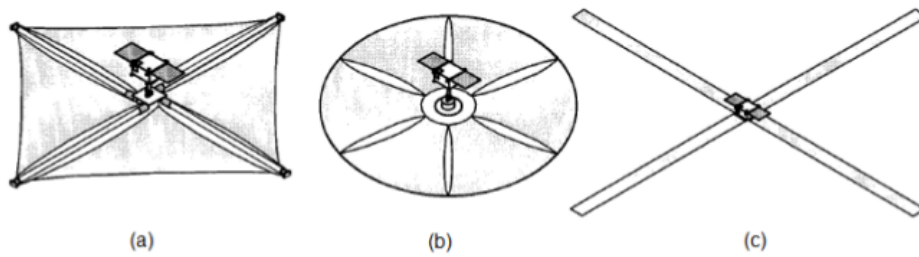
Configurações: (a) Vela quadrada, (b) Vela circular, (c) Heliogyro Fonte: Wie (2004a) .
