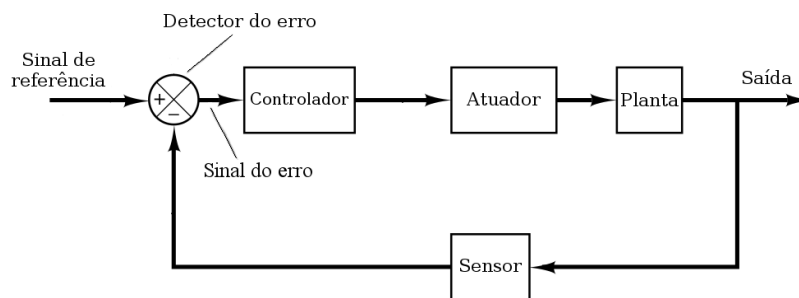
Figura 3.7 - Diagrama de blocos de um sistema de controle
