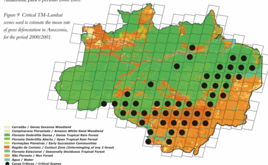
Figura 9 Cenas TM-Landsat críticas consideradas na geração da estimativa da taxa média do desflorestamento bruto na Amazônia, para o período 2000/2001.
