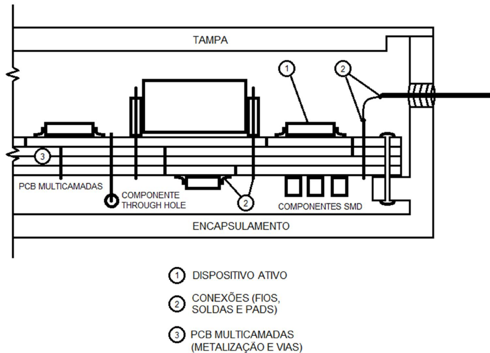
Figura 2.3 – Pontos de susceptibilidade a falhas em conversores compactos.
