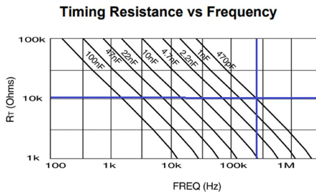
Figura 4.6 – Determinação da frequência de operação do PWM.
