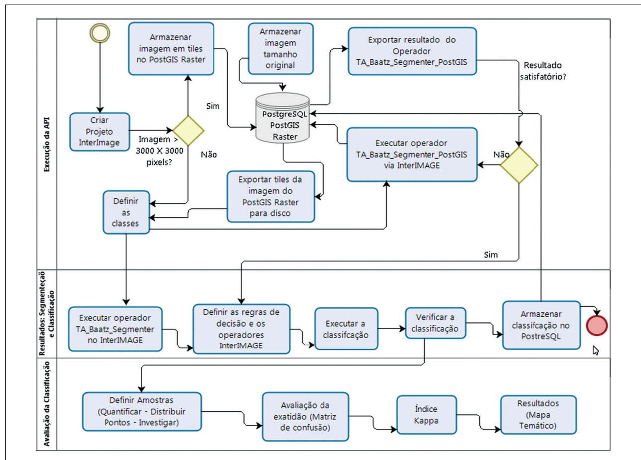
Figura 2 Fluxograma de construção da API TA_Baatz_Segmenter_PostGIS no PostgreSQL/PostGIS Raster e classificação no InterIMAGE.
