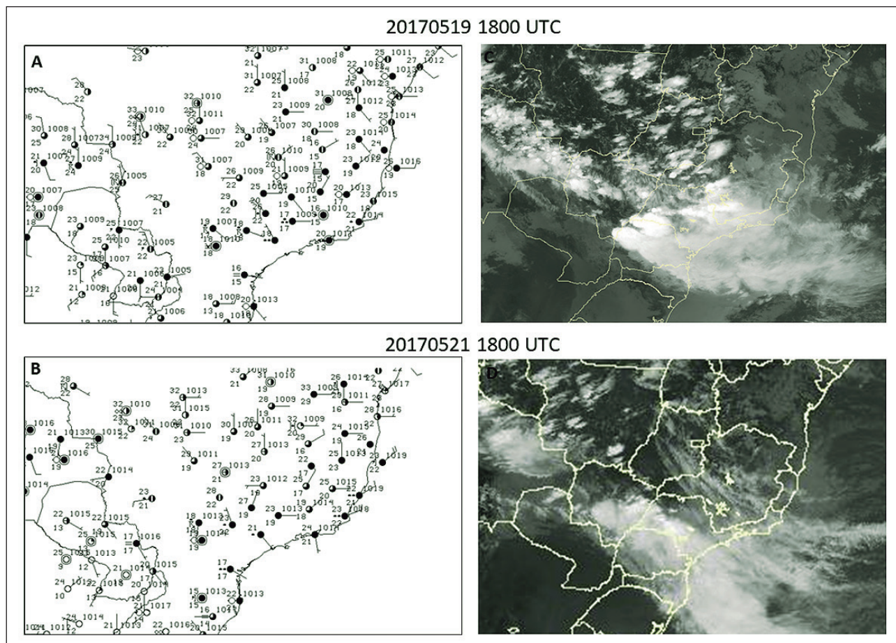
Figura 8 A-B: Synop ( http://img0.cptec.inpe.br/~rp/proc/cartas/ ) e C-D imagens do canal infravermelho (10,7 μm) do satélite GOES-13 ( http://satellite.cptec.inpe.br/acervo/goes.formulario.logic ) dos dias 19 (A-C) e 21 (B-D) de maio de 2017 às 1800 UTC.
