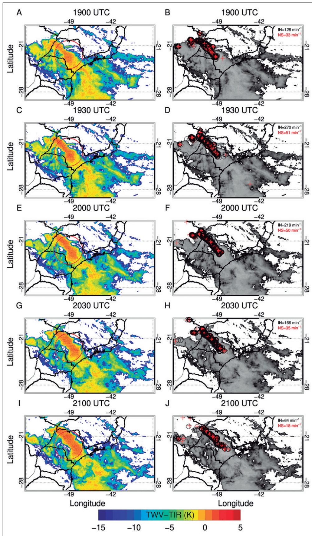
Figura 9 (A.; C.; E.; G. e I.) diferença de temperatura de brilho (K) entre o canal do vapor d'água (TW, 6,5 \mu\text{m} ) e a temperatura de brilho no canal do infravermelho (TIR, 10,7 \mu\text{m} ) (TWV-TIR, região colorida) no dia 21 de maio de 2017 entre 1900 e 2100 UTC e (B.; D.; F.; H. e J) frequência de ocorrência de relâmpagos (número de relâmpagos acumulados em 30 min) intra-nuvem (círculo aberto na cor preta) e nuvem-solo (cruz na cor vermelha). Os círculos vermelhos nos painéis a esquerda indicam o raio de 240 km de atuação do radar de Bauru.
