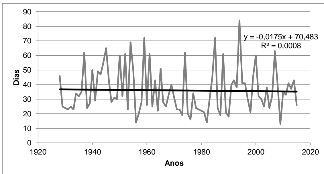
Figura 12 – Dias consecutivos sem precipitação (CDD) calculados para a série de precipitação anual média em Jacareí – SP (área urbana e rural) no período de 1928 até 2015
