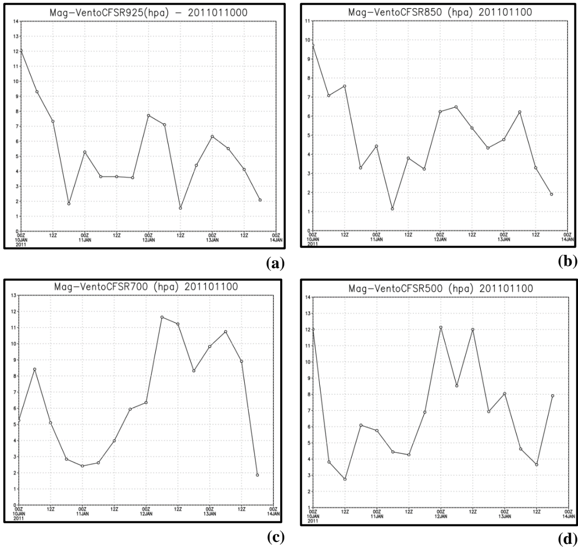
Figura 03 - Evolução temporal da magnitude do vento no ponto de latitude XX e longitude XX. Dados da reanálise CFSR. (a) nível de 925 hPa; (b) nível de 850 hPa; (c) nível de 700 hPa e (d) nível de 500 hPa
