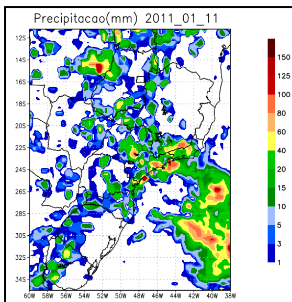
Figura 4 – Precipitação observada acumulada em 24 horas, válida para 11/01/2011.às 12Z.
