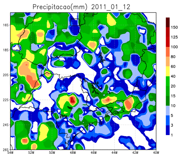
Figura 4 – Precipitação observada acumulada em 24 horas, válida para 12/01/2011.às 12Z
