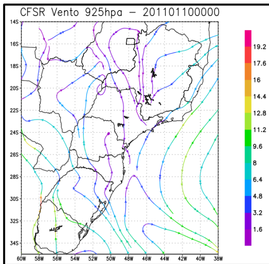
Figura 01 – Intensidade do vento a 925, 10 de janeiro 2011 as 00 Horas.
