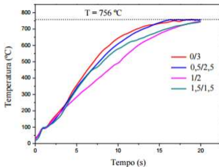
Figura 8 – Curvas de temperatura dos catalisadores obtidas nos testes no micro reator de leito fixo
