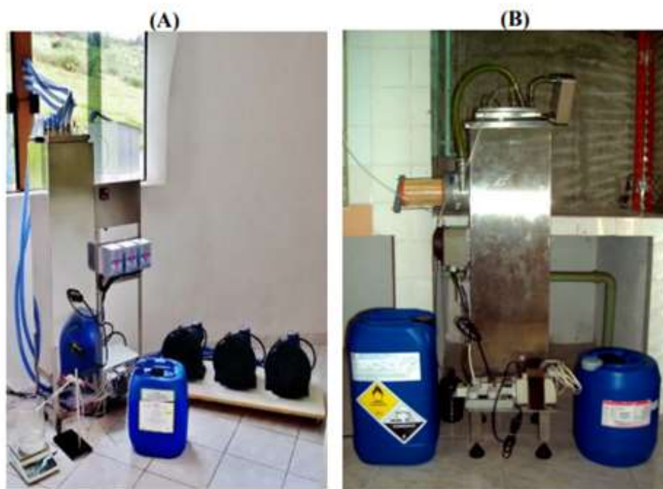
Figura 1 – (A) Novo concentrador de \text{H}_2\text{O}_2 , (B) Antigo concentrador do LCP/INPE
