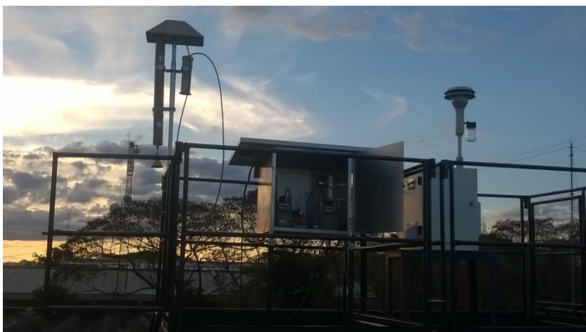
Figura 2 Amostrador dicotomico de São José dos Campos
