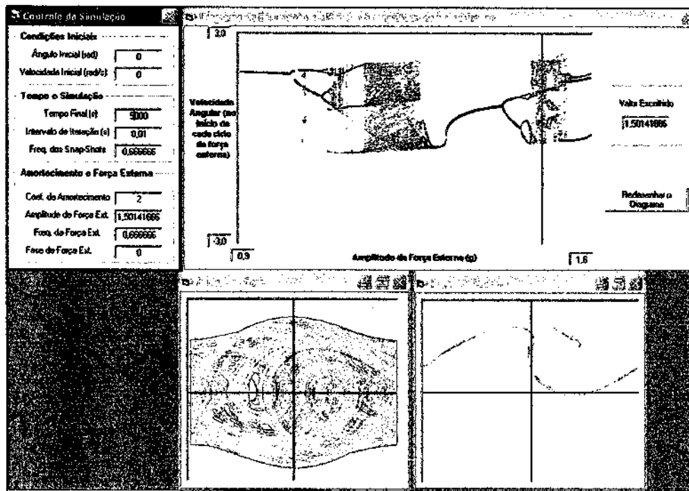
Figura 9: Situação de comportamento caótico
