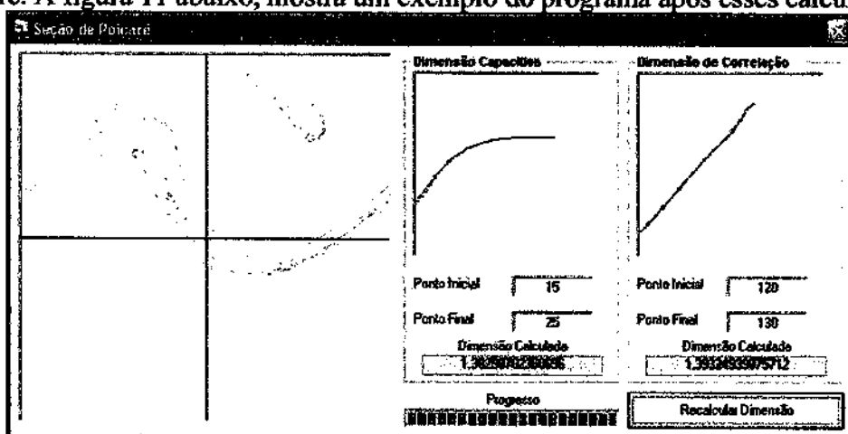
Figura 11: Dimensões para o atrator com g = 1,4954 , q = 4 , \omega_D = 2/3
