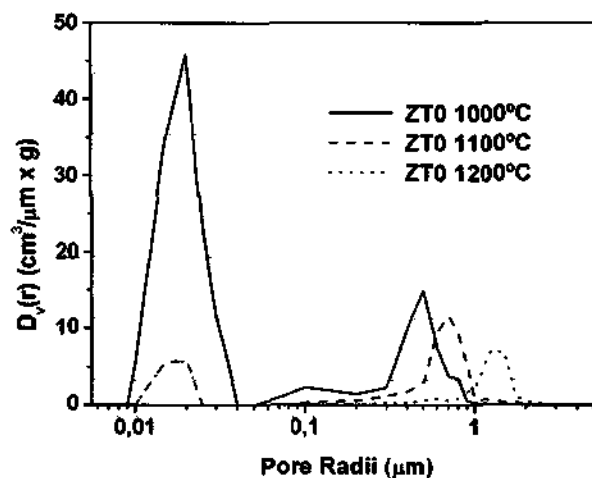
FIGURA 19. Distribuição de volume de poros em função dos raios dos poros para cerâmicas de ZrO_2-TiO_2 sinterizadas nas temperaturas de 1000, 1100 e 1200°C.
