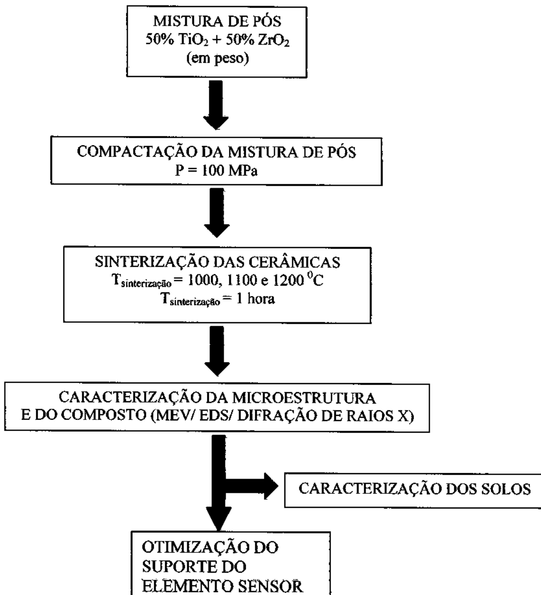
FIGURA 1. Fluxograma do processo de fabricação e caracterização das cerâmicas porosas.
