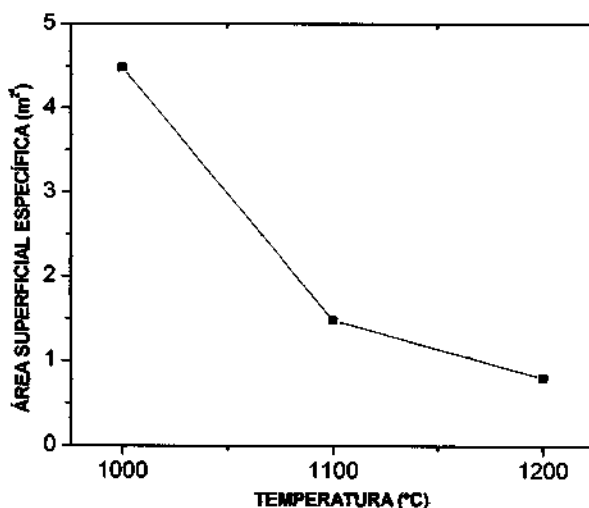
FIGURA 18. Área superficial específica das cerâmicas sinterizadas em 1000, 1100 e 1200 °C por 1 hora.
