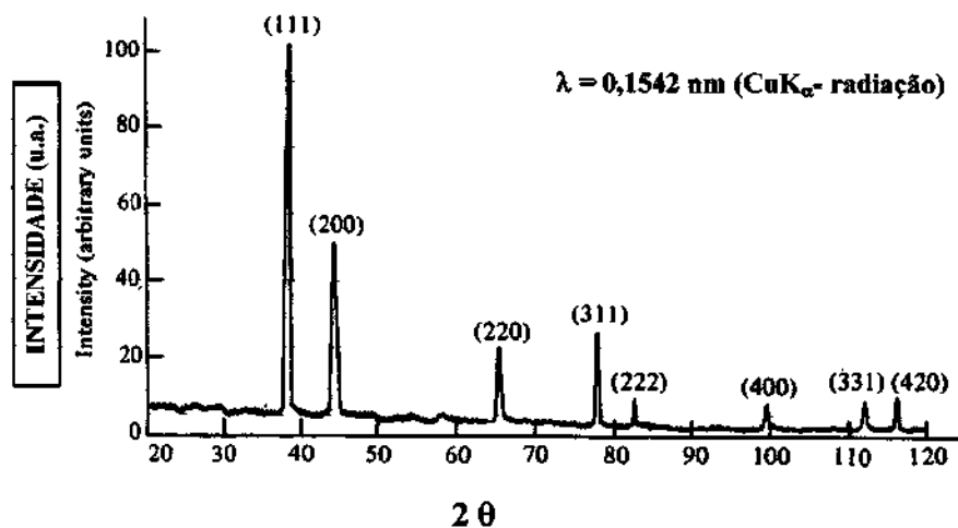
Figura 12. Difratoograma de difração de raios X do alumínio puro [14]
