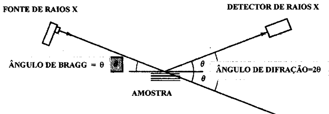
Figura 11. Relação entre o ângulo de Bragg ( \theta ) e a medida experimental do ângulo de difração de raios X [15]
