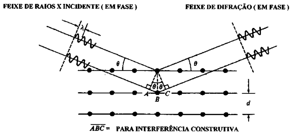
Figura 10. Geometria da difração de raios X [14]
