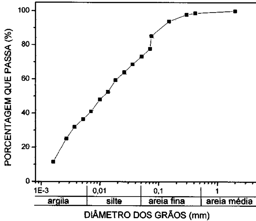
FIGURA 20. Gráfico granulométrico do solo "C", apresentando 25% de argila, 36% de silte, 26% de areia fina e 2% de areia média.
