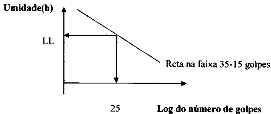
FIGURA 13. Gráfico representativo para a obtenção do limite de liquidez
