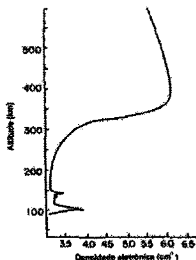
Fig. 2.5 – Perfil de densidade eletrônica típico da região equatorial no período após o pôr-do-sol.
