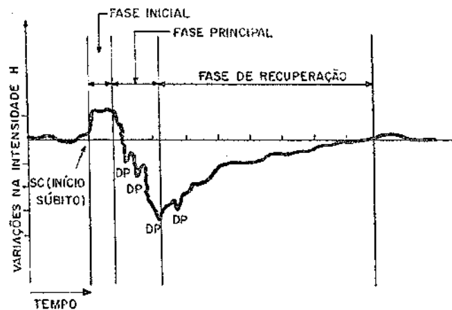
Fig. 3.3 – Fases características de uma tempestade magnética.
