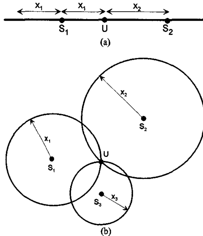
Fig. 4.3 – Posicionamento (a) unidimensional e (b) bidimensional de um usuário U .
