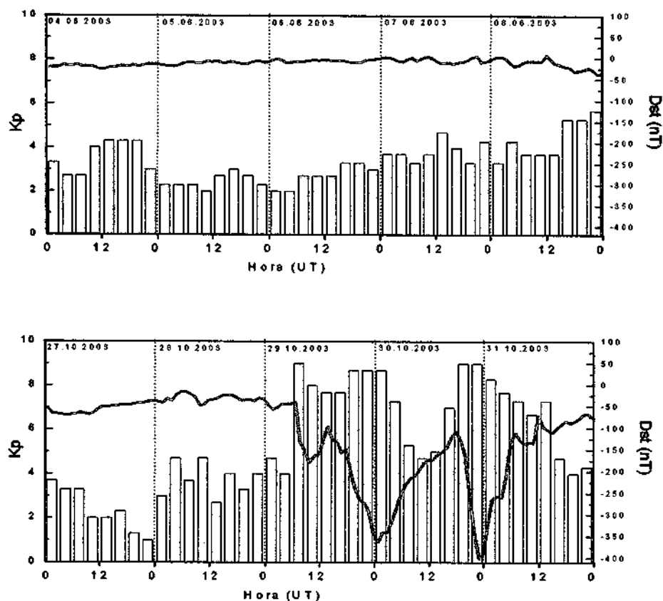
Fig. 7.3 – Variação dos índices Kp e Dst entre os dias 04 e 08 de junho, 27 e 31 de outubro de 2003.
