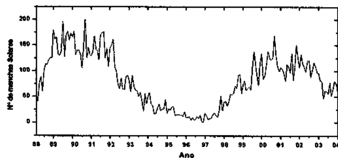
Fig. 7.2 – Variação do fluxo solar em 10.7 cm, entre Janeiro/1988 e Dezembro/2003.
