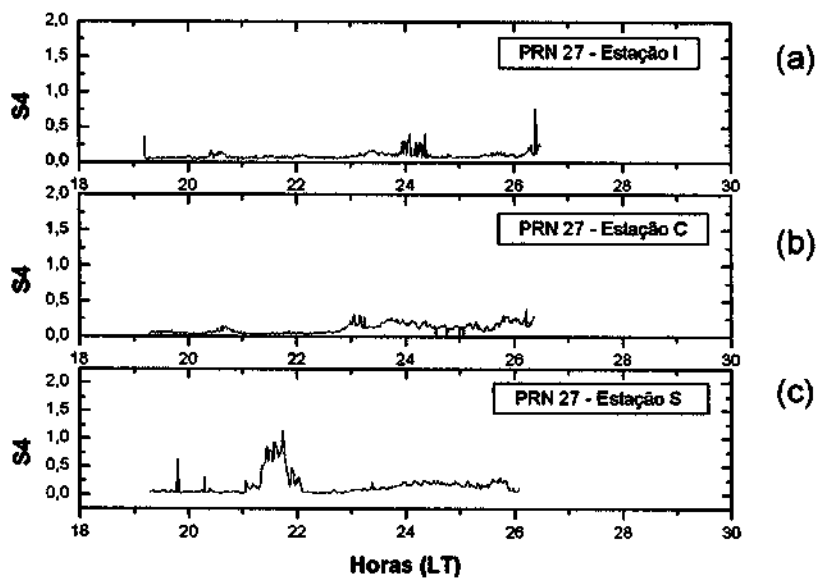
Fig. 7.5 – Variação do índice S4 do satélite PRN 27 para as estações GPS de (a) - São Luís, MA, (b) - São José Campos e (c) - São Martinho da Serra respectivamente para o dia 29.10.03 com incidência de tempestade magnética.
