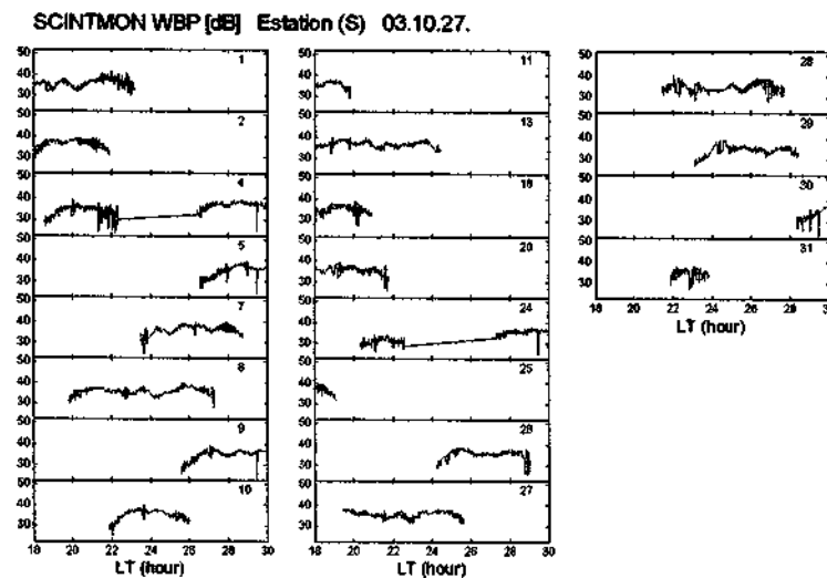
Fig. 6.2 - Os diversos painéis mostram os valores de potência em banda larga de sinal recebido, WBP em decibéis, para os satélites rastreados na noite de 27/10/2003 para 28/10/2003. O PRN, identificação, de cada satélite é indicado no canto superior direito de cada painel, observados no Observatório Espacial do Sul, RS.
