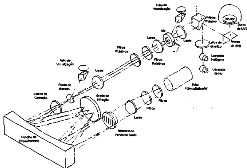
Fig. 4.13 - Vista esquemática dos componentes do sistema ótico do Brewer.
