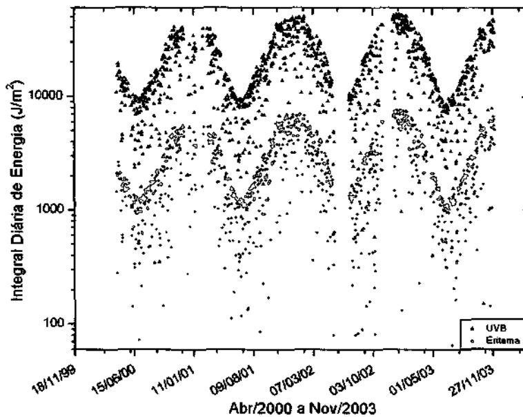
Fig. 6.2 – Dados brutos de Integral Diária de Energia de Radiação UVB e Eritematosas incidentes no OES/CRSPE/INPE, plotados em escala logarítmica para todo o período analisado.
