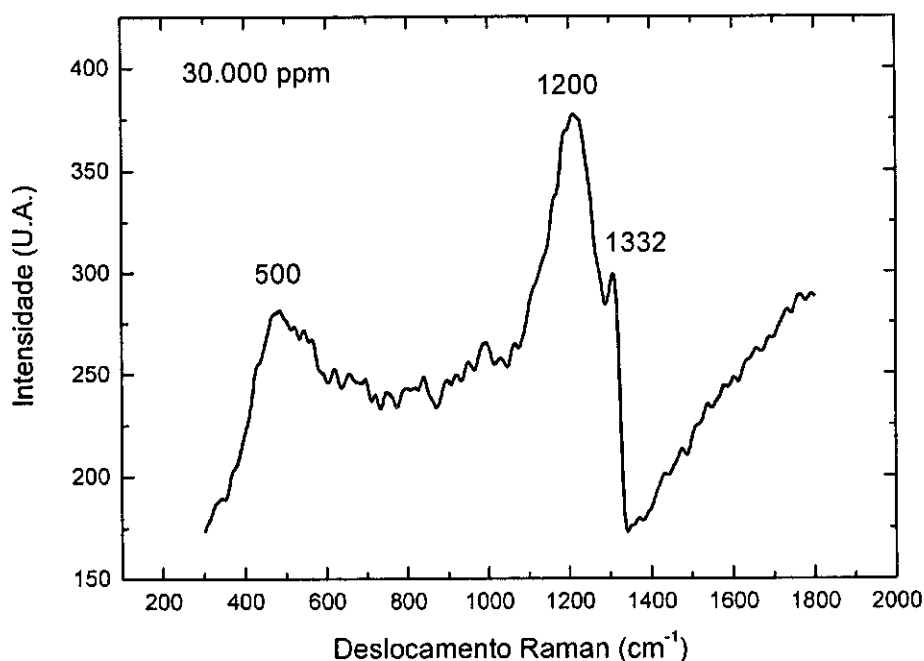
Figura 4: Espectro Raman do filme DDB obtido.
