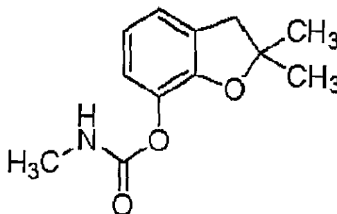
Figura 1: Estrutura do Carbofurano
