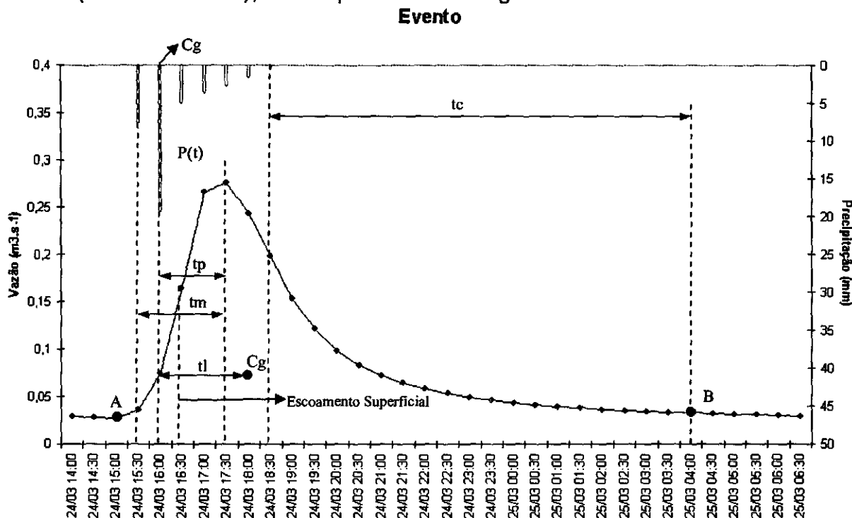
Figura 5 - Precipitação - Vazão
