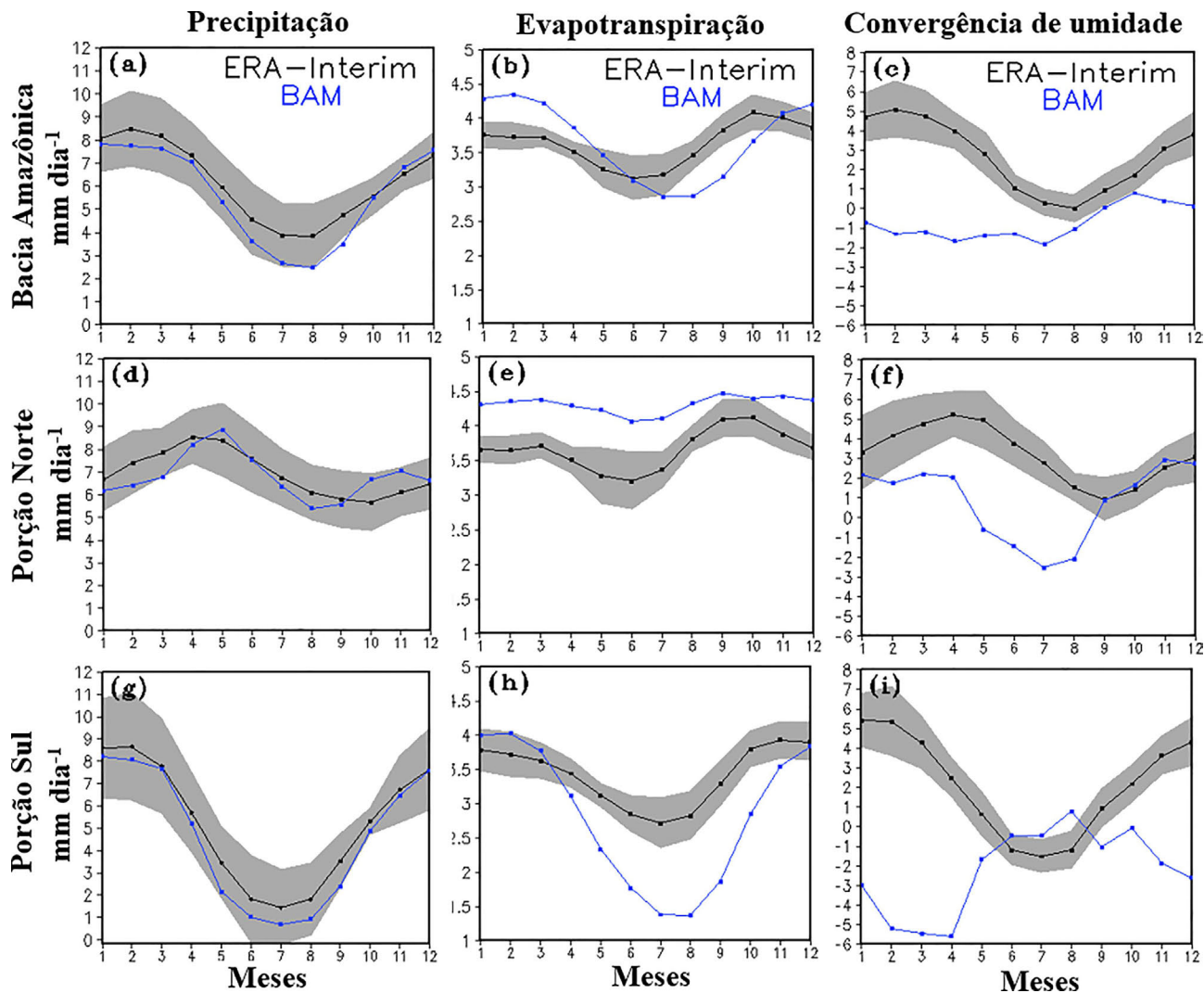
Figure 7 - Ciclo anual dos componentes do balanço de água (Precipitação, Evapotranspiração e Convergência de umidade) em (mm.dia -1 ), simulado pelo BAM (linha azul) e da reanálise do Era-Interim (linha preta). A área em cinza representa o desvio padrão da reanálise: (a,b,c) para toda a Bacia Amazônica; (d,e,f) para Porção Norte da bacia e (g,h,i) para Porção Sul da bacia.
