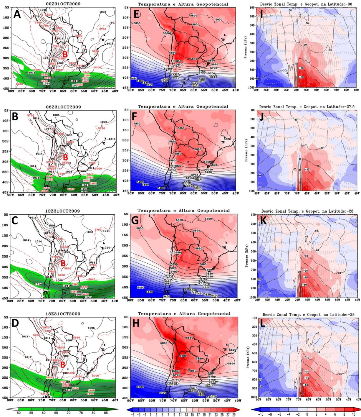
Figura 6. A-D) Pressão ao nível médio do mar (hPa; linhas pretas), espessura da camada 500/1000 hPa (metros, linhas vermelhas tracejadas) e intensidade do vento em 250 hPa (m/s, ventos com intensidade superior a 50 m/s em colorido). E-H) Altura geopotencial em 500 hPa (mgp, linhas pretas) e temperatura do ar em 850 hPa (°C, colorido). I-L) Perfil vertical do desvio zonal de temperatura (°C, colorido), altura geopotencial (mgp, linhas pretas) e velocidade vertical (Pa/s) composta com a componente zonal do vento (m/s; vetores em cor cinza) para os quatro horários sinóticos do dia 31/10/2009. A BNOA é indicada com a letra B.
