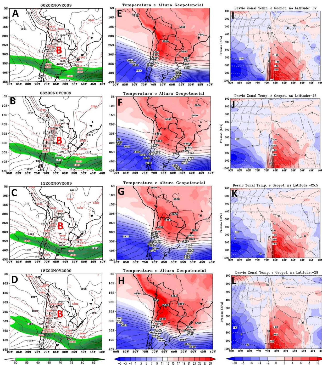
Figura 8. A-D) Pressão ao nível médio do mar (hPa; linhas pretas), espessura da camada 500/1000 hPa (metros, linhas vermelhas tracejadas) e intensidade do vento em 250 hPa (m/s, ventos com intensidade superior a 50 m/s em colorido). E-H) Altura geopotencial em 500 hPa (m, linhas pretas) e temperatura do ar em 850 hPa (°C, colorido). I-L) Perfil vertical do desvio zonal de temperatura (°C, colorido), altura geopotencial (m, linhas pretas) e velocidade vertical (Pa/s) composta com a componente zonal do vento (m/s; vetores em cor cinza) para os quatro horários sinóticos do dia 02/11/2009. A BNOA é indicada com a letra B.
