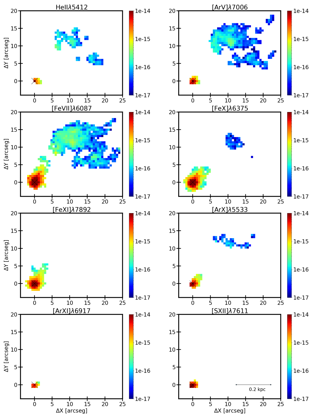
Mapas de fluxos para linhas de He II \lambda 5412 , [Ar V] \lambda 7006 , [Fe VII] \lambda 6087 , [Fe X] \lambda 6375 , [Fe XI] \lambda 7892 , [Ar X] \lambda 5533 , [Ar XI] \lambda 6917 e [S XII] \lambda 7611 .
